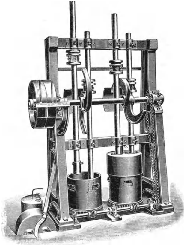
Abb. 10. Pulverisiermaschine.
