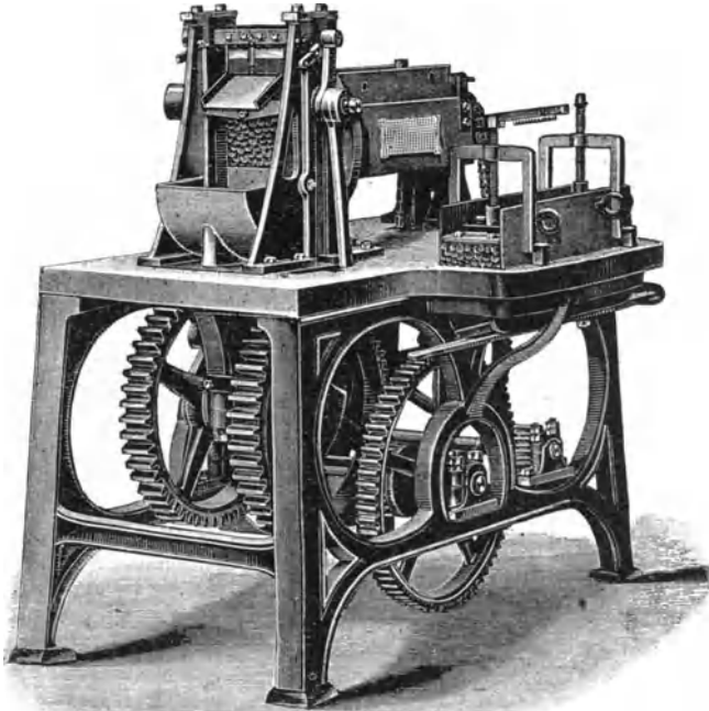
Abb. 7. Würfelschneidemaschine.
