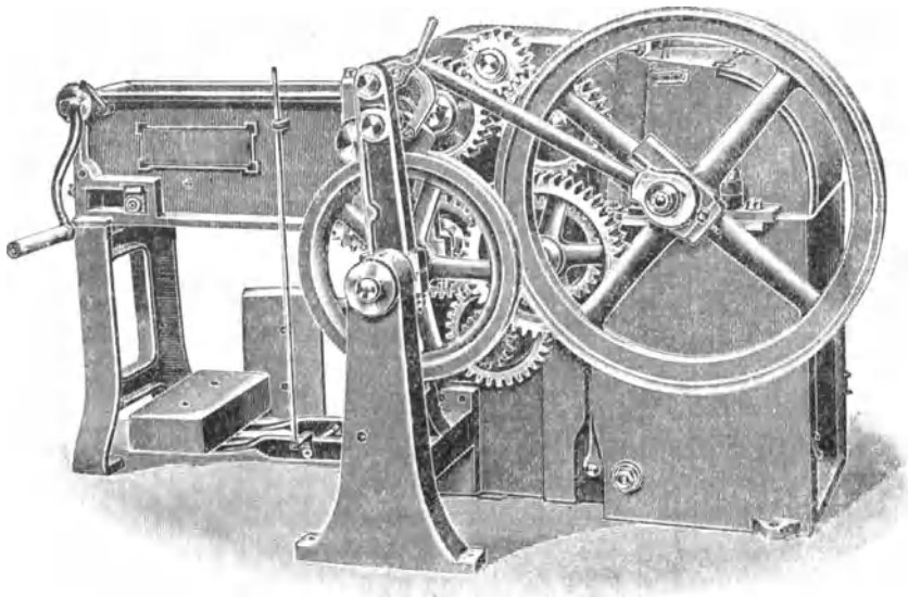
Abb. 6. Quadratschneidemaschine mit erhöhter Leistungsfähigkeit.
