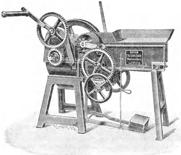
Abb. 5. Quadratschneidemaschine.
