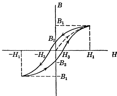
FIG. 21.—Hysteresis loop.
