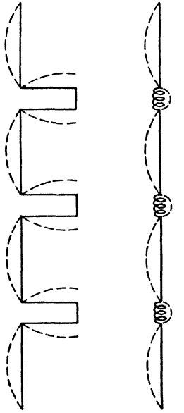
Marconi-Franklin antennas
