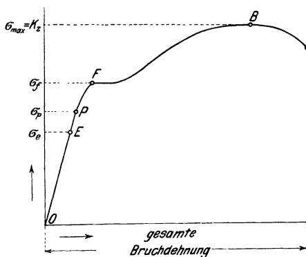
Abb. 91. Dehnungskurve eines Metallstabes (nach WAWRZINIÖK). Auf der Abszisse sind die Dehnungsgrößen, auf der Ordinate die zugehörigen Spannungsgrößen aufgetragen.
