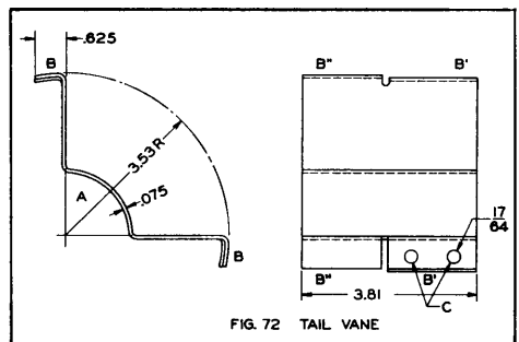
FIG. 72 TAIL VANE
