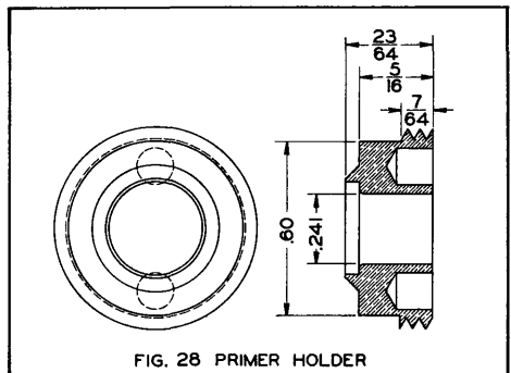
FIG. 28 PRIMER HOLDER
