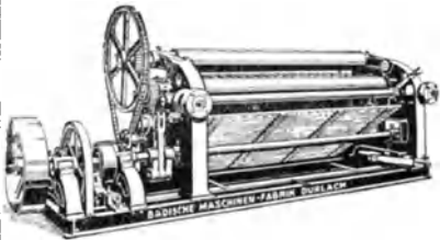
Neueste rotierende Ausreck- und Abwelkmaschine „Rekord“ mit Faltenverteilungswalze
