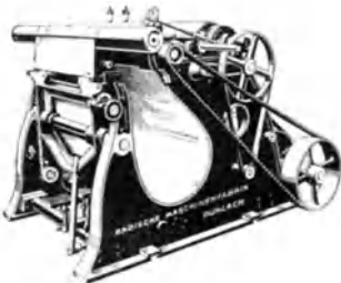
Neueste Falzmaschine „Luna“ mit doppeltbreitem Falzzyylinder
