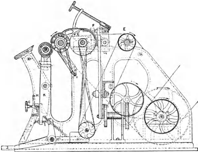
Abb. 37. Schnitt durch eine Falzmaschine.
