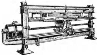
Chagrinier-, Satinier- und Bügelmachine „Gloria“ mit feststehendem Tisch und feststehender Preßplatte
