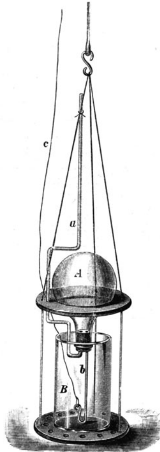
Fig. 28. Apparat zur Probeentnahme aus Bohrlöchern nach Lepsius.
