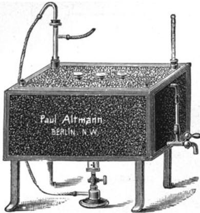
Fig. 12. Einfacher Thermostat.
