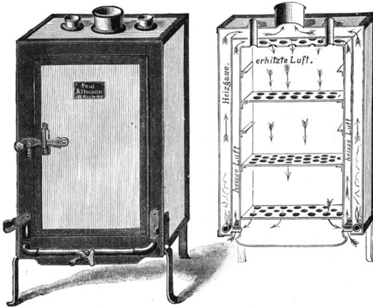
Fig. 11. Heissluftsterilisator mit überall konstanter Innentemperatur.
