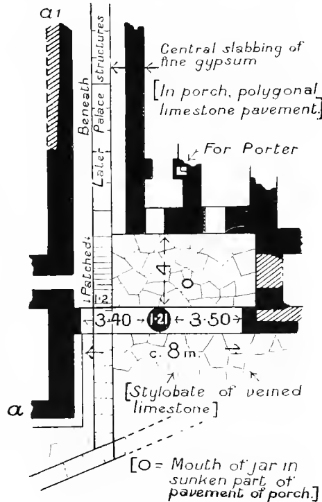
FIG. 159. WEST PORCH, PHAESTOS.
