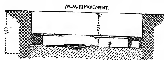
SECTION A-B
