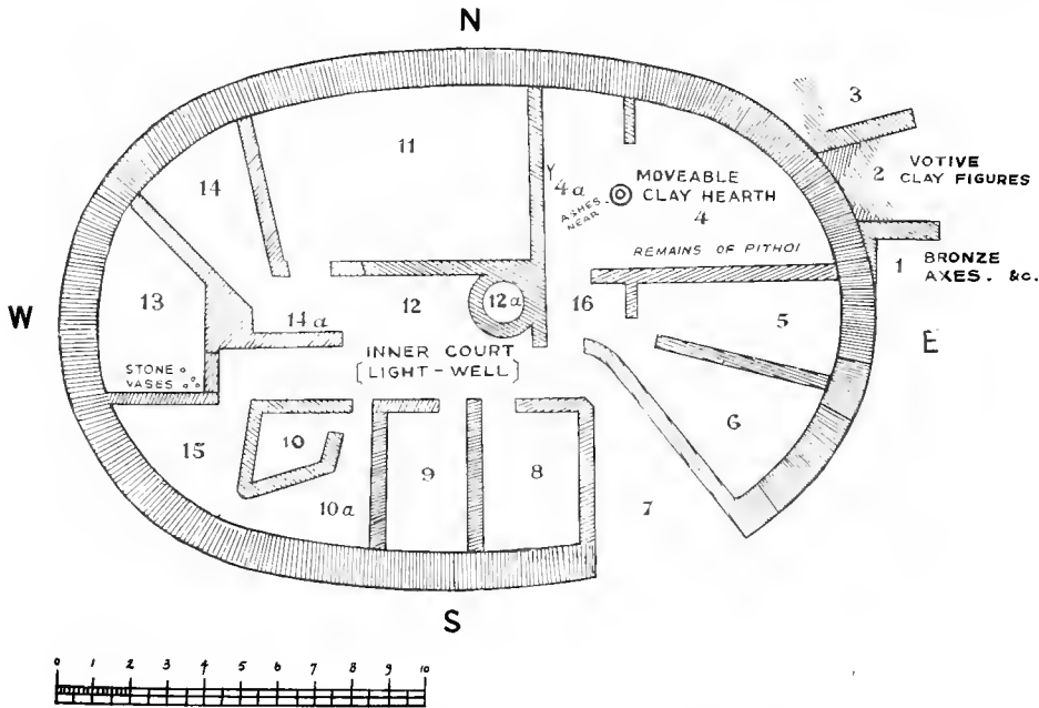
FIG. 108. OVAL HOUSE, CHAMAEZI (M. M. I).
