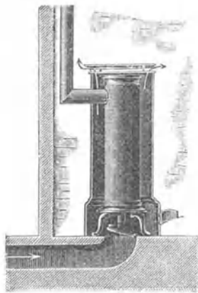
Abbildung 36. Mantelöfen.
