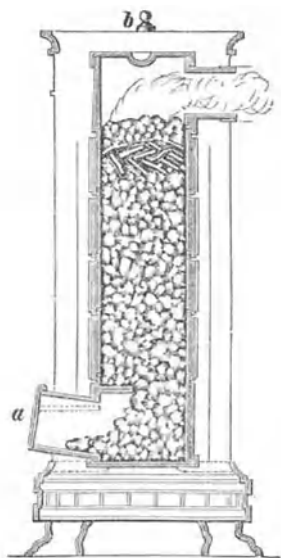
Abbildung 35. Füllöfen.
