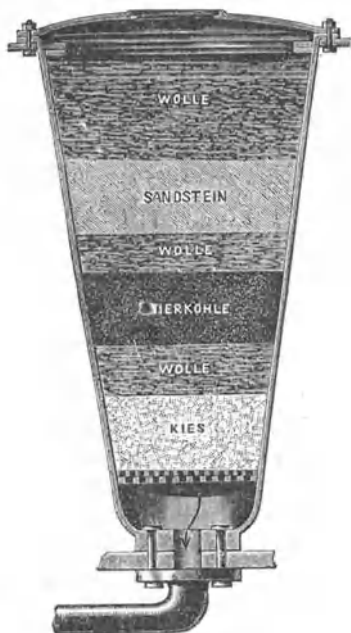
Abbildung 19. Zusammengefügtes Hausfilter.
