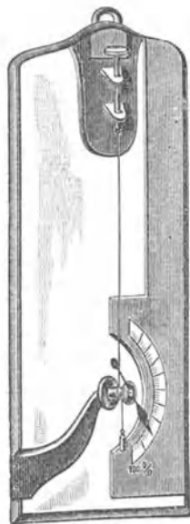
Abbildung 13. Hygrometer. *)
