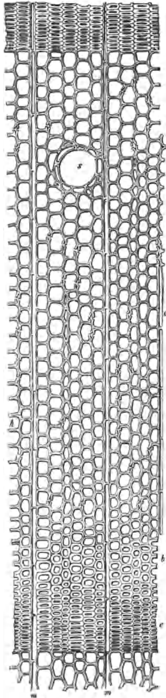
Fig. 52. Querschnitt durch das Holz einer Fichte, welche im Freien erwachsen ist. Die weitleumige dünnwandige Region a überwiegt im Vergleich zur dickwandigen Rundfaserschicht b und Breitfaserschicht c.
