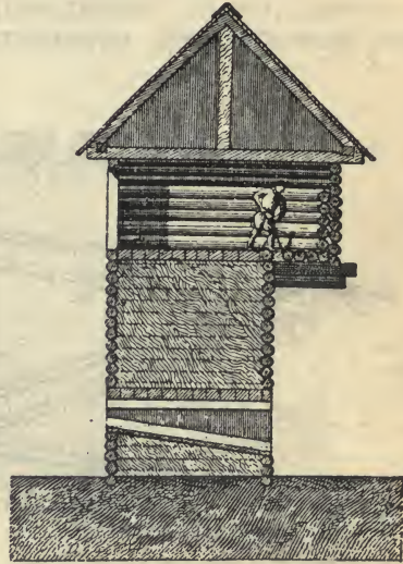
Разрѣзъ старинной деревянной глухой башни.
