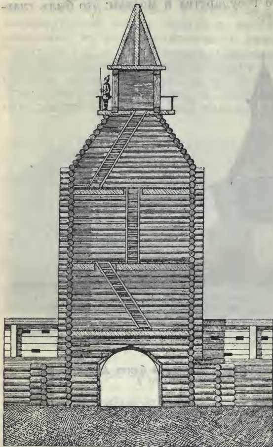
Разрѣзъ старинной деревянной проѣздной башни.
