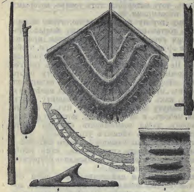
Детали норманской ладьи.
