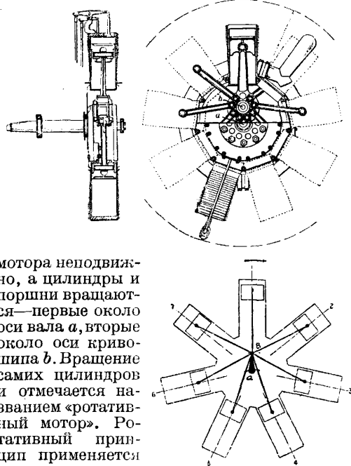
Фиг. 4. Схема ротативного мотора.
