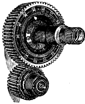
Фиг. 30. Пружинный редуктор двигателя Кертинс GV 1550 600 P.
