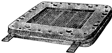
Фиг. 8. Двойная платиновая контактная сетка из конвертора.
