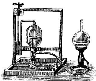
Фиг. 9. Сожигательная пипетка Кокильбона.
