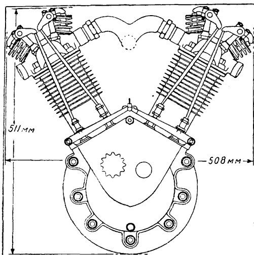
Фиг. 6. Двигатель Бленборн с V-образным расположением цилиндров.
