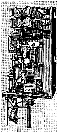
Фиг. 9. Искатель системы Autelco.
