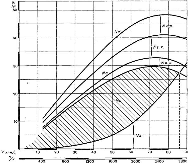
Фиг. 29. Баланс мощности автомобиля на прямой передаче.
