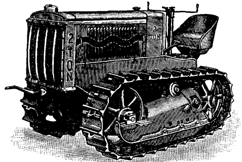
Фиг. 1. Новейшая 2\frac{1}{2} -т модель американского гусеничного трактора фирмы Холт.
