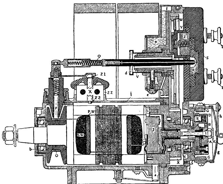
Фиг. 24. Магнето Бош.
