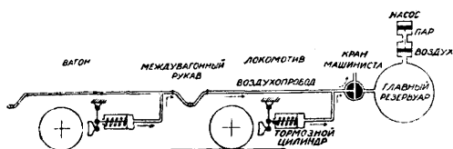
Фиг. 1. Неавтоматический тормоз.—Схема положения оттормаживания.
