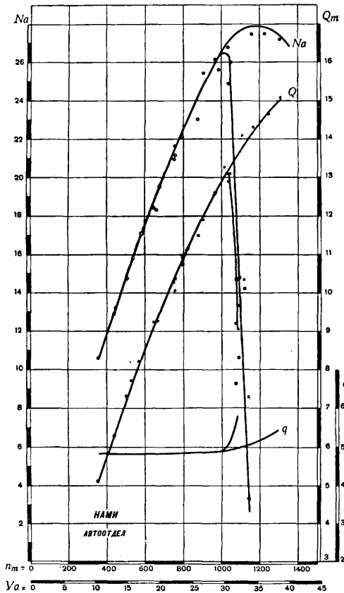
Фиг. 33. Диаграмма N_{а.} , Q и q на прямой передаче в зависимости от V_{а} и N_{м.}
