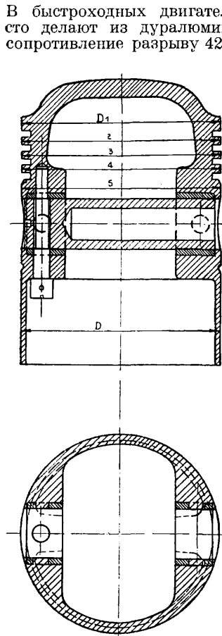
Фиг. 12. Легкие поршни.
