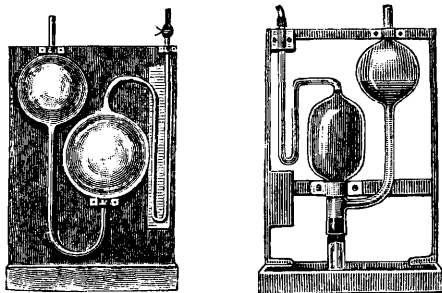
Фиг. 8. Газовые пипетки.
