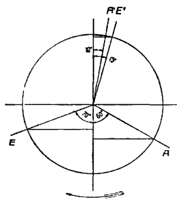
Фиг. 3. Диаграммы распределения мотора: A — начало выпуска, A' — конец выпуска, E' — начало всасывания, E — конец всасывания.
