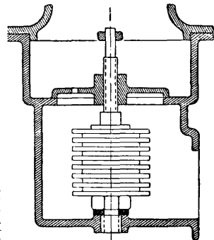
Фиг. 22. Термостат.
