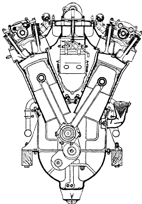
Фиг. 10. Поперечный разрез авиационного двигателя Либерти 400 HP.
