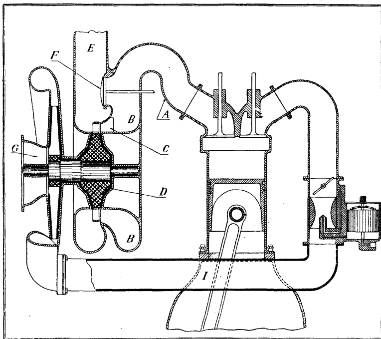
Фиг. 34. Схема установки турбокомпрессора.
