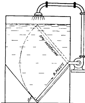
Фиг. 2. Агитация с помощью центробеж. насоса.
