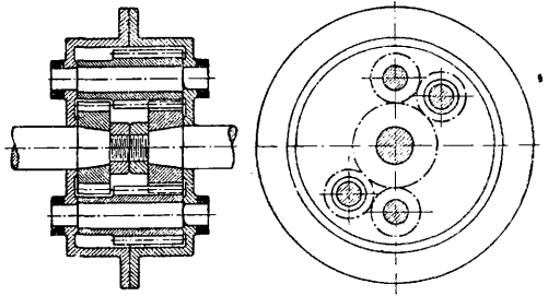
Фиг. 16. Дифференциал с цилиндрическими шестернями.
