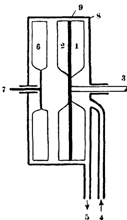
Фиг. 13. Схематич. разрез через камеру прибора Ранарекс.
