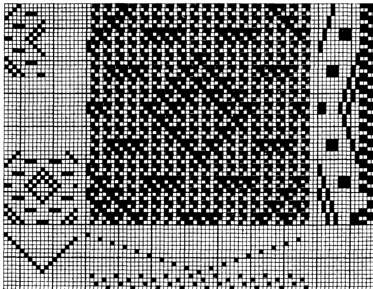
Определение переплетения пикэ.
