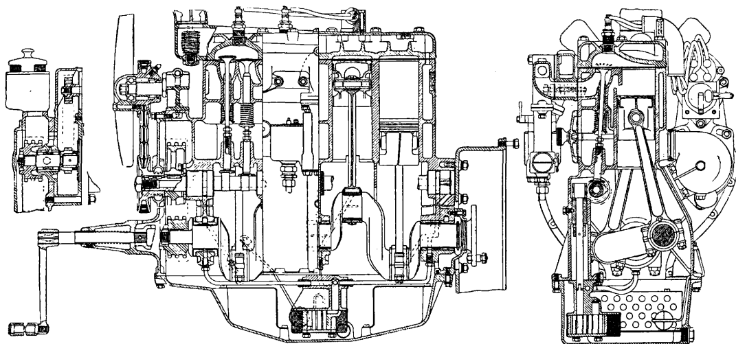
Фиг. 6. Продольный и поперечный разрезы мотора Триумф.
