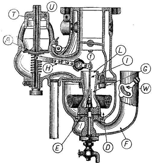
Фиг. 29. Карбюратор Шеблер.
