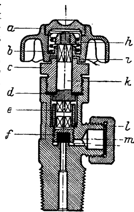
Фиг. 2. Вентиль баллона в разрезе: а — маховичок, б — пружина, с — гайка, d — прокладка, e — муфта, f — уплотняющ. прокладка, g — верхний шпindel, h — шпindel, i — колпачковая гайка, m — манодетандер, n — выступ.
