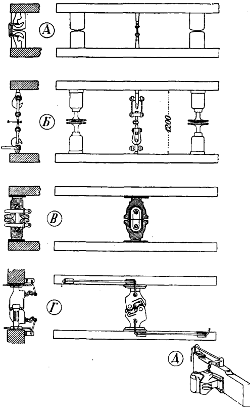
Фиг. 1. Типы сцепок, применявшихся и применяемых на железных дорогах: А — примитивная трехзвенная сцепка, Б — винтовая ж. д. сцепка, В — сцепка «колокол—серьга—штырь», Г и Д — американская сцепка.
