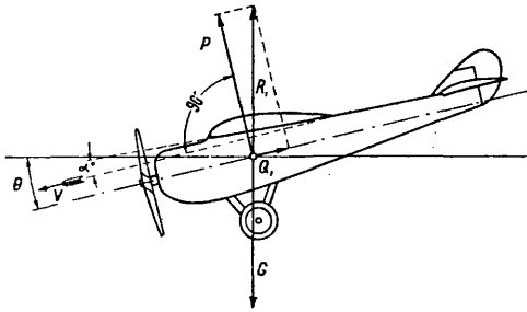
Фиг. 17. Схема усилий в планирующем аэроплане.
