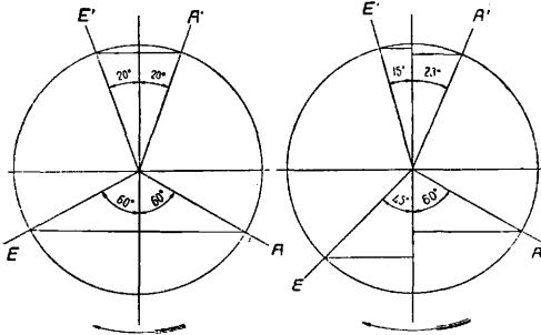
Фиг. 3. Диаграммы распределения мотора: A — начало выпуска, A' — конец выпуска, E' — начало всасывания, E — конец всасывания.
