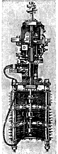
Фиг. 10. Искатель системы Сименс и Гальске.
