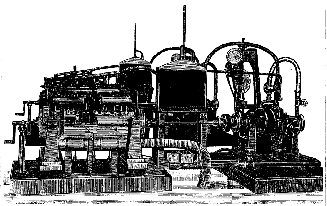
Фиг. 38. Испытательная установка с тормозом Фруд.
