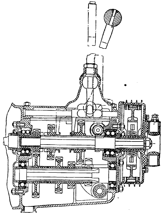
Фиг. 5. Коробка передач легкового автомобиля. груза, работу мотора можно перевести на меньшее число оборотов и полное открытие дросселя, т. е. на более экономичный
