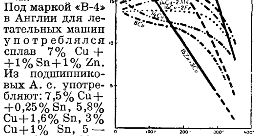
Фиг. 9. Коэфф. крепости при высоких t^{\circ} у различных алюминиевых сплавов, отлитых в кокиль, и у «Силумина», отлитого в песок (Gorson).
