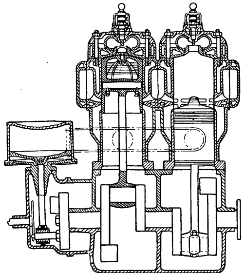
Фиг. 31. Двигатель Тартрэ.
