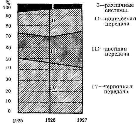
Фиг. 10. Передачи на задние колеса.
