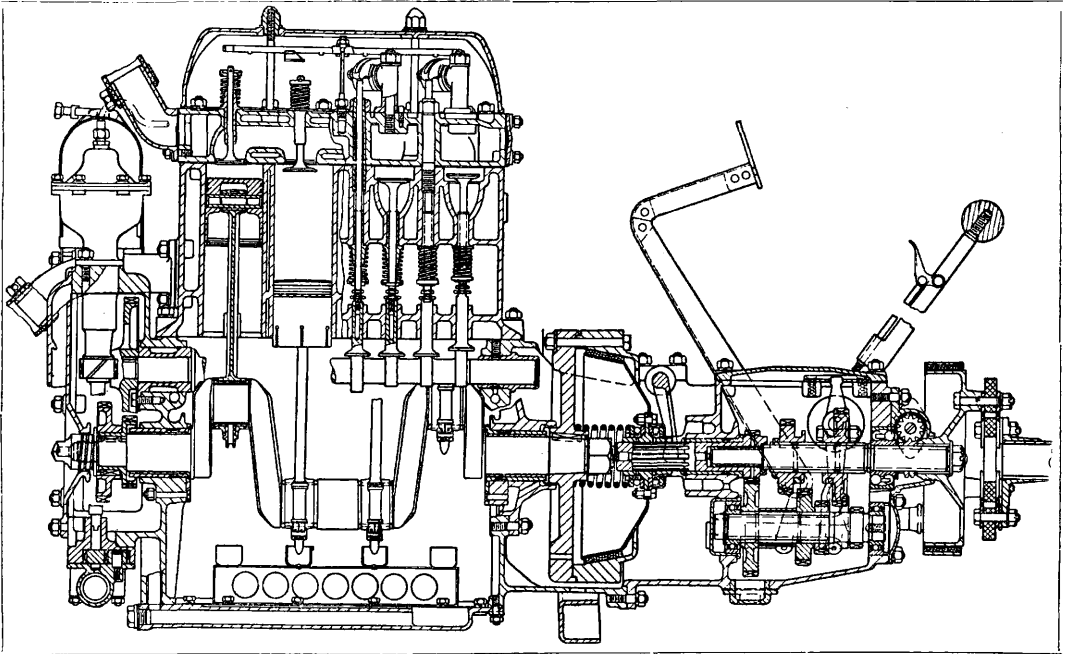
Фиг. 7. Продольный разрез автомобильного мотора Гумбер.
