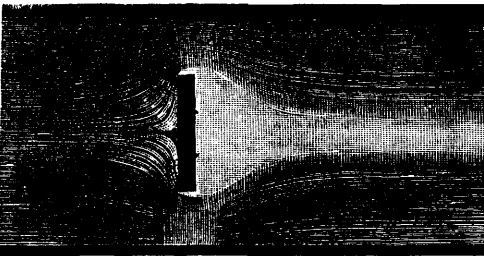
Фиг. 9. Обтекание плоской пластинки на большой скорости.
