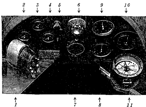
Расположение приборов на самолете: 1—выключатели мотора, 2—манометр для бензина, 3—аэротермометр, 4—манометр для масла, 5—бензиновый насос, 6—переклюатель бензина, 7—поперечный уклономер, 8—тахометр, 9—альтиметр, 10—показатель скорости, 11—компас.
