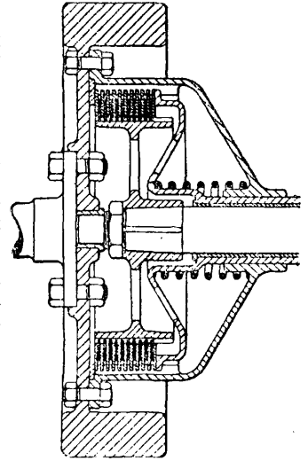
Фиг. 4. Многодисковое сцепление.
