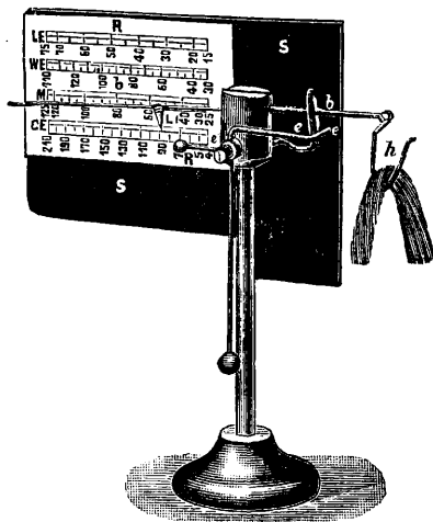
Фиг. 4. Универсальный баланс Штауба.
