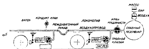
Фиг. 3. Автоматический тормоз.—Схема положения оттормаживания.
