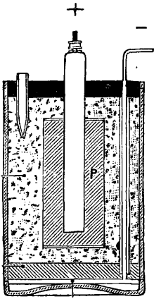
Фиг. 13. Сухой аккумулятор Ферри.
