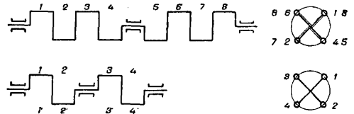
Фиг. 15в. Схема коленчатых валов 8-цилиндр. мотора.
