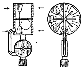
Фиг. 9. Анемометр фирмы Р. Фюс.
