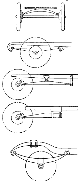
Фиг. 20. Различные типы автомобильных рессор.
