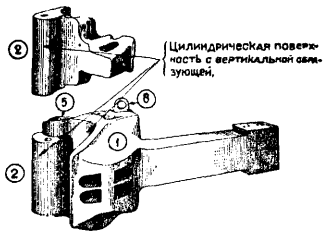
Фиг. 3. Головна американской сцепки.
