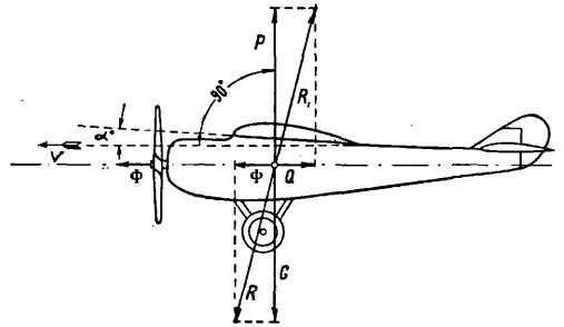
Фиг. 16. Схема усилий в горизонтальном полете аэроплана.
