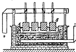
Фиг. 2. Электролитическая ванна: А — угольная набойка, В — электроды.
