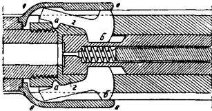
Фиг. 4. Схема винтовки системы Маузера.
