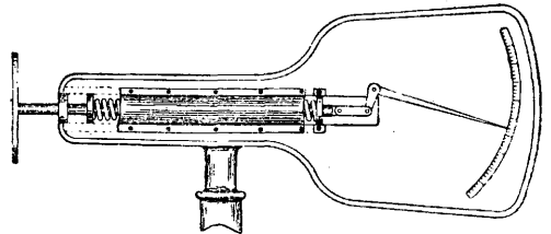
Фиг. 4. Анемометр Ослера.
