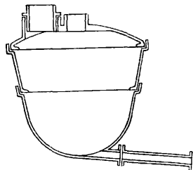
Фиг. 1а. Чугунная реторта установки Гутмана.
