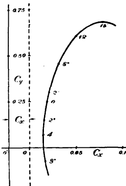
Фиг. 15. Поляра Лилиенталя всего самолета.
