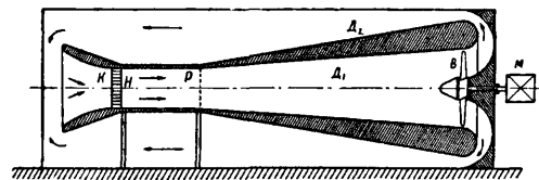
Фиг. 18. Открытая труба (СССР—Англия): К—коллектор, Р—рабочая часть, Д 1 , Д 2 —диффузор, В—вентилятор, М—мотор, Н—направляющая решетка.
