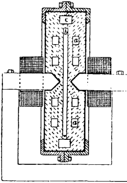
Фиг. 1. Схема печи Биркелянда и Эйде (первоначальная конструкция): а—каналы для притока воздуха, б—камера для вольтовой дуги, с—выход окисленных газов.
