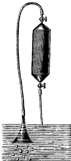
Фиг. 3. Сосуд для отбора пробы в минеральных источниках.
