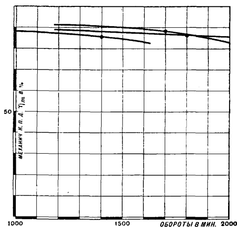
Фиг. 2. Изменение \eta_m с числом оборотов.
