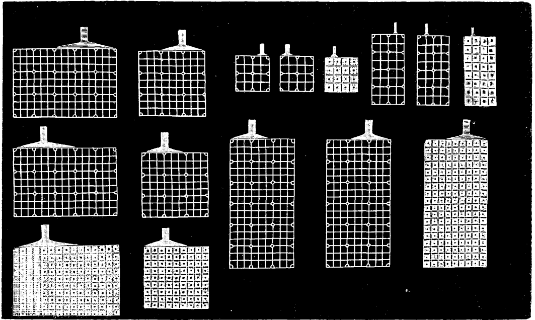
Фиг. 6. Решетки и пластированные пластины фирмы S. A. A. U.
