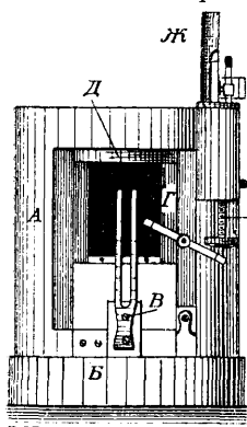
Фиг. 1. Акселерограф Марселя Дебре.
