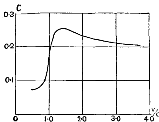
Фиг. 7. Зависимость коэфф. сопротивления от скорости.
