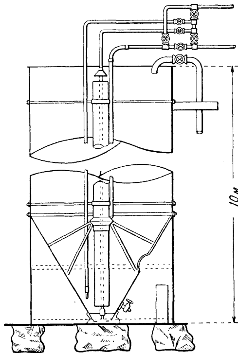
Фиг. 1. Чан для взмучивания шлама.
