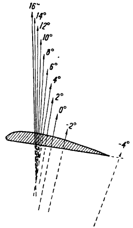
Фиг. 12. Положения равнодействующей на профиле крыла.
