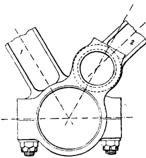
Фиг. 23. Шатунное сочленение на пальце: 1 — главный шатун, 2 — малый шатун.
