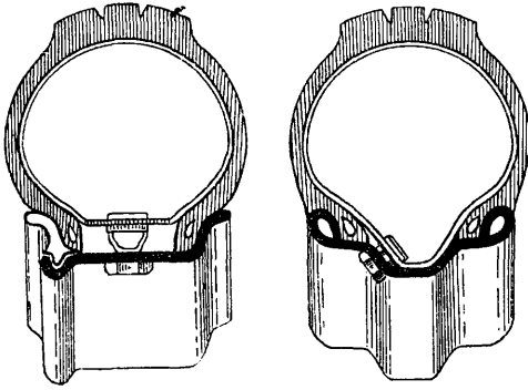
Фиг. 2. Типы безбортовых автошин.
