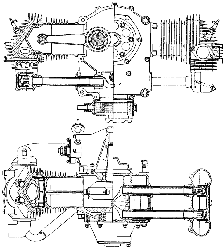
Фиг. 7. Двигатель Бристоль «Cherub III» 30 НР.
