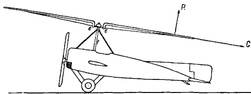
Фиг. 1. Схема бокового вида автожира.
