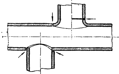
Фиг. 12. Сварка патрубков.
