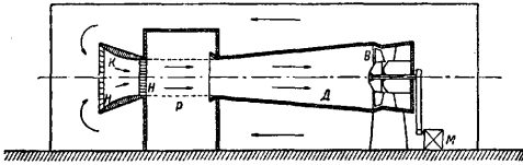
Фиг. 19. Труба Эйфеля (Франция): К—коллектор, Р—рабочая камера, Д—диффузор, В—вентилятор, М—мотор, Н—направляющая решетка.
