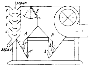
Схематический чертеж аспиратора.
