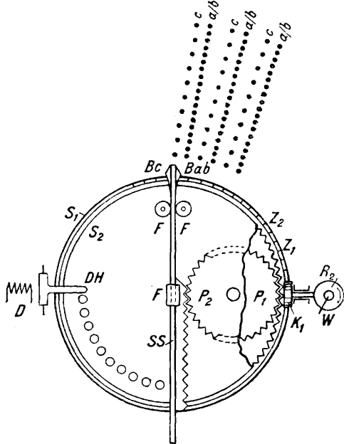
Фиг. 21. Схематический вид искателя системы Эриксона.
