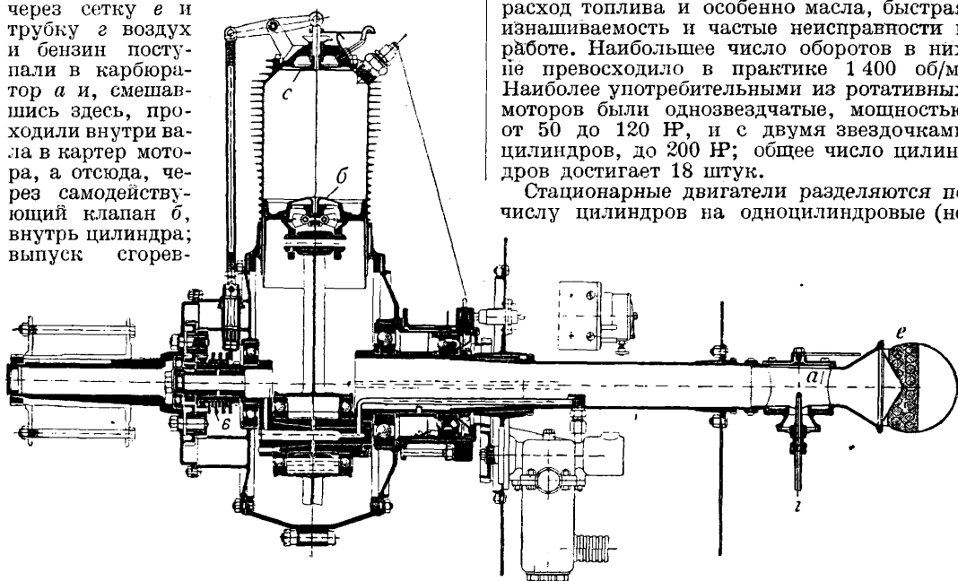
Фиг. 5. Ротативный двигатель Гном.
