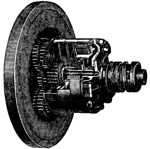
Фиг. 10. Общий вид коробки передач Форда.
