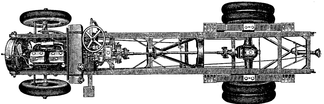
Фиг. 2. Нормальное шасси грузового автомобиля.
