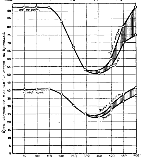
Фиг. 5. Термическая обработка алюмин. сплава «Лауталь» (Fuss u. Bohne).
