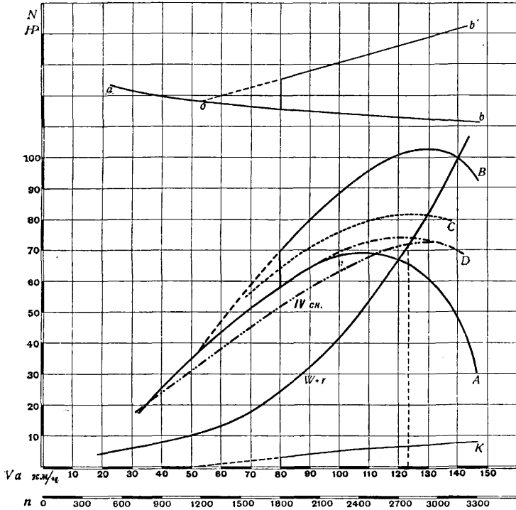
Фиг. 38. Испытание автомобиля Мерседес-Даймлер.
