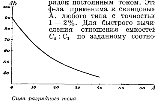
Фиг. 11. Емкость аккумулятора в зависимости от силы разрядного тока (примерная кривая).
