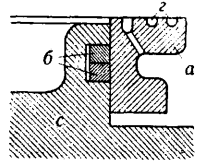
Золотник Адамса.
