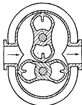
Фиг. 33. Нагнетатель типа Рута.
