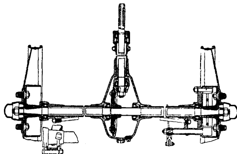
Фиг. 19. Задний мост без дифференциала.
