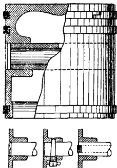
Фиг. 9. Поршень и детали укрепления пальца.
