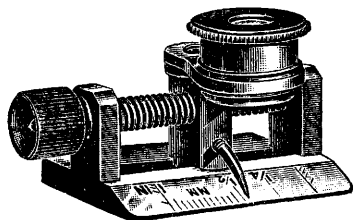
Фиг. 2. Универсальная счетная лупа.
