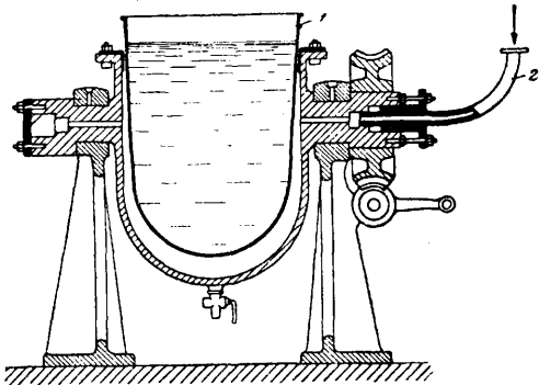
Фиг. 1. Котел для варки аппрета: 1—котел, 2—паропровод.
