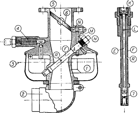
Фиг. 30. Карбюратор Паллас: 1 — поплавок, 2 — подвод воздуха, 3 — уровень бензина, 4 — фильтр для бензина, 5 — смесь, 6 — дроссельная заслонка, 7 — отверстие жиклера.
