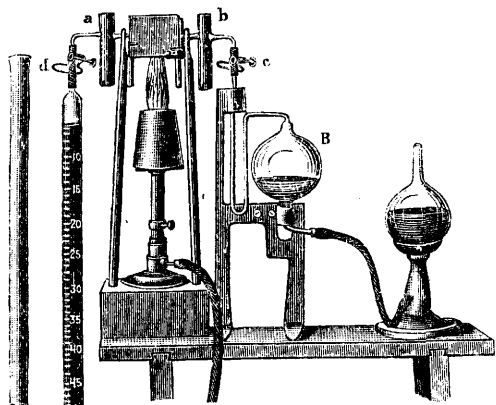
Фиг. 10. Платиновый капилляр Дрешмидта-Виклера.
