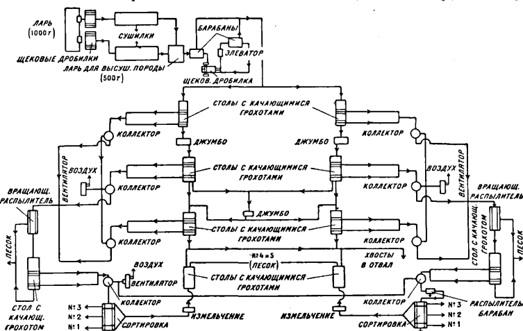
Фиг. 1. Типичная схема обработки продольноволокнистого асбеста.
