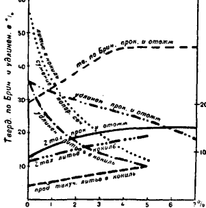
Фиг. 10. Механические качества Al-Ni сплавов (Gorson).
