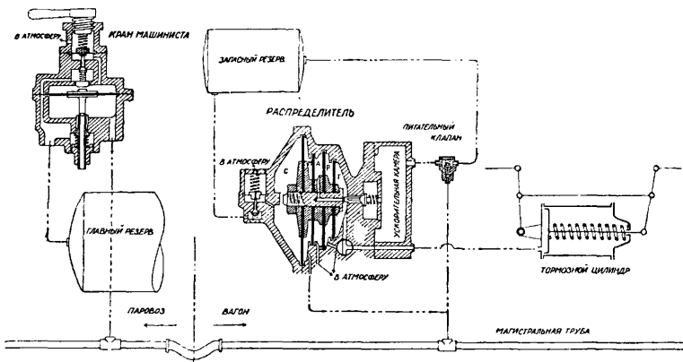
Фиг. 14. Схема расположения приборов двухрежимного тормоза Казанцева.
