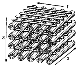
Модель среды, обладающей по трем взаимно перпендикулярным направлениям проводимостями различного характера: 1—металлического, 2—электролитического (или электроосмотического) и 3—газового.
