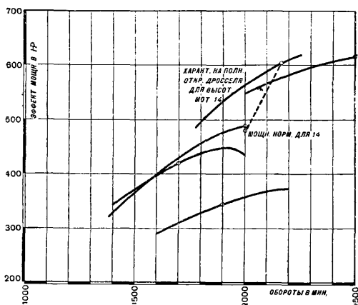
Фиг. 1. Внешняя характеристика авиационного двигателя.
