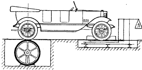
Фиг. 32. Станок Ридлера (поперечный разрез).
