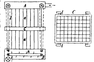
Фиг. 2. Схематический чертеж фильтра.
