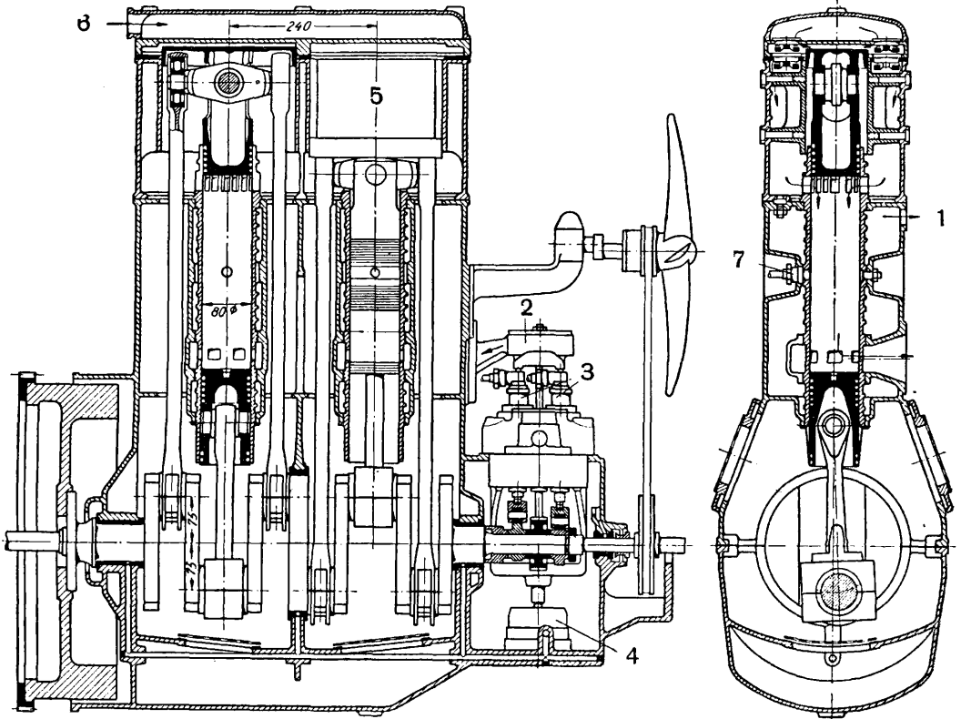
Фиг. 32. Двигатель Юнкер: 1—выход охлаждающей воды, 2—водяной насос, 3—насосы для подачи горючего, 4—масляный насос, 5—насос для продувки, 6—воздух для продувки, 7—форсунка.
