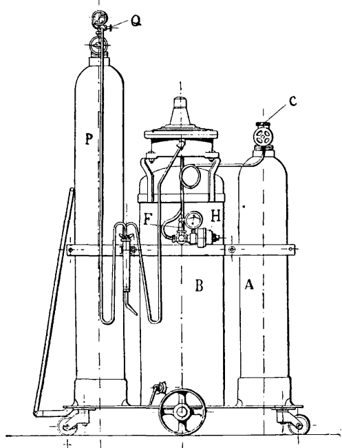
Фиг. 14. Передвижной сварочный аппарат: А—баллон с блаугазом, В—газоборник (расширитель), С—бутылочный вентиль, F—обратный клапан, Н—предохранительный клапан, P—кислородная бутылка, Q—редуктор для кислорода.
