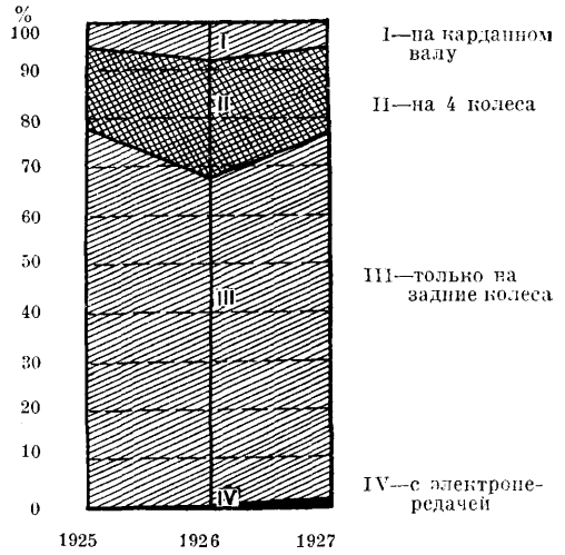
Фиг. 4. Полные тормоза.
