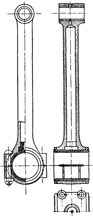
Фиг. 13. Шатун из дуралюминия.
