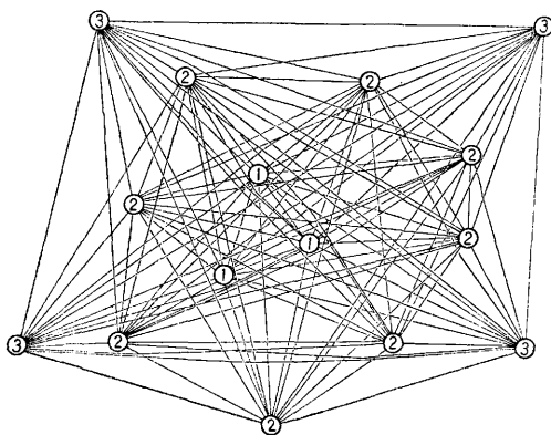
Фиг. 5. Телефонная сеть при ручном обслуживании.
