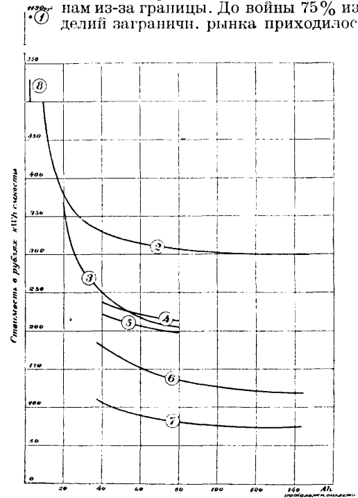
Фиг. 19. Стоимость кВт·ч емкости щелочных и кислотных аккумуляторов разных типов. Щелочные А.: 1—радиобатарея, 2—емкостный. Свинцовые А. разных типов производства Аккумуляторного треста СССР: 3, 4 и 5—типа Ц.В., 6—Г.О., 7—К., 8—Р.Г.
