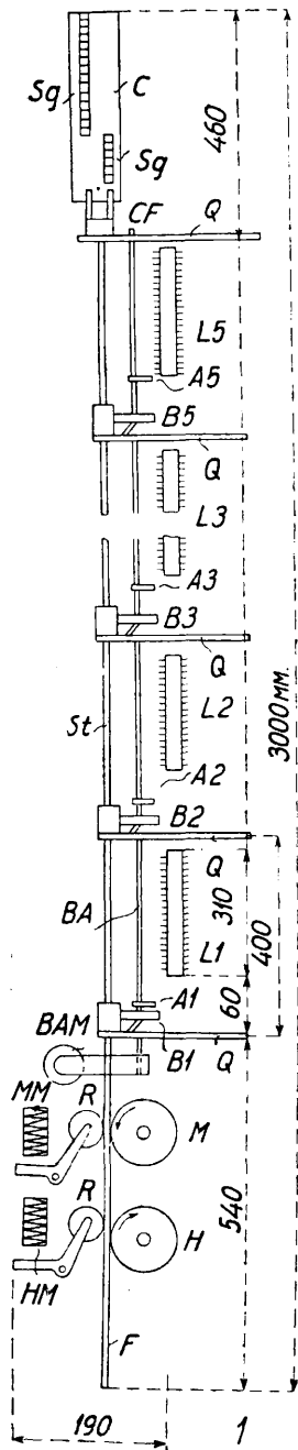
Фиг. 14. Линейный искатель Вестерн.
