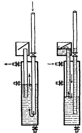
Фиг. 7. Схема водяного затвора: слева — в состоянии нормальной работы, справа — в случае обратного удара (при взрывах и выпешках).
