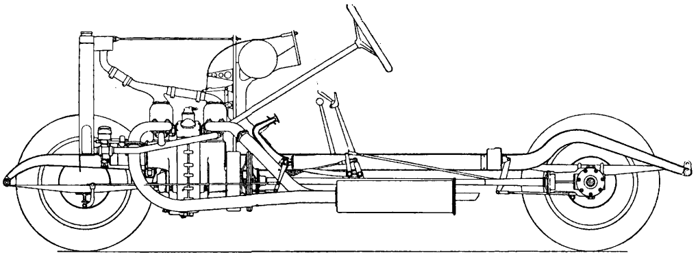
Фиг. 40. Шасси автомобиля Константиנסко (общий вид).
