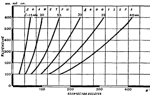
Фиг. 27. Расход воздуха через диффузор карбюратора.
