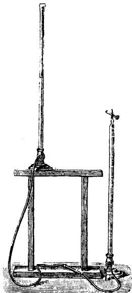
Фиг. 6. Газовая бюретка Гемпеля.
