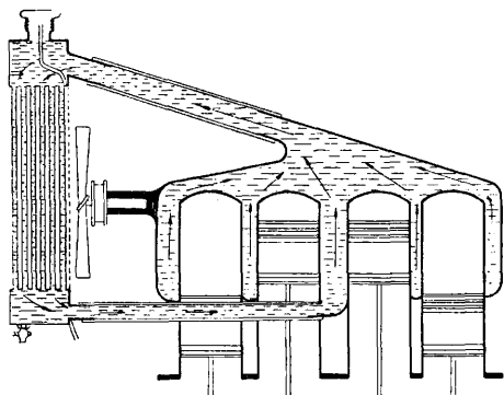
Фиг. 18. Схема термосифонного охлаждения.
