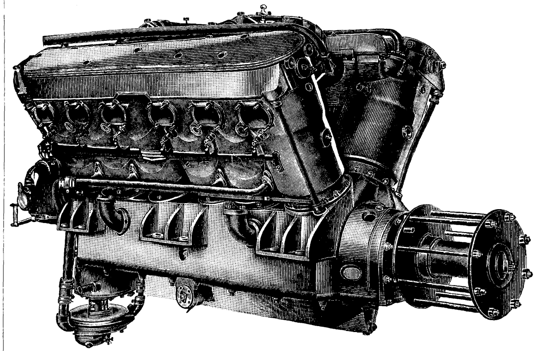
Фиг. 9. 12-цилиндровый двигатель Райт 600 HP.
