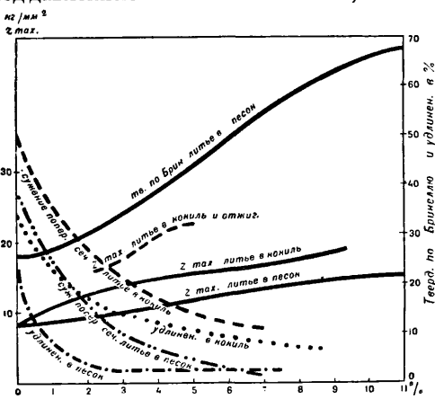
Фиг. 8. Механич. качества Al-Cu литых сплавов (Gorson).
