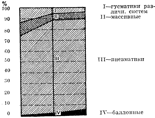
Фиг. 7. Шины передние и задние.
