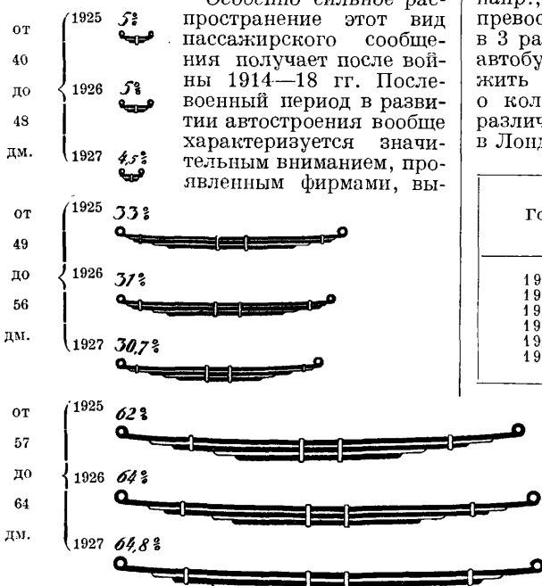
Фиг. 5. Длина задних рессор.
