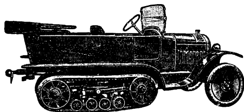
Фиг. 1. Автомобильные сани Кегресс фирмы Ситроэн.
