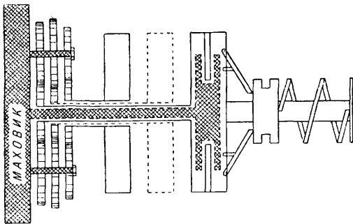
Фиг. 8. Схема коробки передач Форда.
