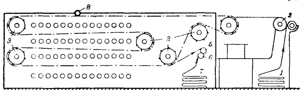
Фиг. 5. Сушильно-ширильный станок (шпан-рама): 1 — влажная ткань, 2 — расширительный валик, 3 — цепные барабаны, 5 и 6 — натяжные ролики, 7 — высушенная ткань, 8 — ролик-щетка.
