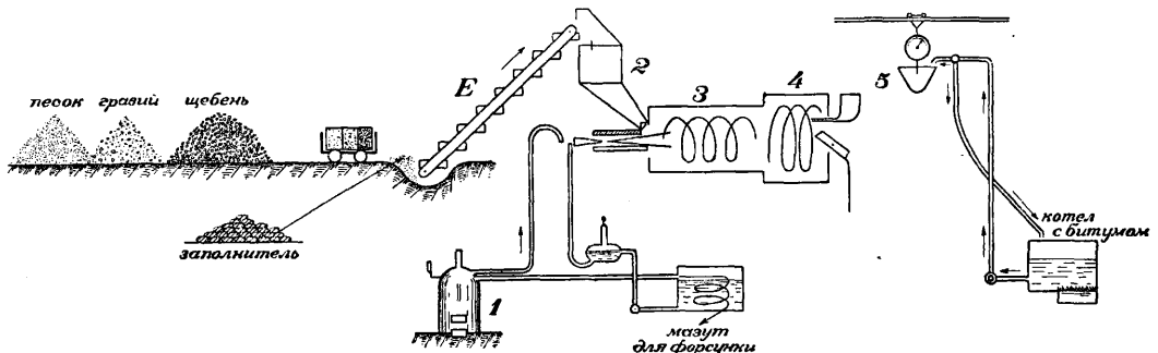
Схема производства асфальтового бетона.
