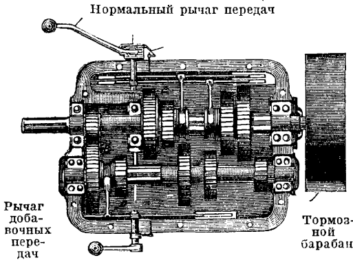
Фиг. 7. Коробка скоростей с добавочной передачей. Когда включена постоянная передача C+D, то 1-я передача становится 5-й, 2-я передача становится 6-й, 3-я передача становится 7-й.
