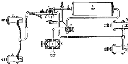
Фиг. 28. Пневматический тормоз.
