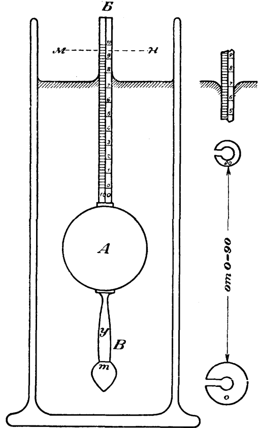
Фиг. 2. Металлический спиртомер.
