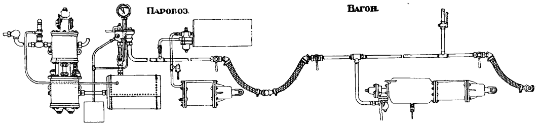
Фиг. 6. Схема расположения приборов тормоза Вестингауза.
