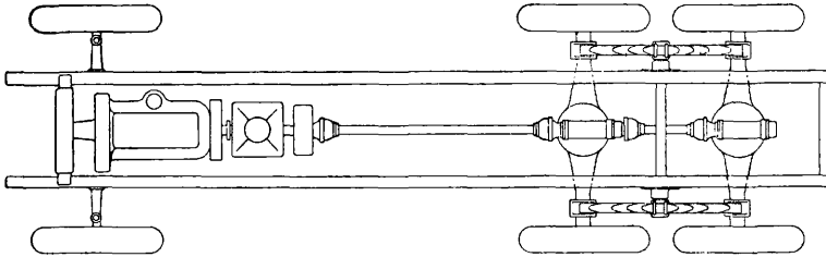
Фиг. 44. План шасси трехосного автомобиля.
