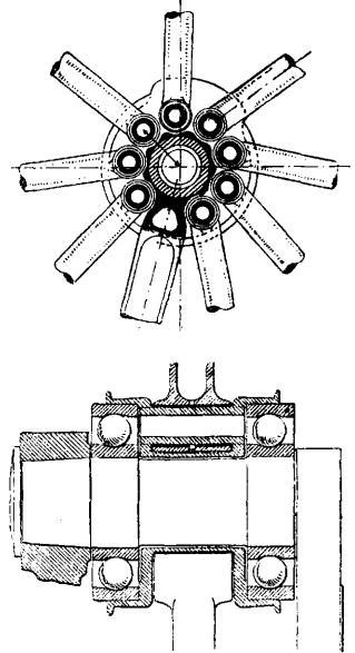
Фиг. 24. Шатунное сочленение на пальцах для звездообразных двигателей.
