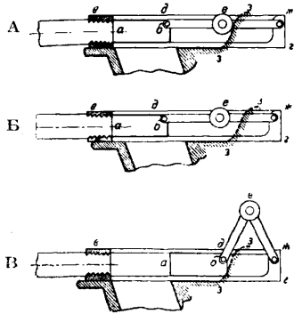
Фиг. 8. Схема автоматического пистолета Борхардта-Люгера: А—положение до выстрела, Б—положение при начале открывания затвора, В—положение после выстрела.
