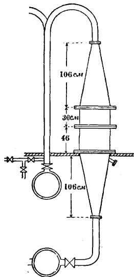
Фиг. 10. Схема окисления аммиака.
