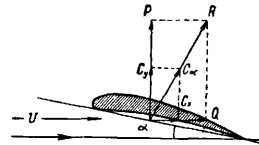
Фиг. 10. Схема разложения силы действия на крыло.
