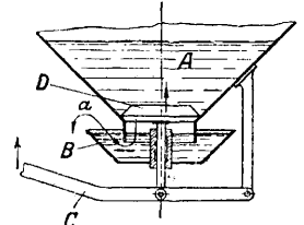
Фиг. 6. Приспособление для спуска известкового шлама (спускной клапан): А — нижняя часть ацетиленового аппарата, В — воронка, С — рычаг для подъема и опускания клапана, а — направление движения спускающего шлама, D — клапан.
