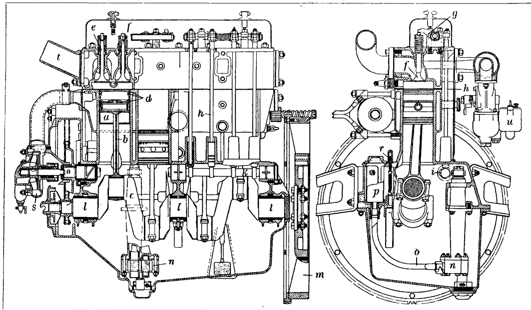
Фиг. 5. Автомобильный мотор с верхними клапанами.
