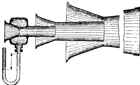
Фиг. 6. Мультипликатор Бурдона.
