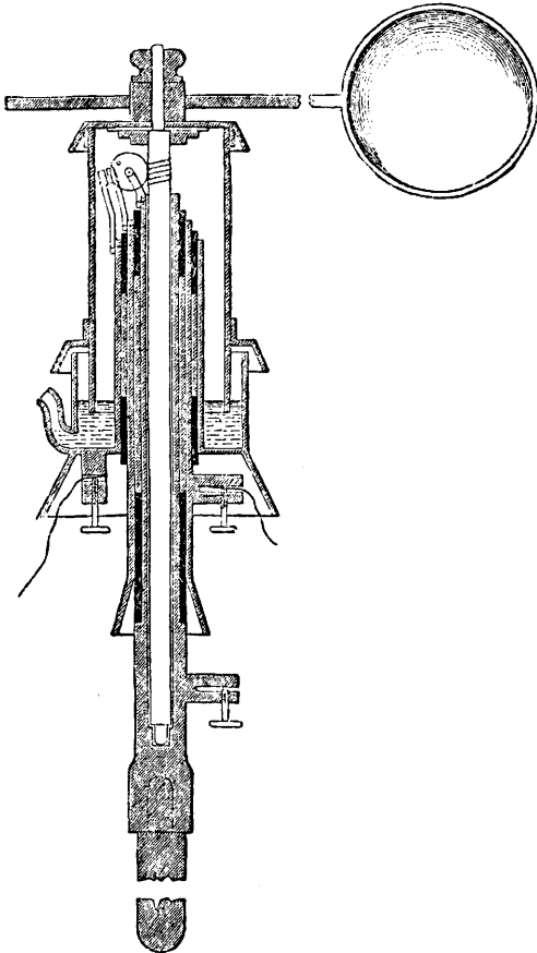
Фиг. 2. Шаровой анемометр Робинсона.
