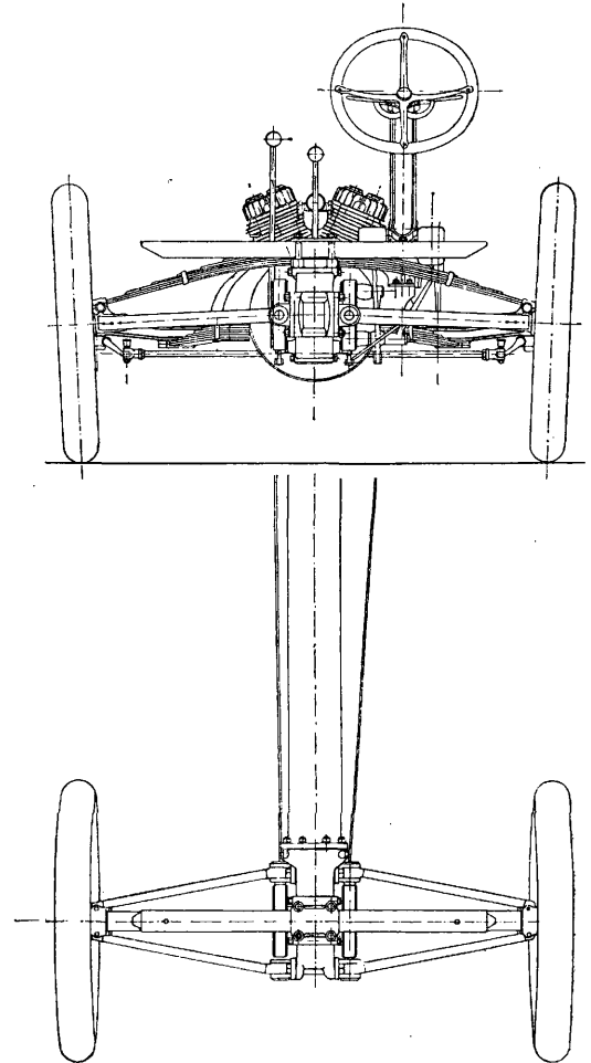
Фиг. 23. Задний мост с разрезной осью автомобиля НАМИ I.
