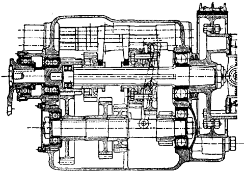
Фиг. 6. Коробка передач грузового автомобиля.
