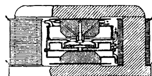
Фиг. 6. Печь Мосъцицкого.
