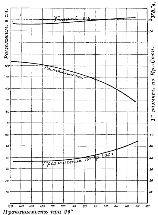
Фиг. 1. Свойства мексиканского остаточного асфальта.
