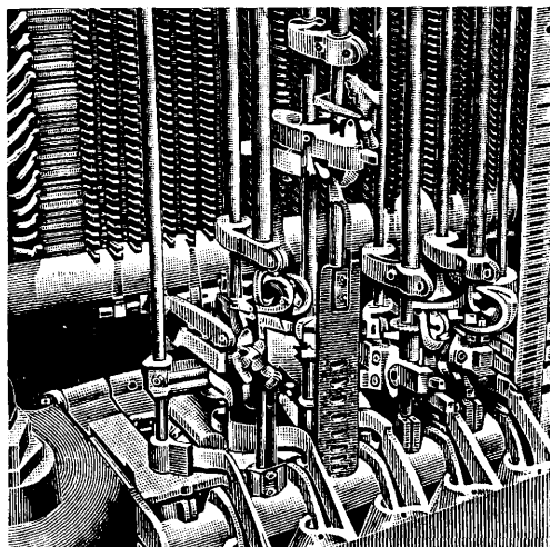
Фиг. 13. Штанговый искатель Вестерн (ниж. часть).
