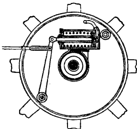
Фиг. 28а. Пневматический тормоз.—Действие на колесо.
