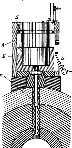
Фиг. 2. Акселерограф Марселя Дебре, установленный на стволе орудия.
