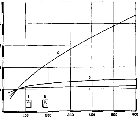
Фиг. 28. Расход топлива через жиклер с изменением разрежения: Q = \psi \sqrt{2gH} — расход топлива, \psi — коэфф. расхода, H — величина разрежения, в метрах водяного столба, f — площадь отверстия жиклера.
