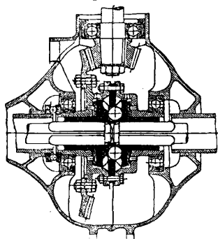
Фиг. 17. Дифференциал Флешера.
