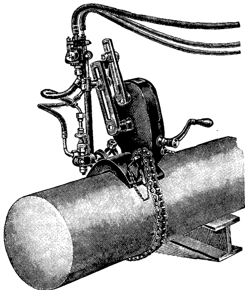
Фиг. 4. Машина для резки валов.
