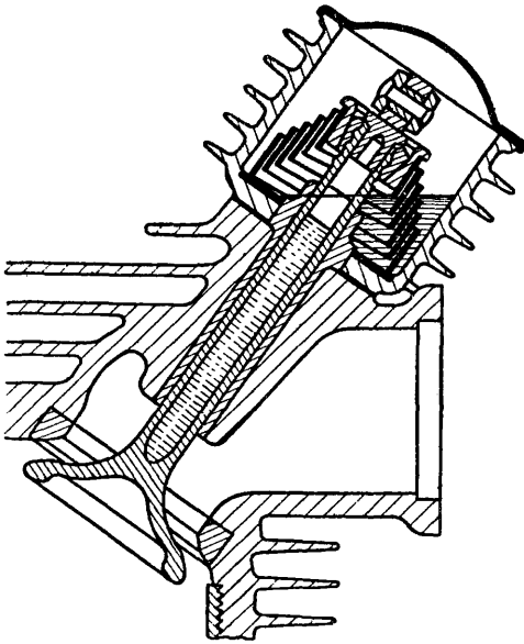
Фиг. 18а. Деталь клапана с охлаждением.
