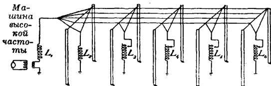
Фиг. 11. Многократная антенна (станции Нью-Брунсвик, С.-А. С. Ш.).
