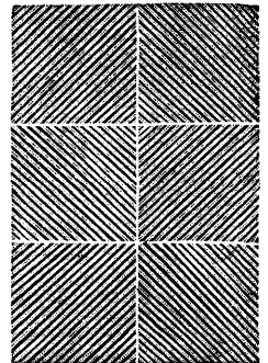
Фиг. 4. Поверхностная однородная пластина Пфаффа, полученная отливкой, с ребрами, наклоненными на 45°.
