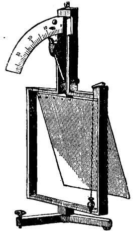
Фиг. 3. Анемометр Вильда.
