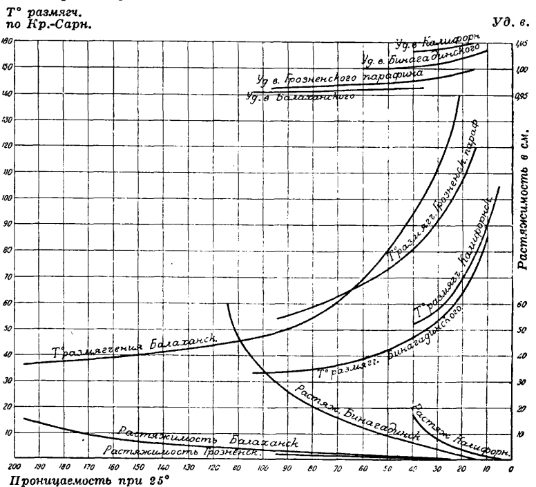
Фиг. 3. Свойства продувочных асфальтов.
