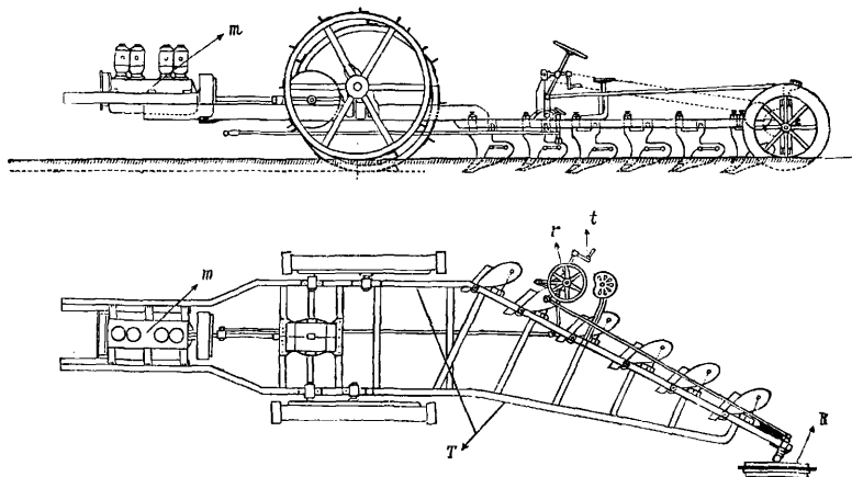
Фиг. 1. Автопflug завода Штока (шток-мотор).
