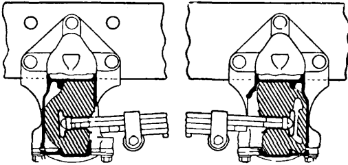
Фиг. 22. Крепление рессоры на резине.
