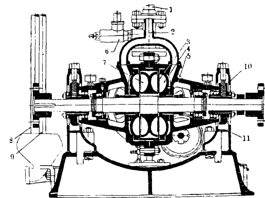
Фиг. 37. Поперечный разрез тормоза Фруд: 1 — выпускной кран, 2 — выпуск воды, 3 — заслонка, 4 — проход для воды 5 — очертание кожуха, 6 — вспомогательный кран, 7 — ротор, 8 — выпускная труба, 9 — вспомогательная труба, 10 — подшипник, поддерживающий кожух, 11 — коренной подшипник.
