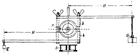
Фиг. 36. Тормоз Прони.
