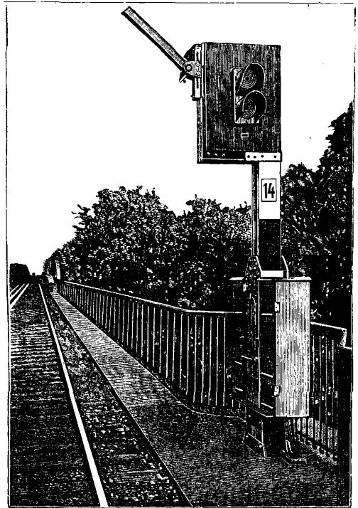
Фиг. 1. Путевой семафор для механич. А. п.
