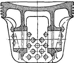
Фиг. 19. Алюминиевый поршень Ринардо (общий вид).
