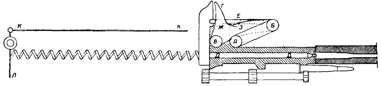
Фиг. 2. Схема пулемета системы Шварцлозе. — Положение частей при закрытом затворе и спущенном ударнике.
