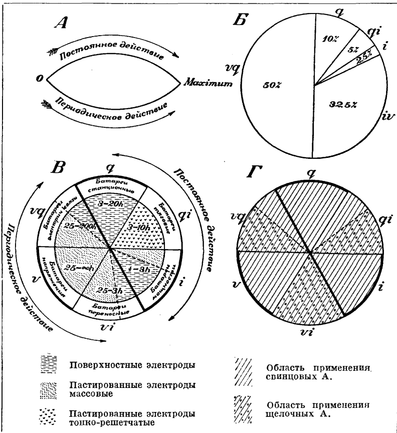
Фиг. 1. Диаграммы функциональной классификации А.
