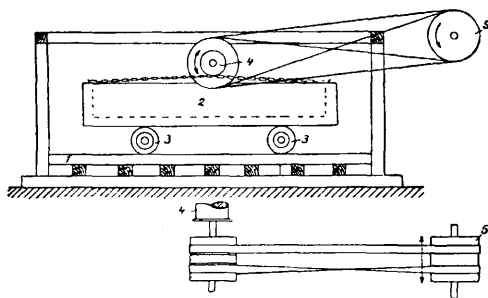
Фиг. 7. Каток ящичный: 1—стол для катания, 2—натальный ящик, 3—катки, 4—цепной барабан, 5—приводной шкив.
