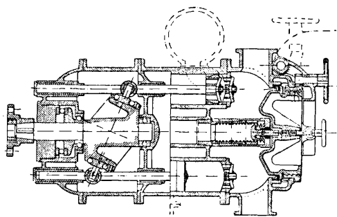
Фиг. 49. Автомобильный пожарный насос.
