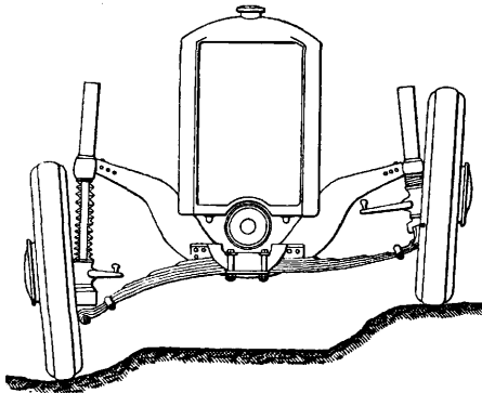
Фиг. 21. Подвеска передних колес автомобиля Коттен-Дегут.
