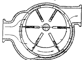
Фиг. 32. Коловратный нагнетатель.
