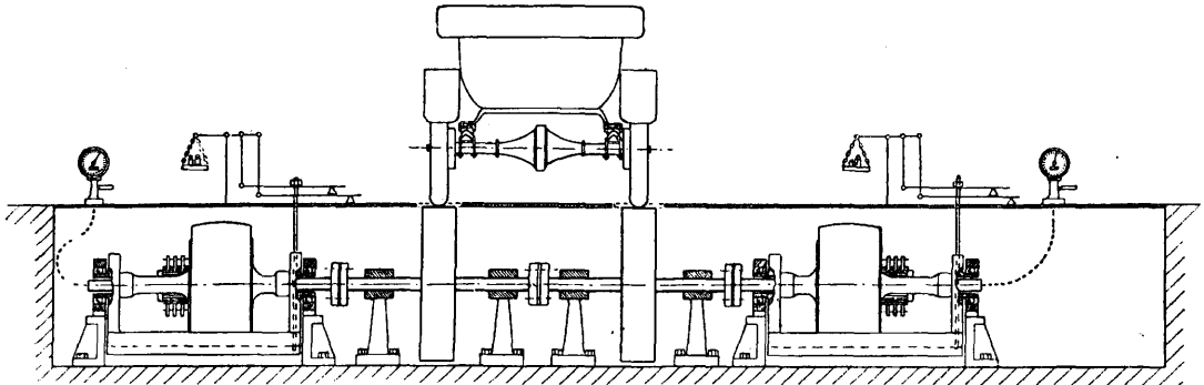
Фиг. 31. Станок Ридлера (продольный разрез).
