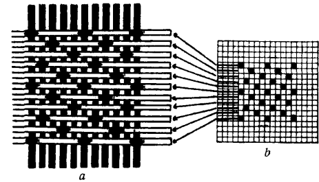
Фиг. 3. Определение атласного переплетения (уточного): a —строение ткани, b —графическое изображение переплетения.
