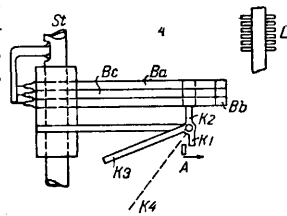
Фиг. 17. Линейный искатель Вестерн.
