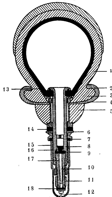
Фиг. 1. Поперечный разрез монтированной А.: 1—покрышка, 2—борт обода, 3—борт покрышки, 4—металлический обод, 5—деревянный обод, 6—медная прокладка, 7—кожаная прокладка, 8—тепло вентиля, 9—резиновая прокладка, 10—игла, 11—коляк вентиля, 12—болт, 13—камера, 14—резиновая прокладка, 15—коляк, 16—клапан, 17—трубка, 18—резиновая шайба.
