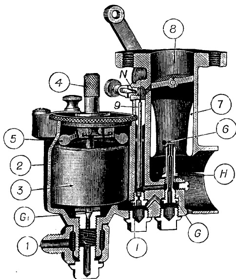
Фиг. 26. Карбюратор Зенит.
