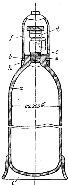
Фиг. 1. Разрез стального баллона: а — стальная труба, б — горловина, с — газовая нарезка, d — бутылочный вентиль (материал — пресованная латунь), f — предохранительный клапан, h — крепительное кольцо, i — пята.
