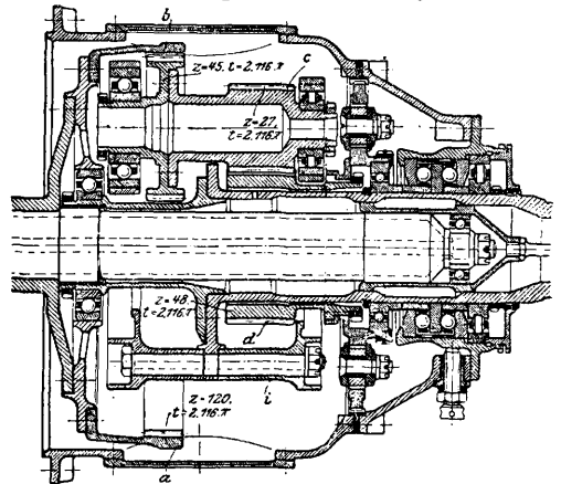
Фиг. 29. Планетарный редуктор двигателя Рольс-Ройс 300 НР.
