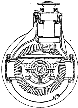
Фиг. 14. Карданная и коронная шестерни с непересекающимися осями.
