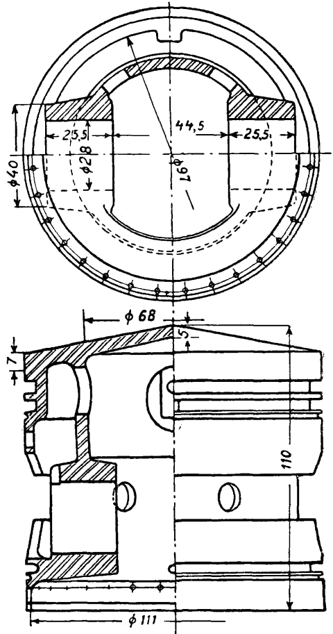
Фиг. 20. Поршень мотора Рольс-Ройс (детальный вид).
