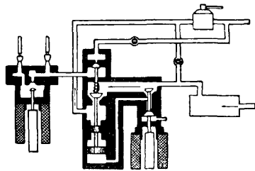
Фиг. 4. Прибор, приводящий в действие непрерывные тормоза.
