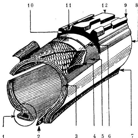
Фиг. 4. Пневматическая автошина: 1—крыло бортовой покрышки, 2—сердечник безбортовой покрышки, 3—каркас, 4—прокладка, 5—буфер, 6—подпротектор, 7—бортовая ленточка, 8—боковая часть, 9—боковая дорожка, 10—протектор, 11—канавка, 12—центровая дорожка.
