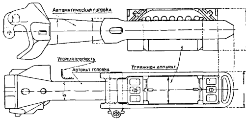
Фиг. 8. Комплектный американский автоматический сцепной прибор с упругим аппаратом.
