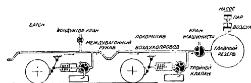
Фиг. 4. Автоматический тормоз.—Схема положения торможения.
