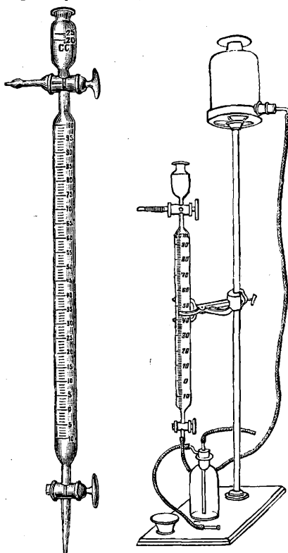
Фиг. 5. Газовая бюретка Бунте.
