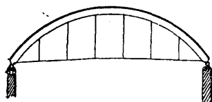
Фиг. 3. Стропильная арка с затяжкой.
