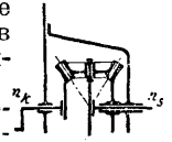
Фиг. 28. Схема конического редуктора.
