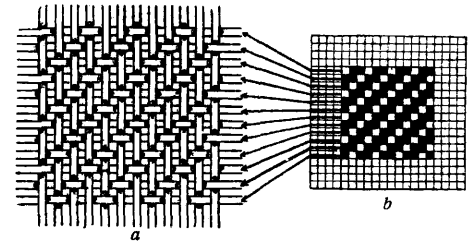
Фиг. 2. Определение саржевого переплетения: a —строение ткани, b —графическое ее изображение.
