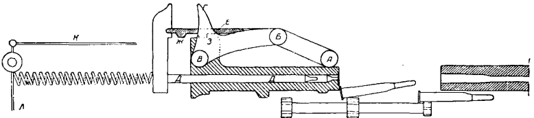
Фиг. 3. Схема пулемета системы Шварцлозе. — Положение после выстрела, затвор в крайнем заднем положении, ударник взведен, пружина сжата.
