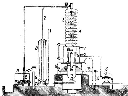
Фиг. 1. Установка Грюнберга и Блюма.
