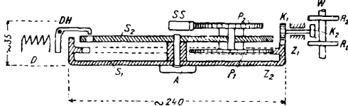
Фиг. 22. Схема разреза искателя системы Эриксона.
