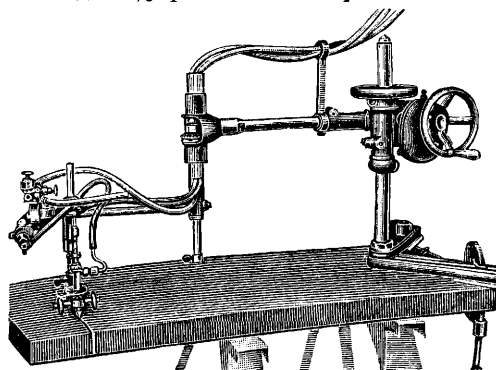
Фиг. 5. Машина для циркульной резки.
