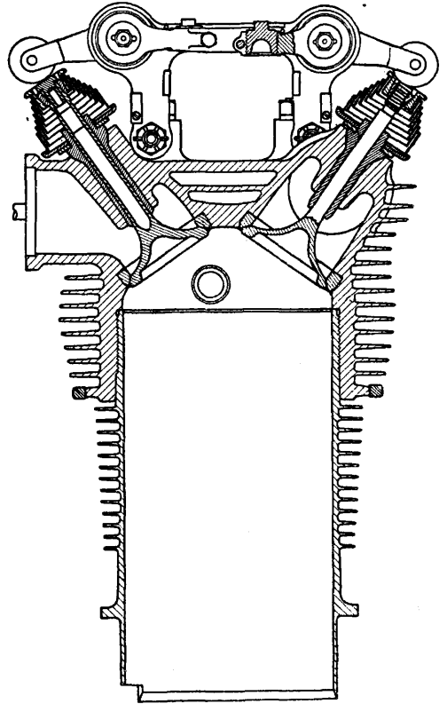
Фиг. 18. Цилиндр типа J.
