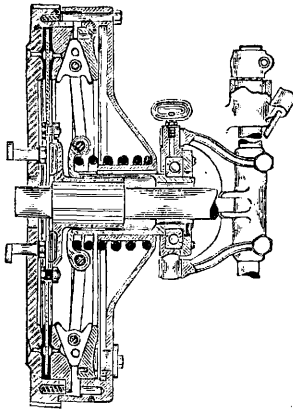
Фиг. 3. Однодисковое сцепление.
