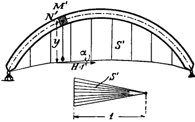
Фиг. 24. Многоугольник сил при условии H=1 .
