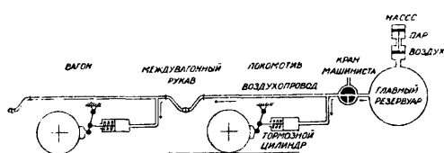
Фиг. 2. Неавтоматический тормоз.—Схема положения торможения.
