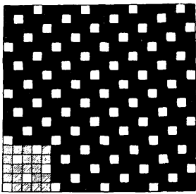
Строение основного атласного переплетения (атлас %).
