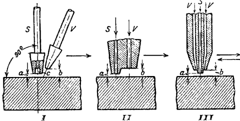
Фиг. 1. Горелки резаков различных конструкций. I—эксцентрическое расположение сопел, II—параллельное » » » III—концентрическое » » » S—кислородное сопло, V—водородное сопло, а и б—расстояние до объектов резки.
