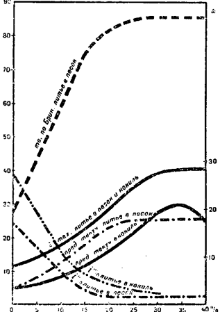
Фиг. 6. Механические качества литых Al-Zn сплавов (Rosenhain u. Archibutt).
