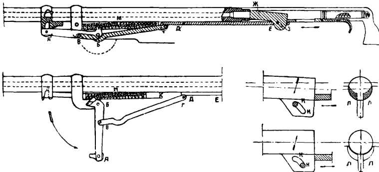
Фиг. 13. Схема пулемета системы Кольта: вверху — положение перед выстрелом, внизу — положение после выстрела.
