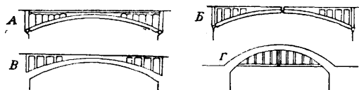
Фиг. 2. Примеры сплошных мостовых арочных ферм: А — двухшарнирная сплошная арка, Б — трехшарнирная сплошная арка, В — бесшарнирная сплошная арка, Г — железобетонная арка с подвешенным мостовым полотном.
