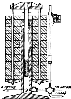
Фиг. 1. Прямой гидравлический аккумулятор.
