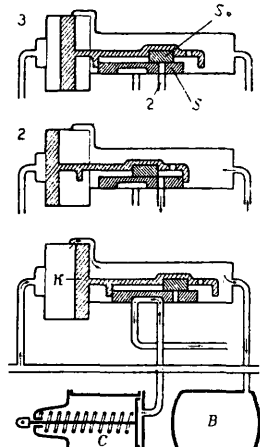
Фиг. 5. Схема тройного клапана: 1 — отпуск, после отпуска и зарядки, 2 — торможение и после полного торможения, 3 — после неполного торможения.
