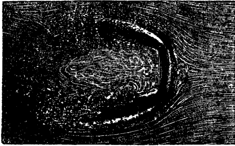
Фиг. 14. Спектр Рябушинского. Обтекание плоской пластинки.
