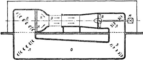
Фиг. 20. Замкнутая труба Прандтля (Германия): К—коллектор, Р—рабочая часть (открытая), В—вентилятор, Л—направляющие лопатки, О—обратный канал, М—мотор, Н—направляющая решетка.
