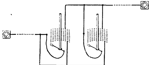
Фиг. 2. Искатель системы Струуджера с сотенными группами.
