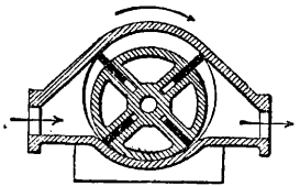
Фиг. 31. Коловратный масляный насос.
