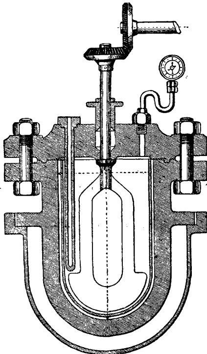
Автоклав.
