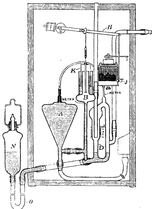
Фиг. 11. Схема установки саморегистрирующего газоанализатора Адос.
