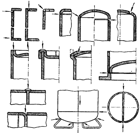
Фиг. 11. Сварка днщ и перегородок. (Стрелки показывают места сварки.)
