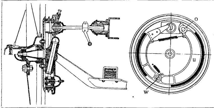
Фиг. 27. Серво-тормоз Перро.
