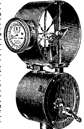
Фиг. 8. Анемометр фирмы Р. Фюс.
