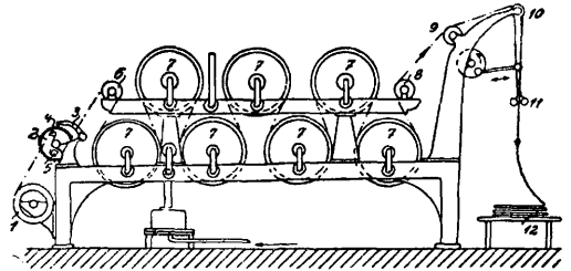
Фиг. 3. Сушильные барабаны: 1—навои поступающей ткани, 2 и 3—храновик, 4 и 5—направляющие ригеля, 6 и 8—расправители, 7—сушильные барабаны, 9—направляющий ролик, 10 и 11—приспособление для складывания ткани, 12—стол для укладки высушенной ткани.
