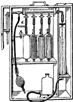
Фиг. 7. Аппарат Орса-Лунге.
