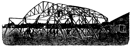
Фиг. 1. Переносный ангар Бессона.
