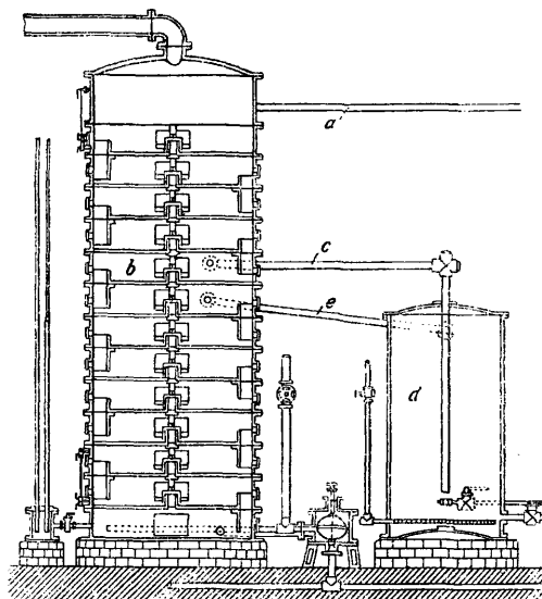
Фиг. 2. Установка Вильтона.
