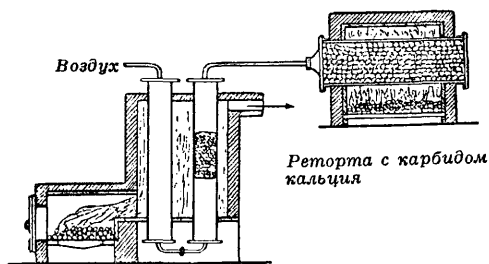
Фиг. 1. Печь для получения азота с ретортой для приготовления кальций-цианмида.
