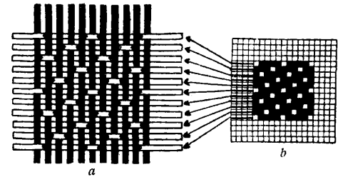
Фиг. 4. Определение атласного переплетения (основного): a —строение ткани, b —графическое изображение переплетения.
