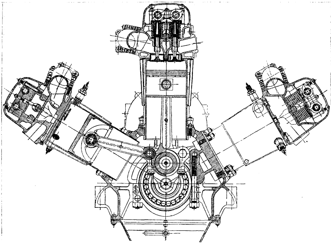
Фиг. 11. Поперечный разрез двигателя Непир «Lion» 450 HP.
