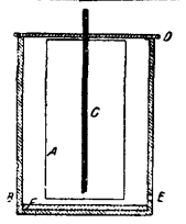
Фиг. 2. Схема азотирования карбида по Франку и Каро: А — перфорированный короб с молотым карбидом, В — шпатовая азотирующая печь, С — угольный электрод, 1 см., D — плотная крышка, E — приток азота, F — другой электрод.
