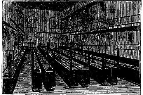
Фиг. 21. Общий вид стационарной аккумуляторной батареи.
