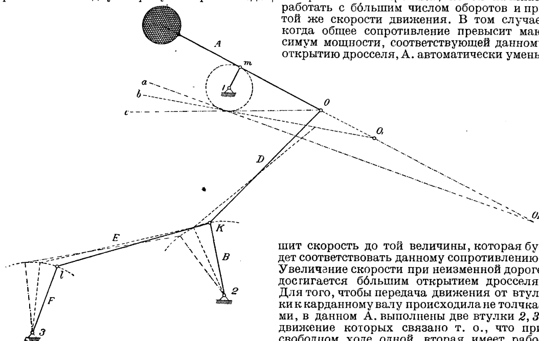
Фиг. 41. Схема действия коробки скоростей в автомобиле Константинеко.
