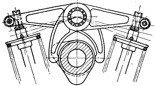
Фиг. 16. Клапан и привод к нему с верхним расположением кулачкового вала.
