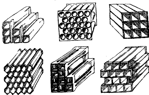
Фиг. 21. Детали сотовых радиаторов.
