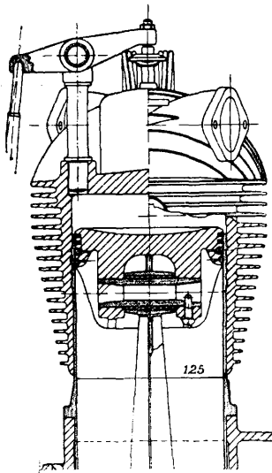
Фиг. 17. Цилиндр двигателя НАМИ 100 Я.
