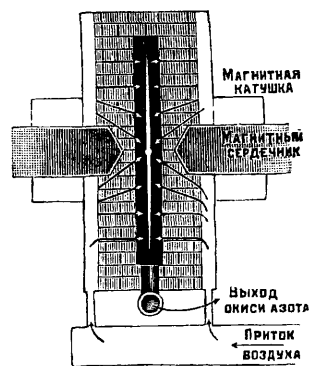
Фиг. 2. Печь Биркелянда.
