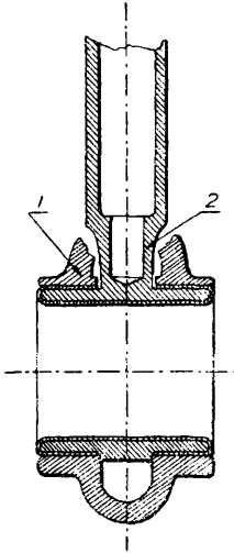
Фиг. 21. Шатунное сочленение: 1 — наружный вильчатый шатун, 2 — внутренний шатун.
