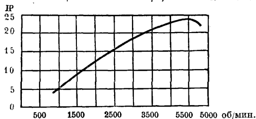
Фиг. 2. Характеристика мотора Блекборн 20 HP с авиатки «Буревестник».
