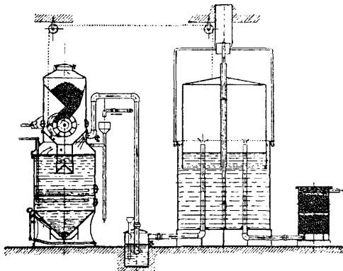
Фиг. 5. Схема ацетиленового аппарата.
