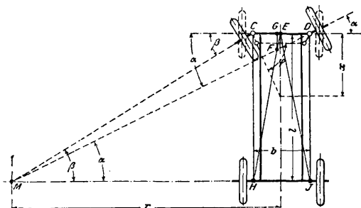
Фиг. 18. Схема четырехугольника Жанто.
