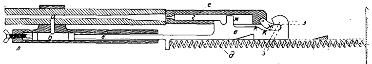
Фиг. 12. Схема пулемета системы Гочкиса.
