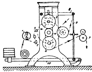
Фиг. 6. Каландр: 1, 2 и 3 — натяжные ригеля, 4 — металлический вал, 5 и 6 — картонные валы, 7 — отводящий вал, 8, 9 и 10 — рычажное приспособление.
