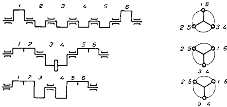
Фиг. 15б. Схема коленчатых валов 6-цилиндр. мотора.
