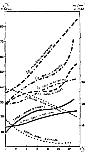
Фиг. 4. Механич. качества сплавов Al-Si (Gorson).
