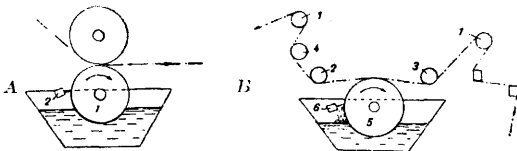
Фиг. 2. Крахмальные плюсовки одностороннего действия: А: 1—вал, подающий аппрет, 2—ракия; В: 1, 2, 3, 4—направляющие ролики, 5—вал, подающий аппрет, 6—ракия.
