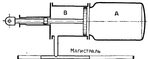
Фиг. 7. Схема двукамерного тормоза.
