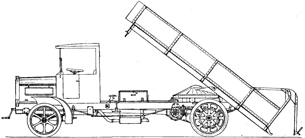
Фиг. 39. Грузовик с поднимающейся платформой.
