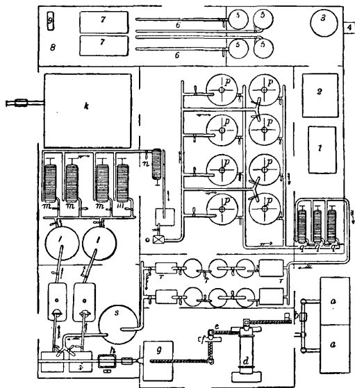
Фиг. 1. Схема завода сернокислого алюминия: а—склад боксита, б—вагон, в—весы, г—резервуар для едкого натра, д—упариват. чаша, е—установка для сушки, ж—склад глинозема, з—бак для кислоты, и—подъемник, к—чаны для растворов, л—кристаллизационная мастерская, м—склад Al_2(SO_4)_3 , н—упаковочное отделение, о—дезинтегратор. Стрелками обозначен последовательный ход обработки боксита (сырой бокситный щелок → алюминатный щелок → разбавл. раствор едкого натра → концентр. раствор едкого натра).
