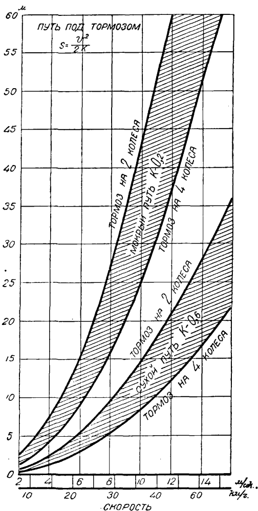
Фиг. 25. Диаграмма пути торможения.
