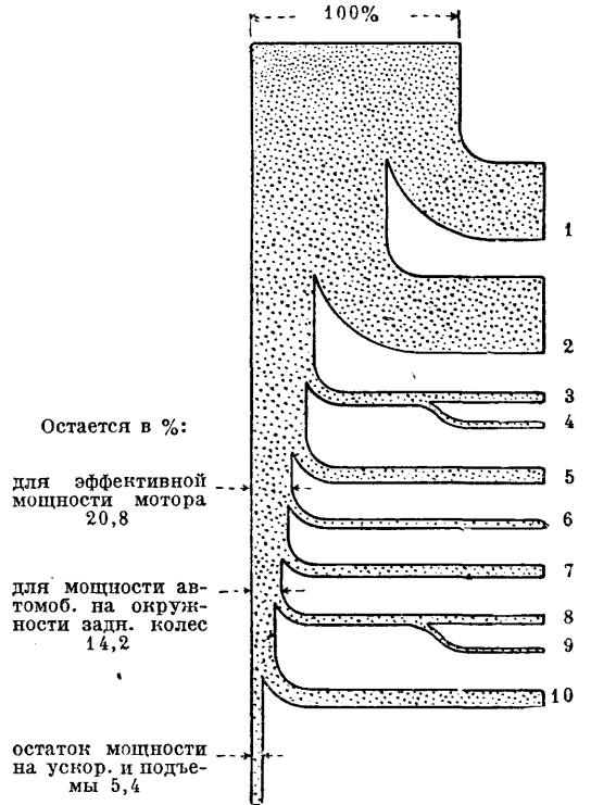
Фиг. 30. Баланс мощности автомобиля (энергия топлива 100%). Потери в %: 1—через охлаждающую воду—35,8; 2—на лучепускание и с отходящими газами—35,6; 3—на сопротивление трубопровода—1,0; 4—через глушитель—1,2; 5—на механические потери в двигателе—5,6; 6—на трение в трансмиссии на прямой передаче—2,9; 7—в задних покрышках—3,7; 8—в передних покрышках—1,1; 9—на сопротивление в перед. колесах—0,6; 10—на сопротив. воздуха—7,1.
