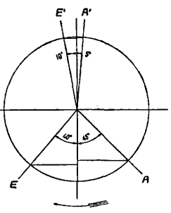
Фиг. 3. Диаграммы распределения мотора: A — начало выпуска, A' — конец выпуска, E' — начало всасывания, E — конец всасывания.
