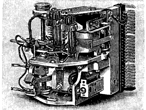
Фиг. 11. Искатель системы Сименс и Гальске. (Вид с передней стороны.)
