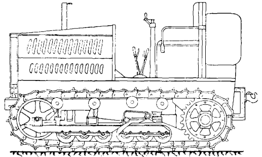
Фиг. 2. Русский 5-т гусеничный трактор Большевик.
