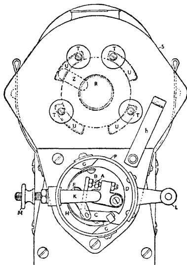
Фиг. 24а. Боковой вид магнето Бош.
