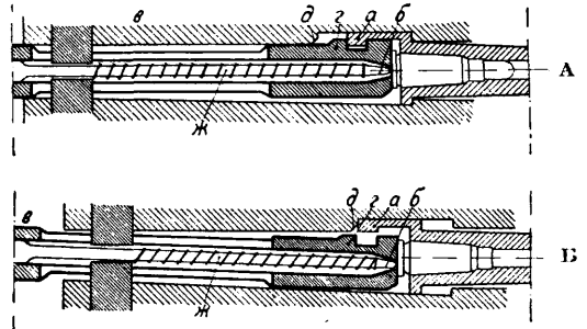
Фиг. 9. Схема автоматического пистолета Бергмана: А—положение при закрытом затворе, Б—положение при начале открывания затвора.
