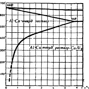
Фиг. 1. Диаграмма состояний двойных сплавов Al-Cu (Dix u. Richardson).
