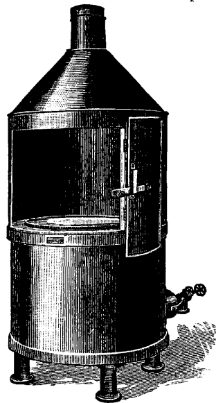
Фиг. 14. Печь системы «Белью» для плавления свинца (газовая или керосиновая).
