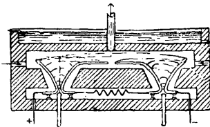
Фиг. 5. Печь Паулинга.
