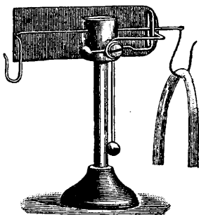
Фиг. 3. Баланс Штауба.
