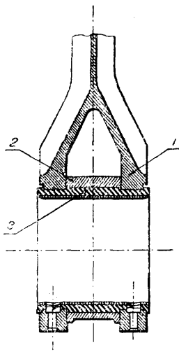
Фиг. 22. Шатунное сочленение: 1 — наружный вильчатый шатун, 2 — внутренний шатун, 3 — вкладыш.
