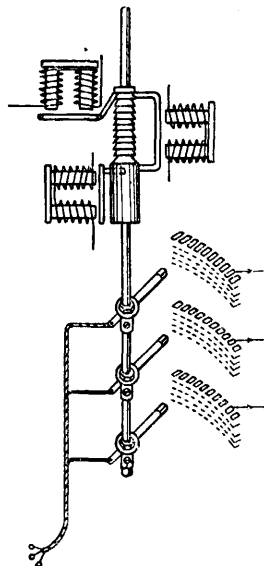
Фиг. 4. Схема установки искателя Струуджера.
