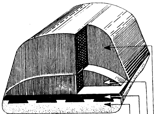
Фиг. 5. Массивная шина: 1 — стальной бандаж, 2 — роговая резина, 3 — полув. резина, 4 — протектор.
