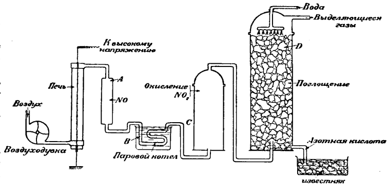
Фиг. 3. Схема производства норвежской селитры.
