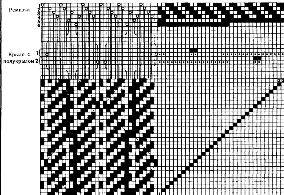
Определение ажурного переплетения.
