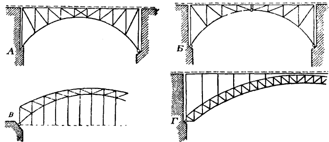
Фиг. 1. Примеры мостовых сквозных арочных ферм: А — двухшарнирная арка с ездой по верху, Б — трехшарнирная арка с ездой по верху, В — двухшарнирная арка с подвешенным мостовым полотном, Г — двухшарнирная арка с ездой по верху, Д — серповидная двухшарнирная арка с ездой по середине.
