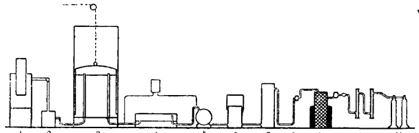
Фиг. 10. Схема расположения стационарной ацетилено-кислородной установки: 1—генератор, 2—газопромыватель, 3—газгольдер, 4—прибор для очистки газа и манометр, 5—газомер, 6—водяной предохранитель, 7—сушилка, 8—фильтр для газа, 9—компрессор, 10—маслоотделитель, 11—бутылки для наполнения.
