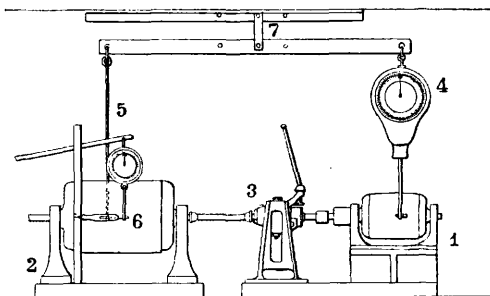
Фиг. 34. Станок для испытания коробки передач: 1—вращающая пендель-динамо, 2—вращаемая динамо, 3—испытываемая коробка передач, 4—динамометр налагаемой нагрузки, 5—динамометр потери нагрузки, 6—указатель, 7—балансирующий рычаг.
