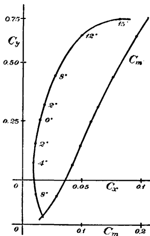
Фиг. 13. Поляра Лилиенталя 1-го рода.
