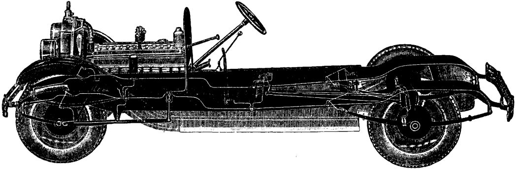
Фиг. 46. Схема центральной смазки шасси.
