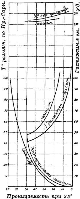
Фиг. 2. Свойства регенерированного асфальта из кисл. отходов от очистки цилиндров и машинного масел.
