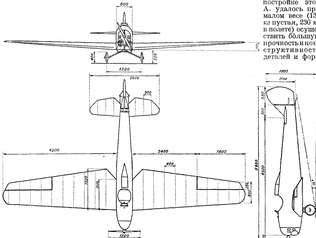
Фиг. 1. Общий вид авиатки «Буревестник С 4», с мотором Блекборн 20 HP, конструкции инженера В. П. Невдачина.
