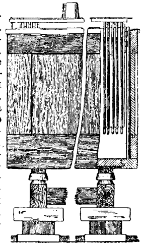
Фиг. 22. Установка стационарного А.
