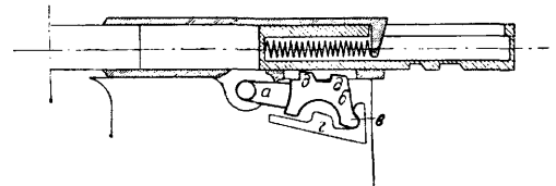
Фиг. 6б. То же.—Положение после выстрела.
