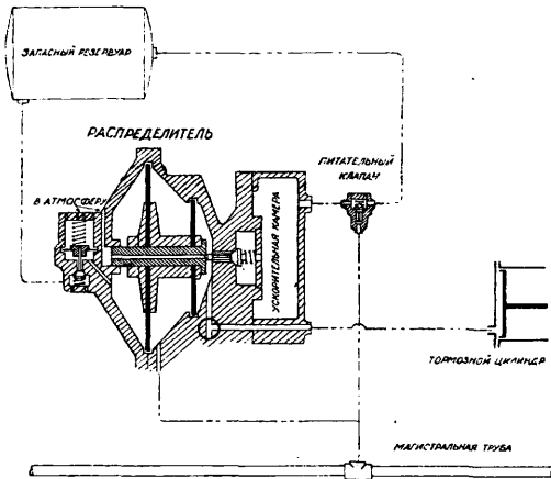
Фиг. 13. Схема однорежимного воздухораспределителя тормоза Казанцева.
