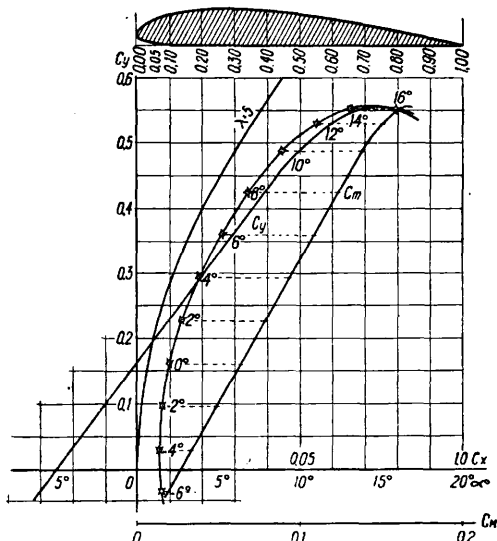
Фиг. 11. Характеристика крыла.
