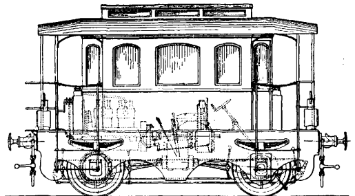
Фиг. 3. Мотовоз системы Матваль.
