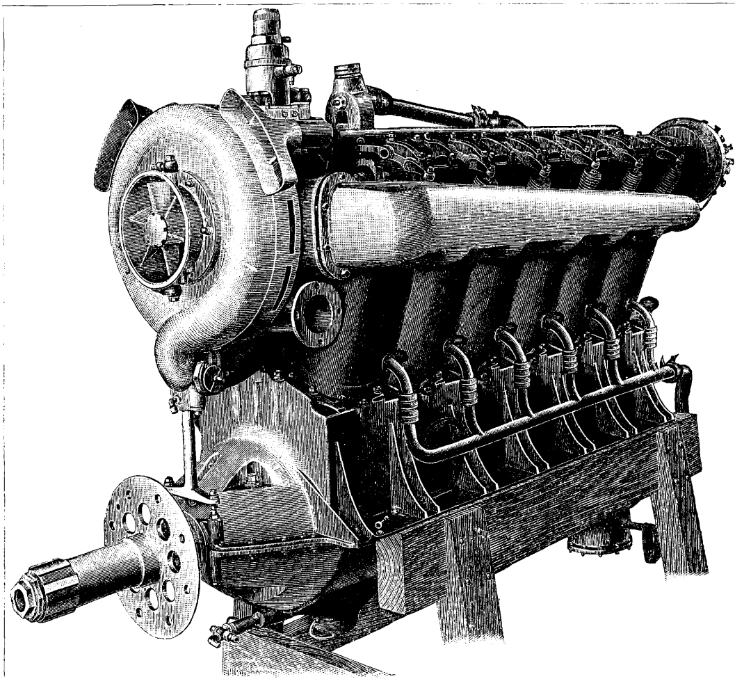
фиг. 33. Установка турбокомпрессора Чербонди на двигателе Либерти 12-А 400 HP.
