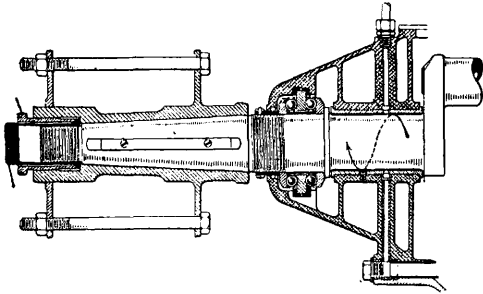
Фиг. 26. Втулка пропеллера двигателя Испано-Суиза 300 Н.
