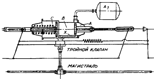
Фиг. 10. Положение тормозных поршней и передачи при отпущае.
