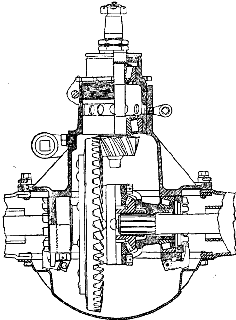
Фиг. 15. Дифференциал с коническими шестернями.
