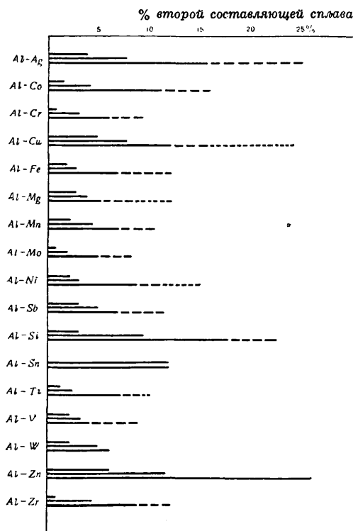
Фиг. 2 Обрабатываемость различных двойных алюминиевых сплавов (Gorson).
