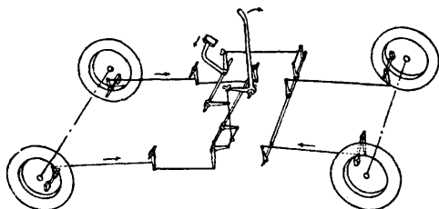
Фиг. 24. Схема привода торможения на четыре колеса.
