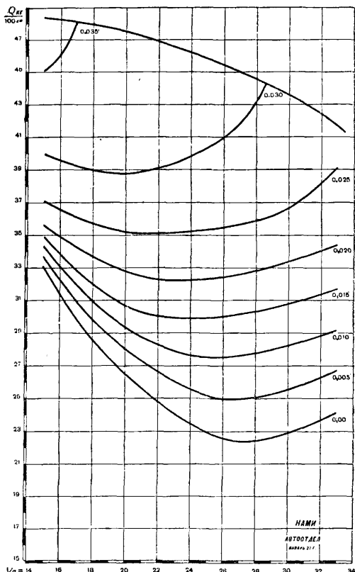
Фиг. 35. Диаграмма экономии автомобиля по испытаниям на станке Ридлера.
