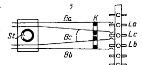
Фиг. 18. Линейный искатель Вестерн.
