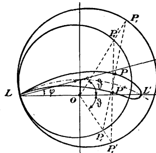
Фиг. 6. Построение инверсии параболы по методу Треффа.
