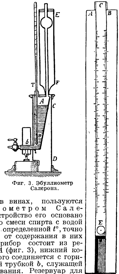
Фиг. 4. Линейка к прибору Салерона.
