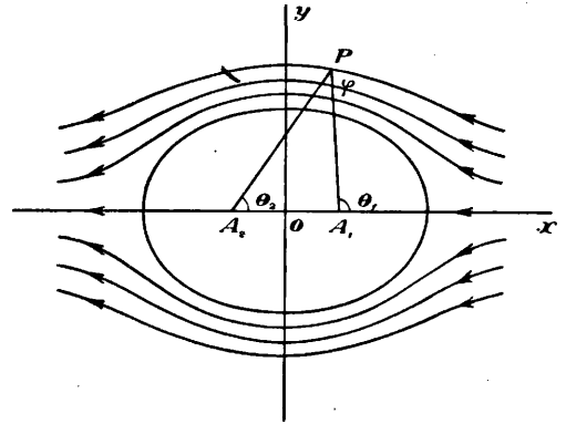
Фиг. 2. Схема источника и стока.
