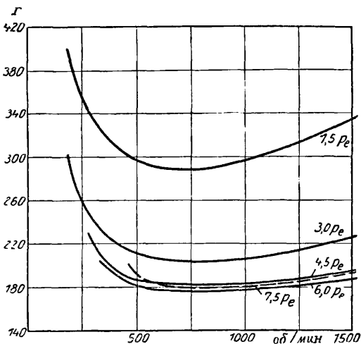
Фиг. 33. Расход топлива двигателя Юнкерс.
