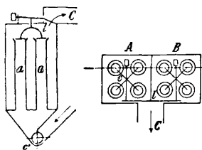
Фиг. 3. Схематический чертеж фильтра Бэта.
