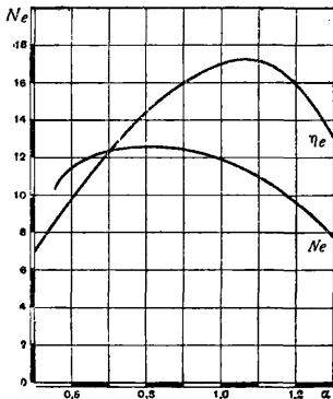
Фиг. 4. Влияние состава рабочей смеси.
