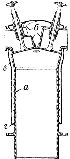
Фиг. 15. Цилиндр двигателя Либерти: а — стальная букса, б — патрубки клапанов, в — рубашка, г — ребра.
