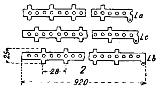
Фиг. 15. Линейный искатель Вестерн.
