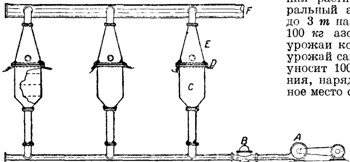
Фиг. 9. Схема «конверторов» Франка-Каро: А—магнетальный насос, В—газорегулятор, С—контактный аппарат, D—платиновая газовая сетка, нагреваемая электричеством, E—алюминиевый шлем с слюдяным глазком, F—выход окислов азота.
