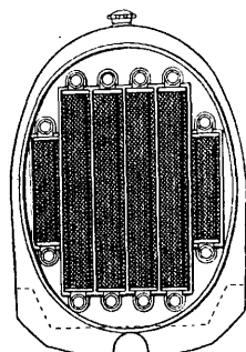
Фиг. 20. Радиатор авт. NAG из отдельных секций.
