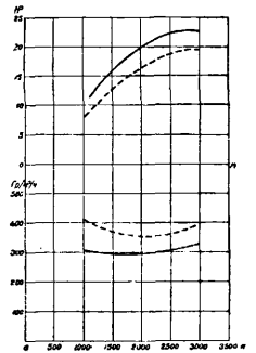
Фиг. 11. Мощность и рас-ход тепла у моторов с чу-гунными (---) и легкими поршнями (—).
