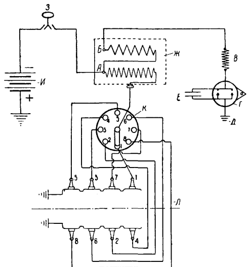
Фиг. 25. Схема зажигания Делько-Кадляк: А—вторичная, В—первичная обмотка, В—постоян. сопротивление (предохранитель), Г—прерыватель с двумя парал. контактами, Д—масса мотора, Е—конденсатор, Ж—индукц. катушка, З—выключатель, И—аккумулятор, К—распределитель.
