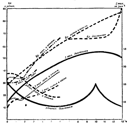
Фиг. 3. Механические качества Al-Mg сплавов (Gorson).
