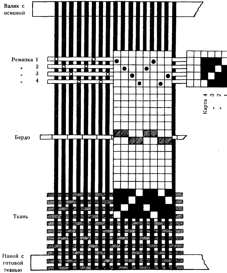
Фиг. 1. Заправка ткани на основании результатов анализа.
