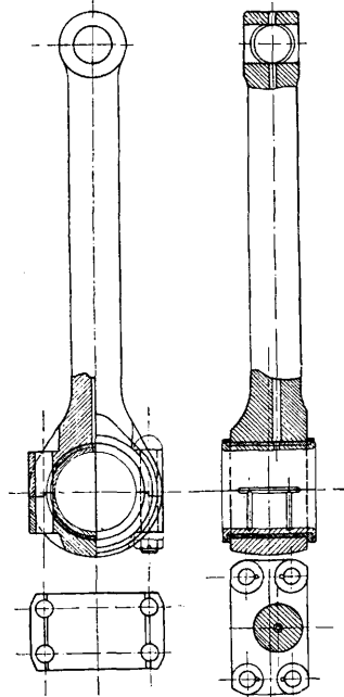
Фиг. 14. Шатун из электрона.
