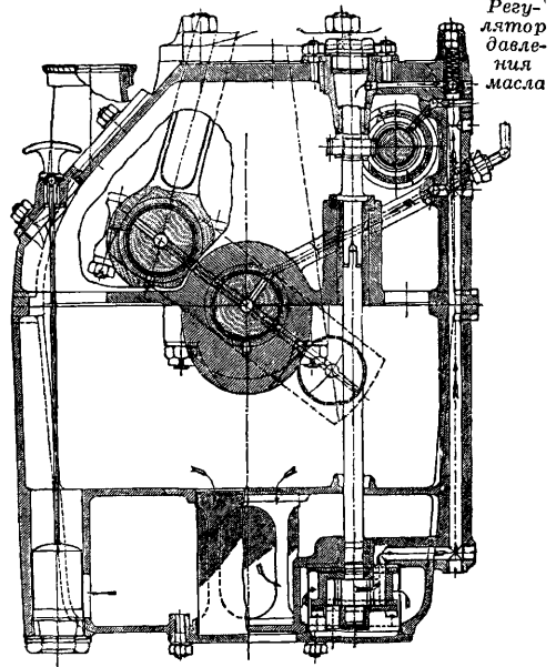
Фиг. 17. Смазка мотора Дикси.
