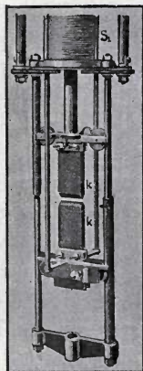
FIG. 27.—PILSEN LAMP.
