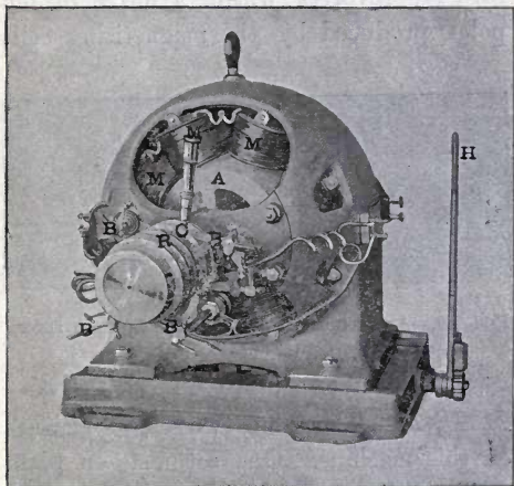
FIG. 149.—30 KILOWATT ALTERNATOR.
