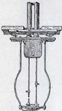
FIG. 32.—BRUSH DOUBLE LAMP.
