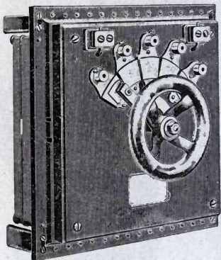
FIG. 119.—PROJECTOR RHEOSTAT.
