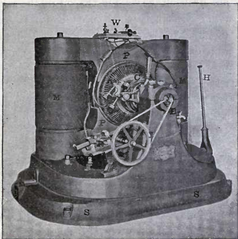
FIG. 139.—SERIES ARC DYNAMO.
