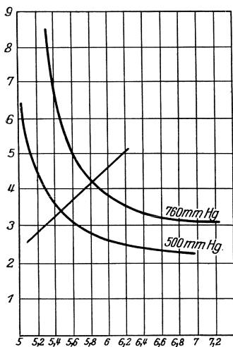
Abb. 29. Gibt nach HASSELBALCH das gegenseitige Verhältnis von Ammoniakzahl und p_{\text{H}} -Wert des Harnes bei verschiedener Sauerstoffspannung. Bei künstlicher Säuerung liegen die Punkte weit rechts oben; lebt ein Mensch bei niedrigem Atmosphärendruck, so kommt es wahrscheinlich zu einer „Alkalose“; bei solchen Menschen liegen die Schnittpunkte links unten.
