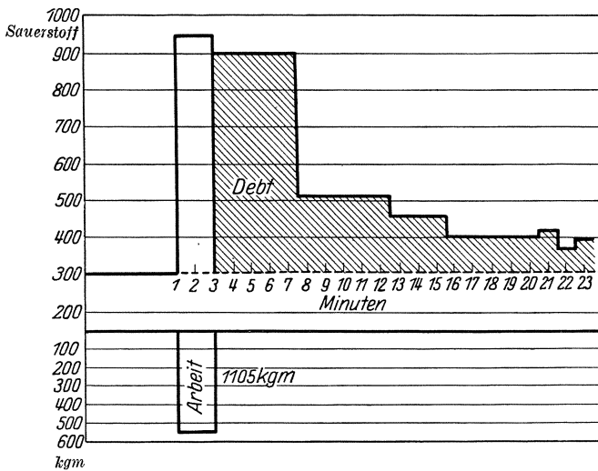
Abb. 24. Herzfehler (A). Requirement: 6110 ccm O 2 . Debt: 4830 ccm Q 2 = 79%.
