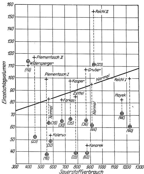
Abb. 15. Verhalten des Einzel Schlagvolumens bei der Arbeit des Herzfehlers.
