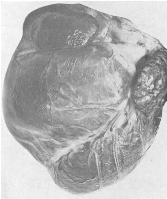
Abb. 53. Dilatation des Herzens, besonders des rechten Abschnittes eines Hundes, der auf der Höhe der \text{CO}_2 -Intoxikation durch Herausschneiden des Herzens akut getötet wurde.
