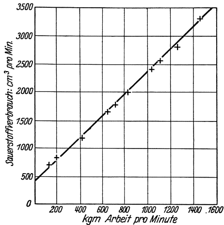
Abb. 3. Sauerstoffverbrauch während der Arbeit des normalen Menschen. Arbeitsleistung in Kilogramm-meter pro Minute. Nach BAINBRIDGE, II. Aufl., S. 25.
