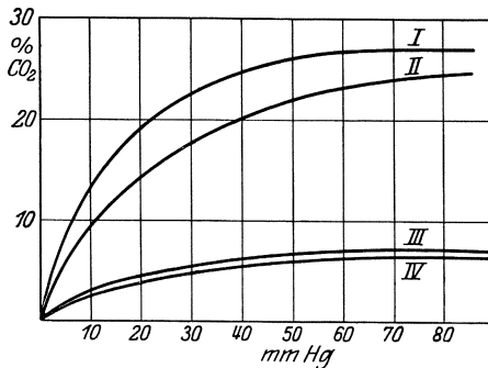
Abb. 39. Kohlensäurebindungskurven von Eiweißlösungen.
