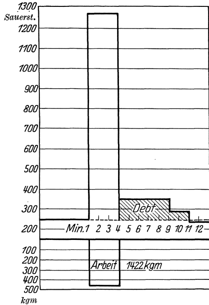
Abb. 22. Normal hell (H. E.). Requirement: 3611 ccm O 2 . Debt: 546 ccm = 15,1%.
