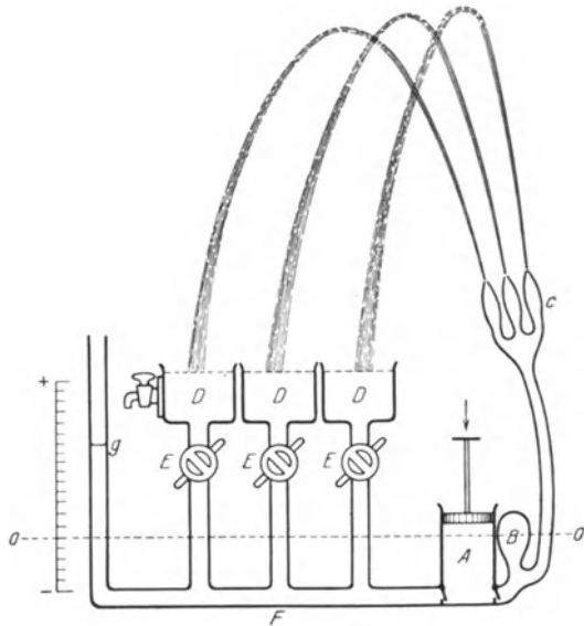
Abb. 1. (Americ. journ. of physiol. Bd. 46, S. 533. 1918.) Kreislaufschema nach HENDERSON: A = Herzpumpe, B = elastische Kammer (Aorta), C = feine Öffnungen (Arteriolen), die sich unter dem Einflusse des Vasomotorensystems bald erweitern, bald verringern. Das Blut, das hier herausspritzt, fängt sich in den Reservoiren D, die das Capillarsystem der Gewebe und Organe repräsentieren. Unter den Reservoiren sind Hähne (E), welche bald mehr, bald weniger geöffnet, den Druck im venösen System (F) erhöhen resp. den Zufluß zum Herzen steigern. Sind die Hähne (E) ganz offen, so ist der Druck im venösen System am höchsten; G steigt fast bis zum Niveau in den Reservoiren D. Sind die Hähne dagegen zum Teil geschlossen, so sinkt G, während sich die Behälter (D) füllen. Die Linie \theta-\theta soll zum Ausdruck bringen, daß sich die Herzpumpe, eingeschlossen im Thorax, unter einem negativen Druck befindet.
