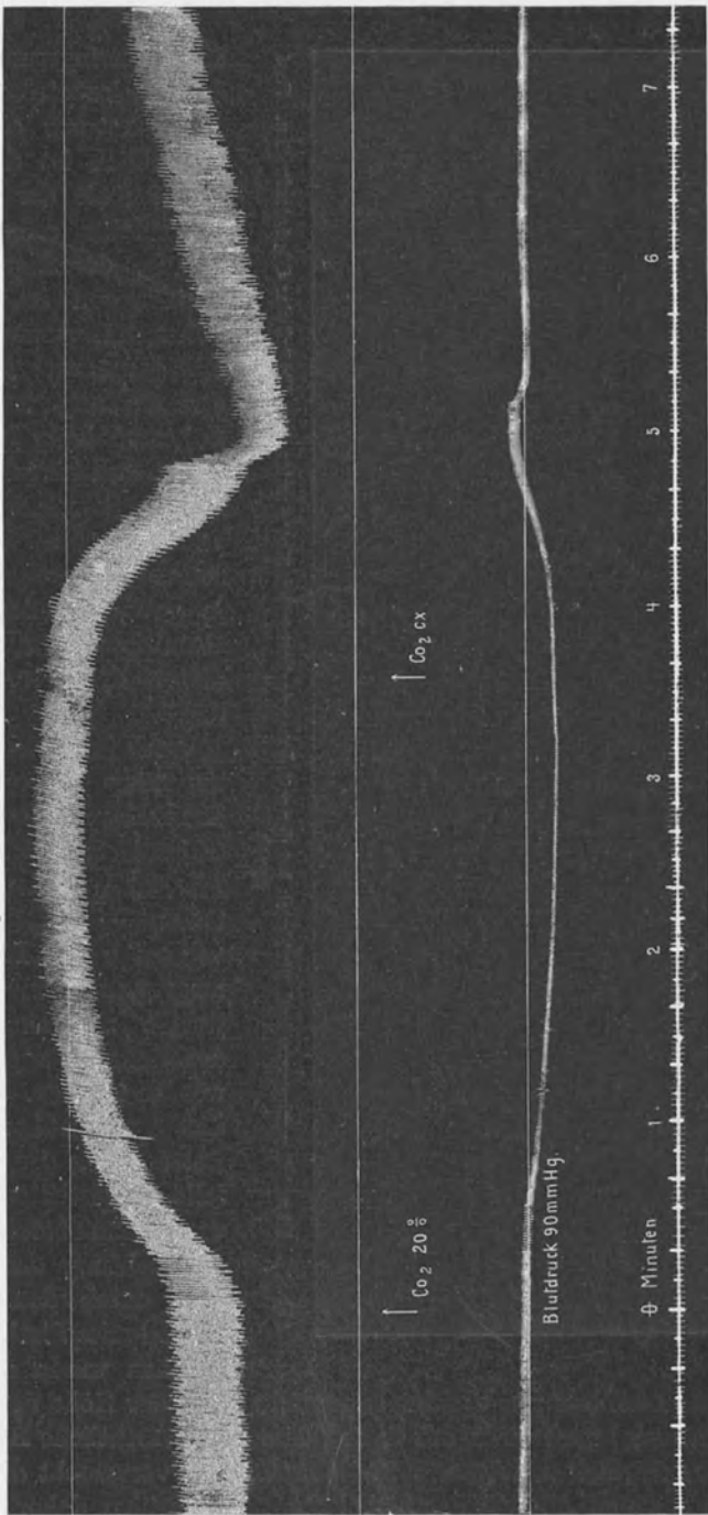
Abb. 47. Einfluß der \text{CO}_2 -Intoxikation auf Plethysmogramm des Herzens und dem Blutdruck einer narkotisierten Katze.
