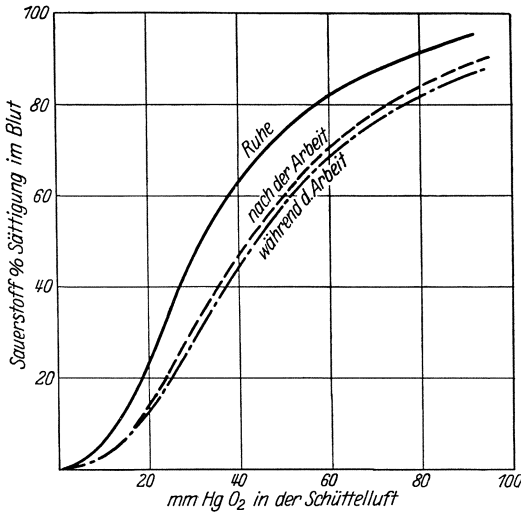
Abb. 36. Nicht inkompensiertes Mitralvitium. Arbeitsleistung 250 kgm pro Min. bei 3 Minuten Gesamtdauer. Die Kurve ist bei 44 mm Hg CO 2 konstruiert.
