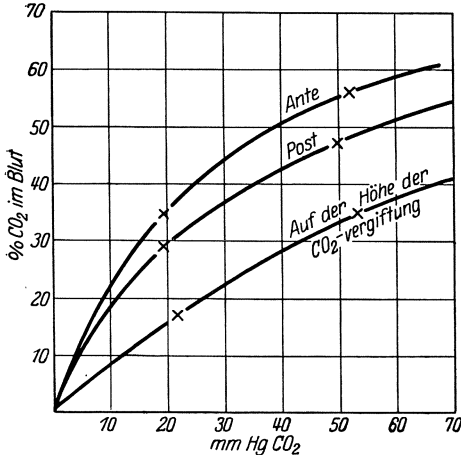
Abb. 41. Kohlensäurespannungskurve im arteriellen Blute vor, während und nach der Kohlensäurevergiftung. Inspirationsluft: 20% \text{CO}_2 und 30% \text{O}_2 ; Dauer 20 Minuten.
