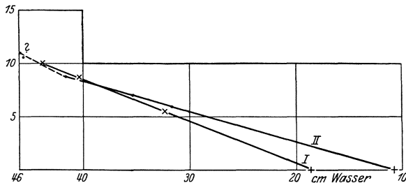
Abb. 43. Kolloidosmotischer Druck im arteriellen Blut vor und während der Kohlensäureatmung. I. Graphisch 18,6, rechnerisch 19,0 cm 2 Wasser. II. Graphisch 10,8, rechnerisch 10,5 cm 2 Wasser.
