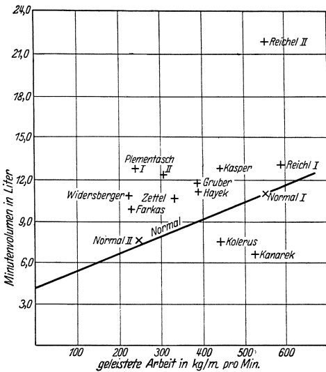
Abb. 11. Gegenseitiges Verhalten von Minutenvolumen und Arbeitsleistung beim Herzfehler.
