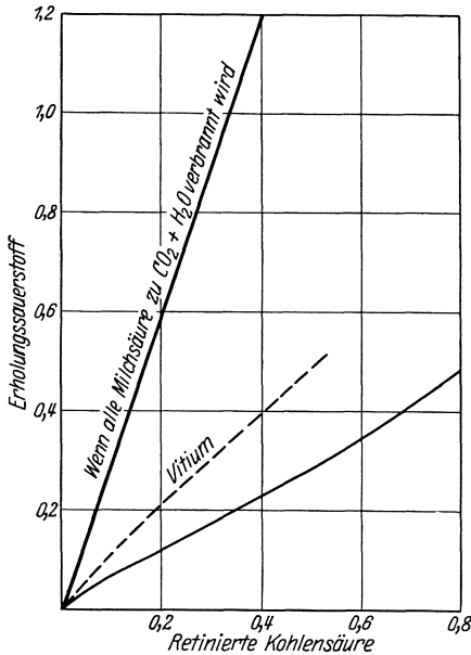
Abb. 28. Gegenseitiges Verhalten von retinierter CO 2 und Erholungssauerstoff; die punktierte Linie entspricht dem Verhalten eines inkompensierten Vitiums.
