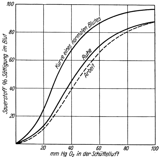
Abb. 35. Inkompensierte Mitralklappenstenose; Arbeitsleistung 200 kgm pro Min. bei 3 Minuten Gesamtdauer. Oben Kurve eines gesunden Menschen mit gleichem Hämoglobingehalt. Alle 3 Kurven bei 40 mm Hg CO 2 konstriert.
