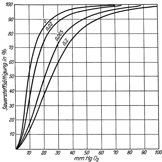
Abb. 37. Sauerstoffdissoziationskurve nach Zusatz von 0,0, 0,02, 0,065 und 0,2% Milchsäure. Nach BARCROFT.
