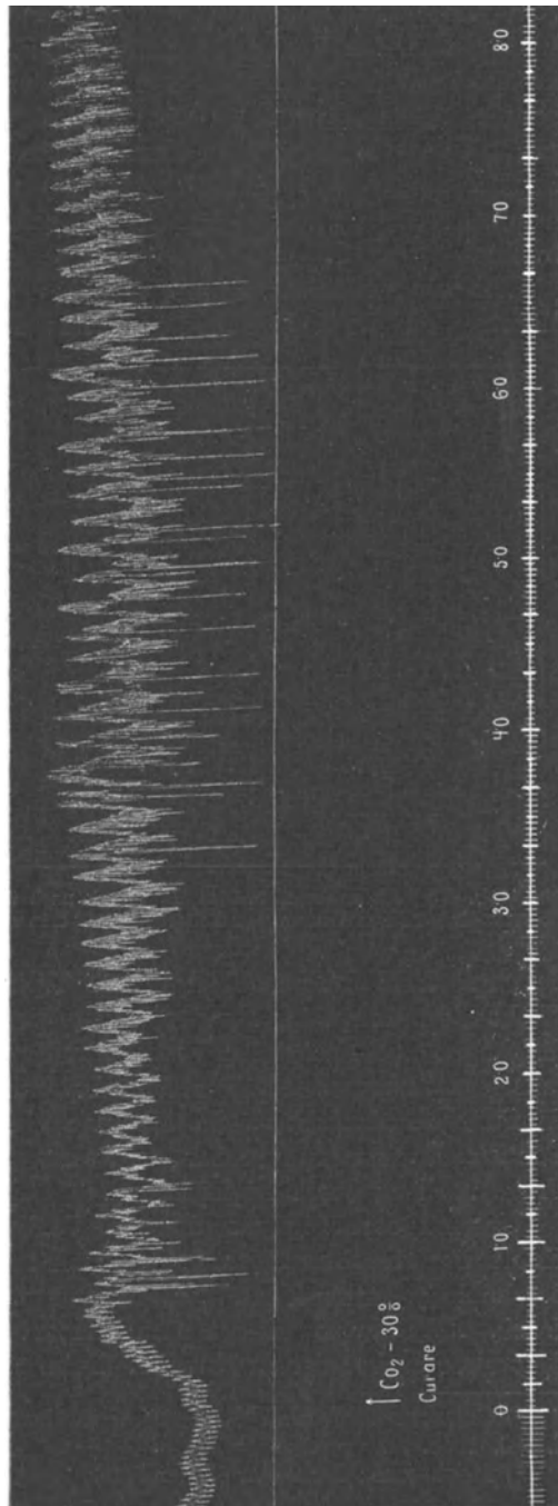
Abb. 44 a. Blutdruckkurve bei einem Hund unter dem Einfluß von Kohlensäureatmung. Curare.
