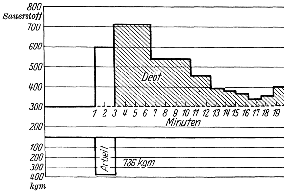
Abb. 25. Herzfehler (B). Requirement: 3894 ccm O 2 . Debt: 3297 ccm O 2 = 84%.
