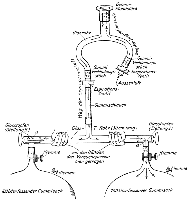
Abb. 21. Die von uns gewählte Versuchsordnung zwecks Feststellung des Requirements und Debts.
