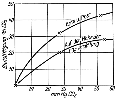
Abb. 42. Kohlensäurespannungskurve im arteriellen Blute vor, während und nach der Kohlensäurevergiftung. Inspirationsluft: 30% \text{CO}_2 und 30% \text{O}_2 ; Dauer 15 Minuten.
