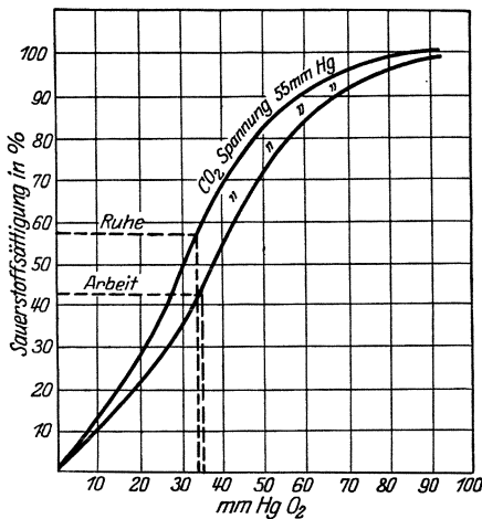
Abb. 9. Sauerstoffspannung in mmHg.
