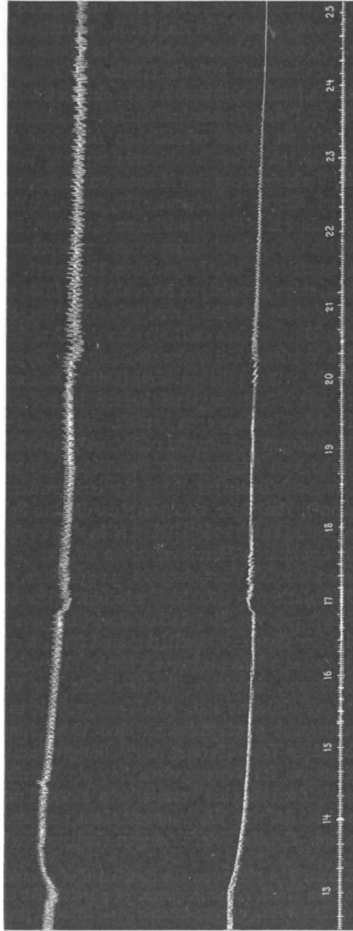
Abb. 54 b. Fortsetzung der Abb. 54 a. Weiteres Absinken des Blutdruckes; das Herz schlägt vollkommen arrhythmisch.
