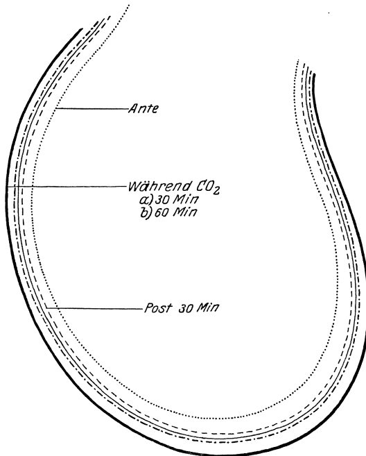
Abb. 52. Orthodiagramm des Hundeherzens, vor, während und nach der CO 2 -Vergiftung.
