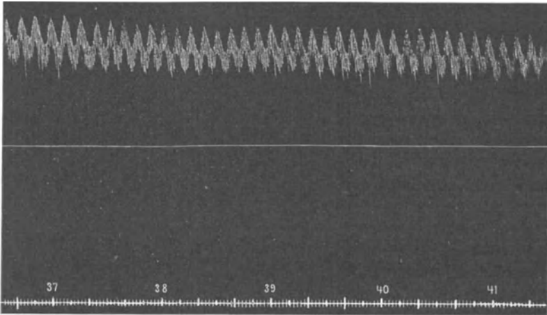
Abb. 44b. Fortsetzung der Abb. 44a. Blutdruck nach wie vor hoch; starke Entwicklung von HERING-TAUBESchen Wellen. Die Zeitangabe läßt erkennen, wie lang die CO 2 -Atmung währt.
