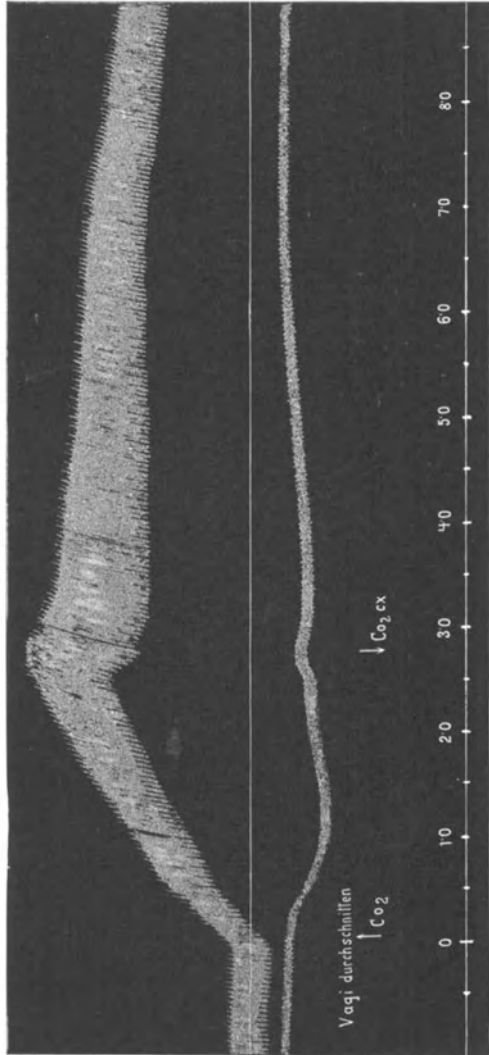
Abb. 49. Fortsetzung der Abb. 48. Nach Rückkehr zu den ursprünglichen Werten werden die Vagi durchschnitten und neuerdings der Einfluß der CO 2 -Intoxikation studiert; wiederum 15% CO 2 .
