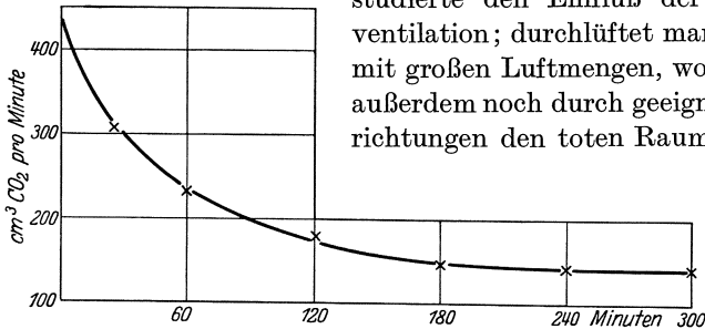
Abb. 40. Graphische Darstellung der innerhalb von 5 Stunden durch Hyperventilation abgegebenen Kohlensäure. Hund 21 kg (Chloralose Narkose). Ruhewert: 132 cm³ CO₂ pro Min.; Atemvolumen 4,023 l pro Min. = 39,6 l CO₂ in 5 Stunden. Tatsächliche Abgabe während der Hyperventilation: 49—50 l Atemvolumen, innerhalb 5 Stunden 53,3 CO₂.
