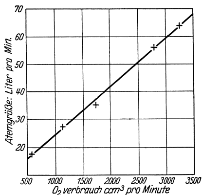
Abb. 6. Atemgröße bei der Arbeit normaler Menschen.
