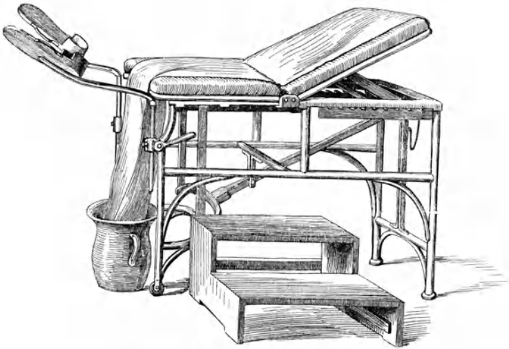
Abb. 3. Untersuchungsstuhl.
