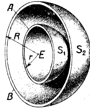
Рис. 3. Два концентрических шара, в центре которых находится электрический заряд.
