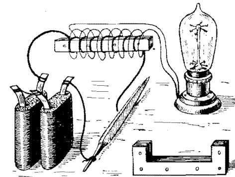
Рис. 44. Каждый раз, как проводочка соскакивала с зубринки напильника, нить лампочки накалялась.
