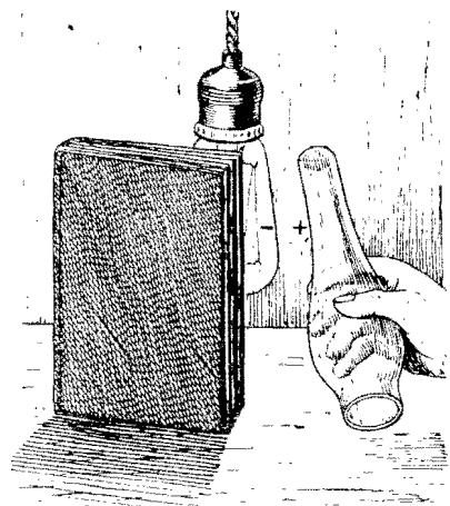
Рис. 7. Я отодвигаю ламповое стекло — и волосок калильной лампочки сильно выгибается.
