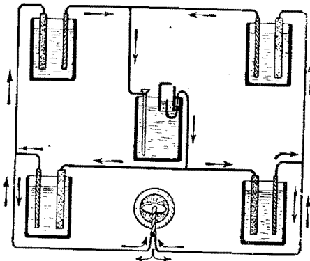
Рис. 29. Соединение четырех выпрямителей, дающее возможность использовать полностью переменный ток.
