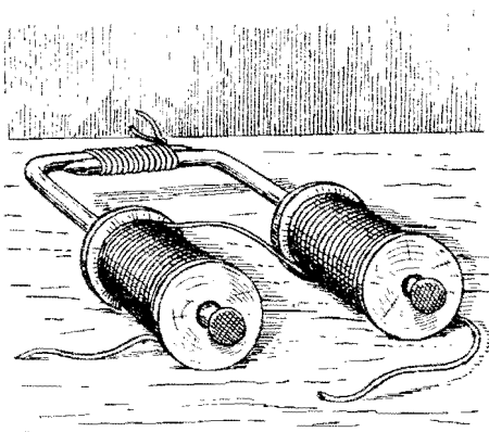
Рис. 38. Электромагнит из двух катушек из-под ниток и двух толстых гвоздей.
