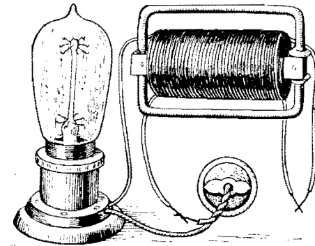
Рис. 47. Если на сердечник катушки наложить два согнутых гвоздя, то свет лампочки сильно ослабевает.
