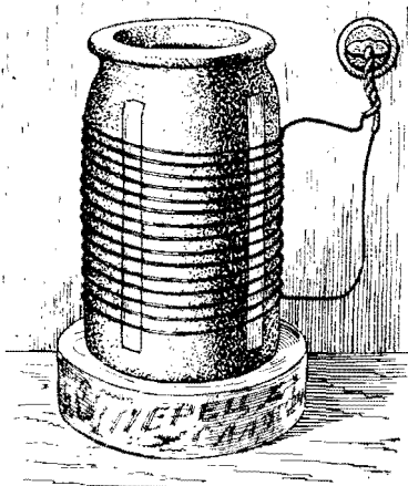
Рис. 31. Новый тип кипятивника. На банку было намотано около 50 витков железной проволоки.
