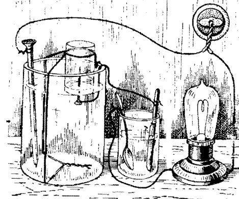
Рис. 28. Наш кулонометр. Объем стакана мы узнали следующим образом: измерили клеенчатым метром его высоту и длину окружности. Как известно, объем цилиндра равен \pi r^2 h .
