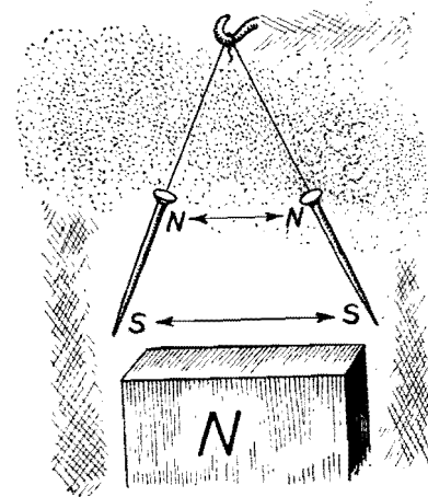
Рис. 36. На нижних концах обоих гвоздей возникают благодаря индукции южные полюса, а на верхних — северные. Так как одноименные полюсы отталкиваются то и гвоздики должны оттолкнуться друг от друга.
