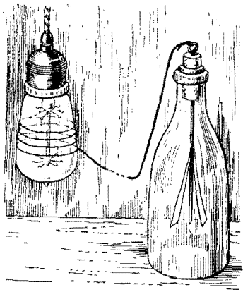
Рис. 8. Если включить электрическую лампочку в сеть, то электроскоп разрядится.
