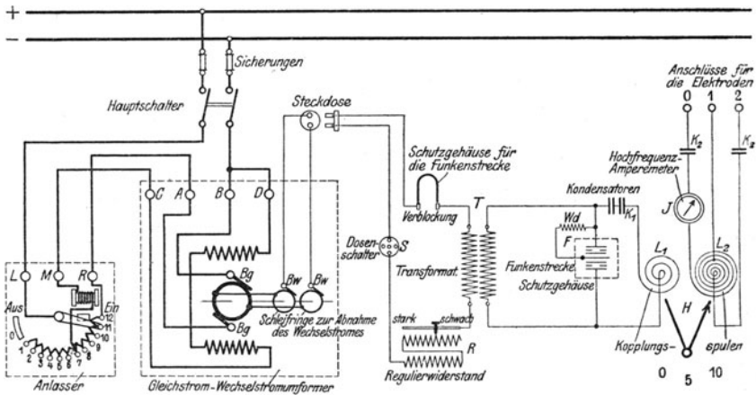
Abb. 17. Siemens'scher Diathermieapparat nach Nagelschmidt. Schaltungsschema.
