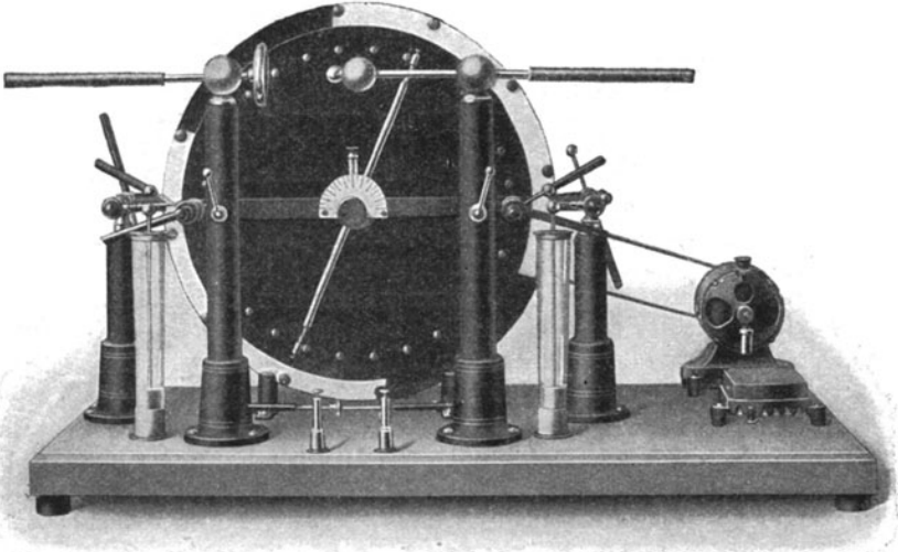
Abb. 1. Influenzmaschine.
