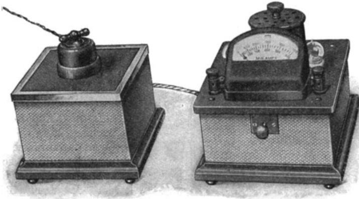
Abb. 27 b. Mikrotherm von Reiniger, Gebbert & Schall.
