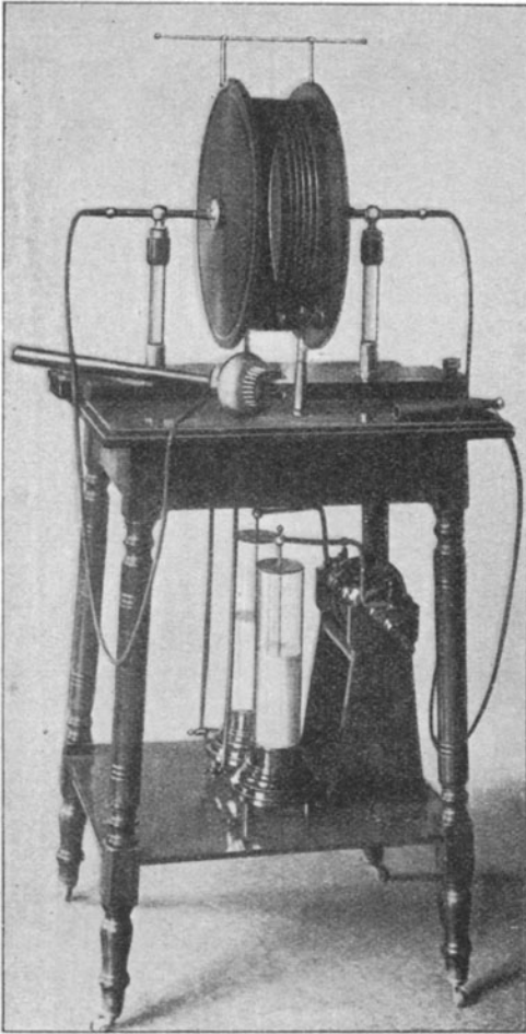
Abb. 12. Sanitas D'Arsonvalapparat.
