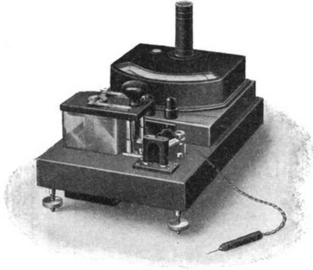
Abb. 62. Temperaturfernmeß- und Registrierapparat von Siemens mit Thermo-Nadel.
