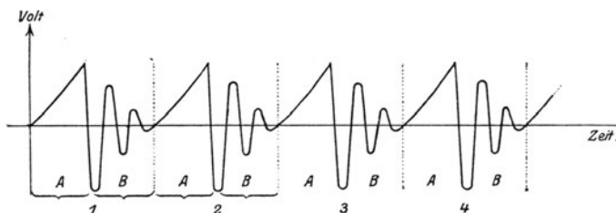
Abb. 20. Spannungsverlauf am Kondensator während einer positiven Phase des primären Wechselstromes. A Ladepériode. B Schwingungsperiode.
