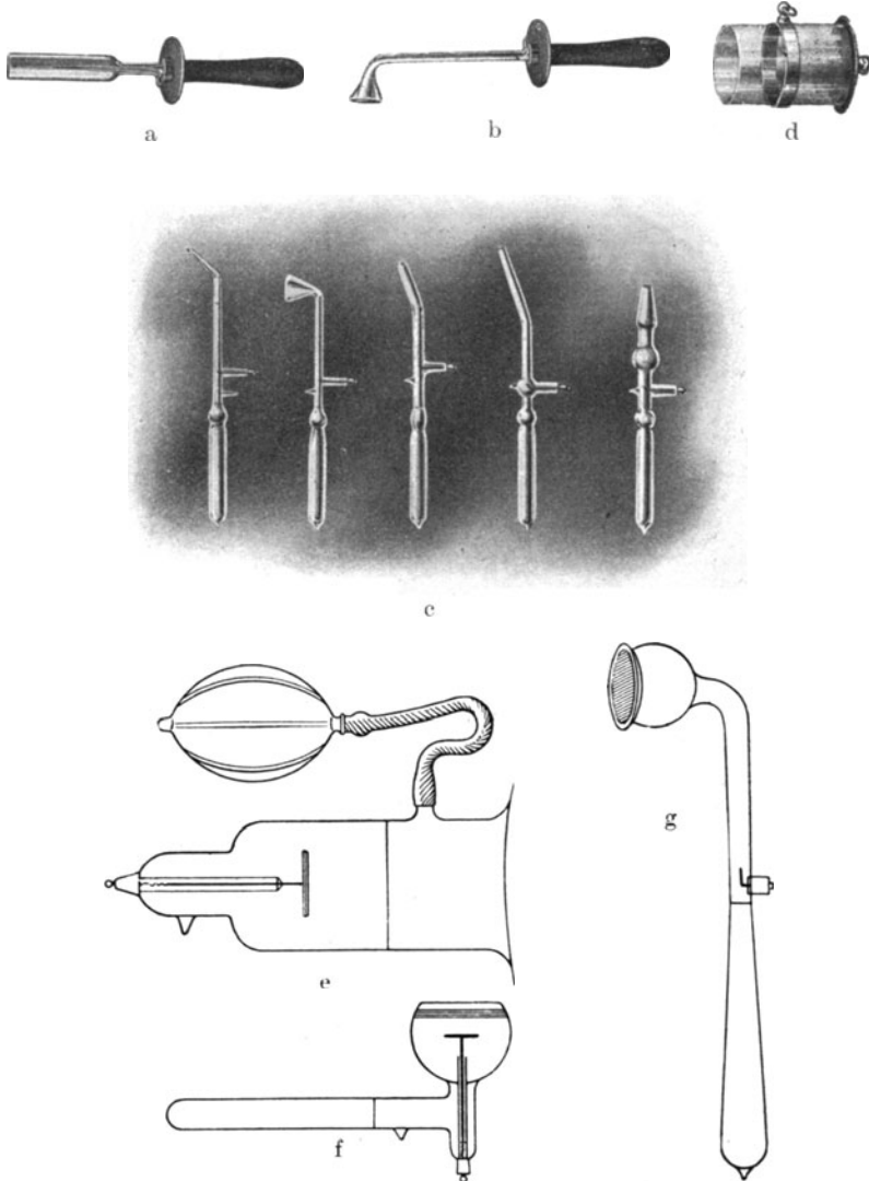
Abb. 32a—g. Kondensatorelektroden verschiedener Form.
