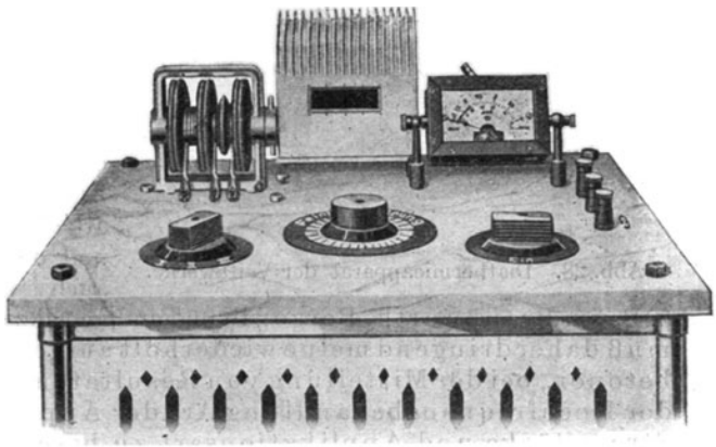
Abb. 27 c. Diathermieapparat der Medizinisch-Technischen Company.
