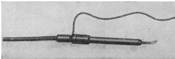
Abb. 65. Chirurgische Metallelektrode, als Thermometer ausgebildet, zur Messung der Temperatur im koagulierten Gewebe.
