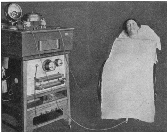
Abb. 31. Kondensatorbett nach Nagelschmidt.
