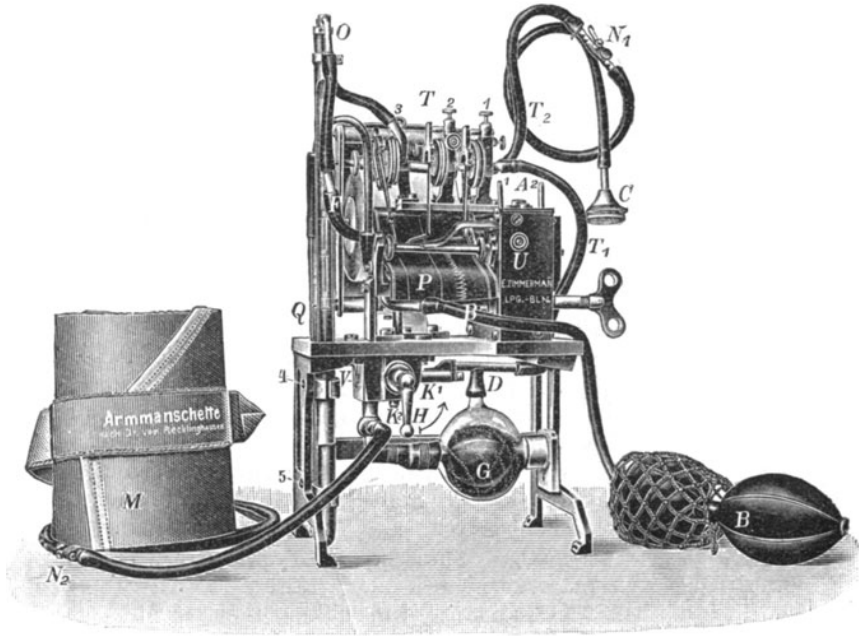
Abb. 78. Sphygmotograph von Uskoff. (Zimmermann, Leipzig.)
