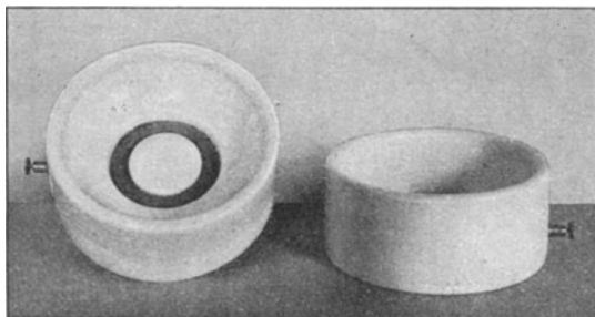
Abb. 38. Kleine Polyfrequenz-Wasserelektroden nach Nagelschmidt.
