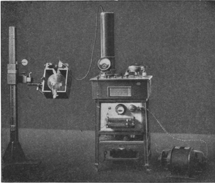
Abb. 23. Äußere Ansicht des Polyfrequenz-Diathermie- und Röntgenapparates.
