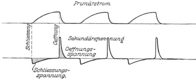
Abb. 2. Stromkurve eines Siemensschen Induktors.
