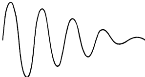
Abb. 3. Lauter Schall.
