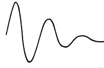
Abb. 6. Kurzdauernder Schall.
