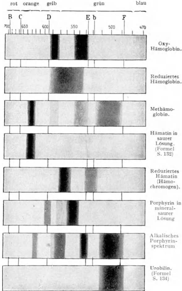
Abb. 59. Spektraltafel.
