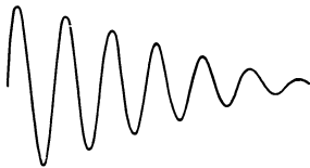
Abb. 7. Hoher Schall.
