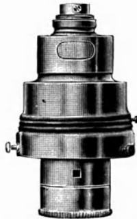
Nippelreduktor 16 Watt. Preis M. 9.50 brutto. \frac{1}{3} nat. Gr.
