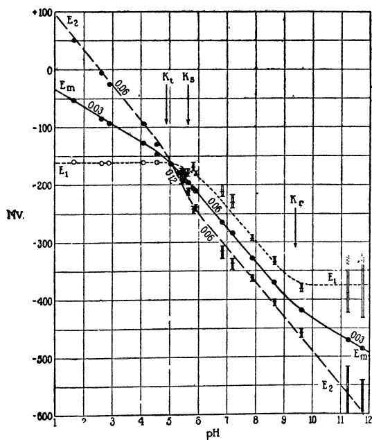
Fig. 14. E/ph-Diagram of pyocyanine acc. to MICHAELIS 808).
