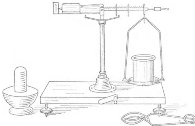
Perplex-Apparat.
