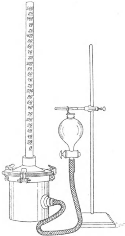
Brotvolumenmesser nach Neumann und Salecker.
