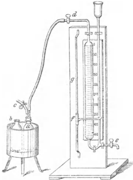
Apparat zur Ermittlung der Gärkraft nach Hayduck.
