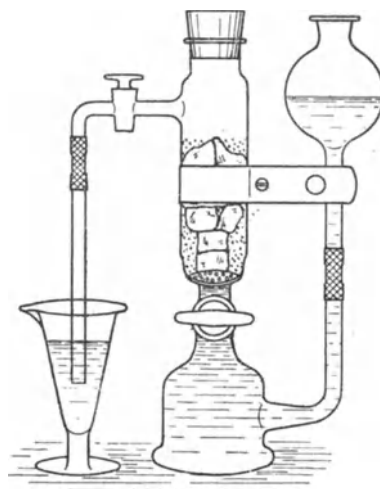
Chlorentwicklungsapparat nach H. Huss.
