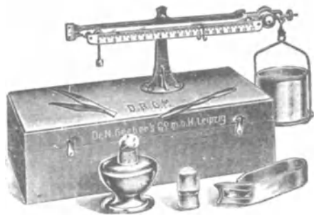
Wage „Superior“
