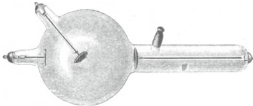
Einfache Röntgenröhre ohne Regeneriervorrichtung.
