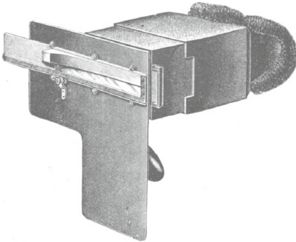
Kryptoradiometer nach Wehnelt.
