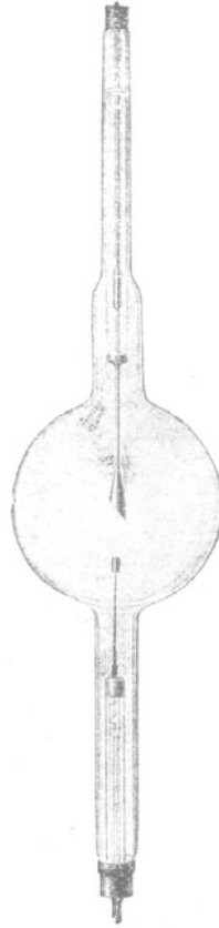
Coolidge-Röhre.
