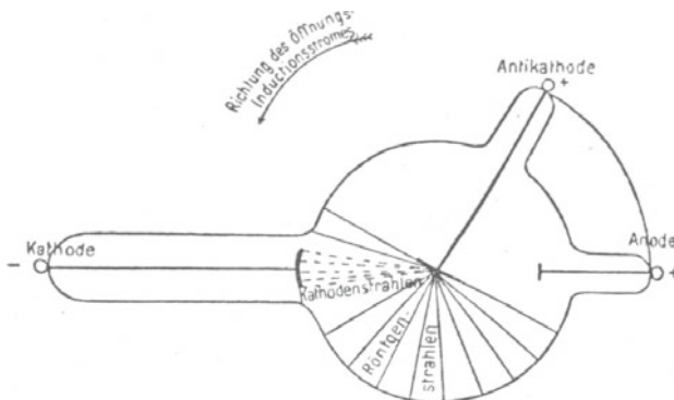
Schema einer Röntgenröhre.
