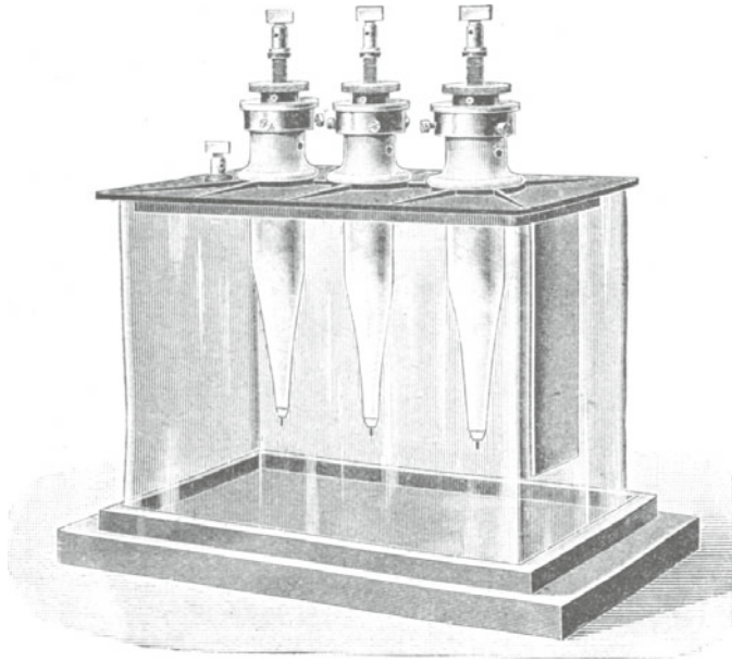
Dreiteiliger Wehnelt-Unterbrecher.
