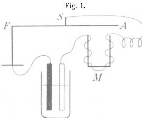
Wagnerscher Hammer.
