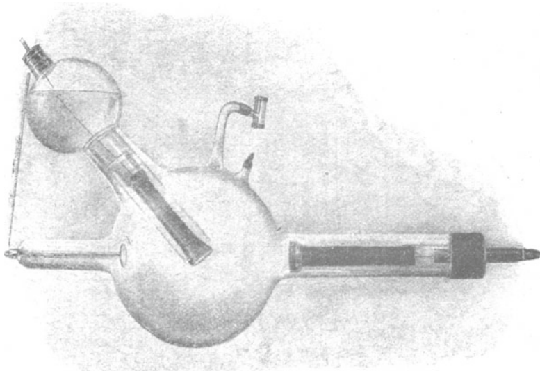
Müllersche Siederöhre.
