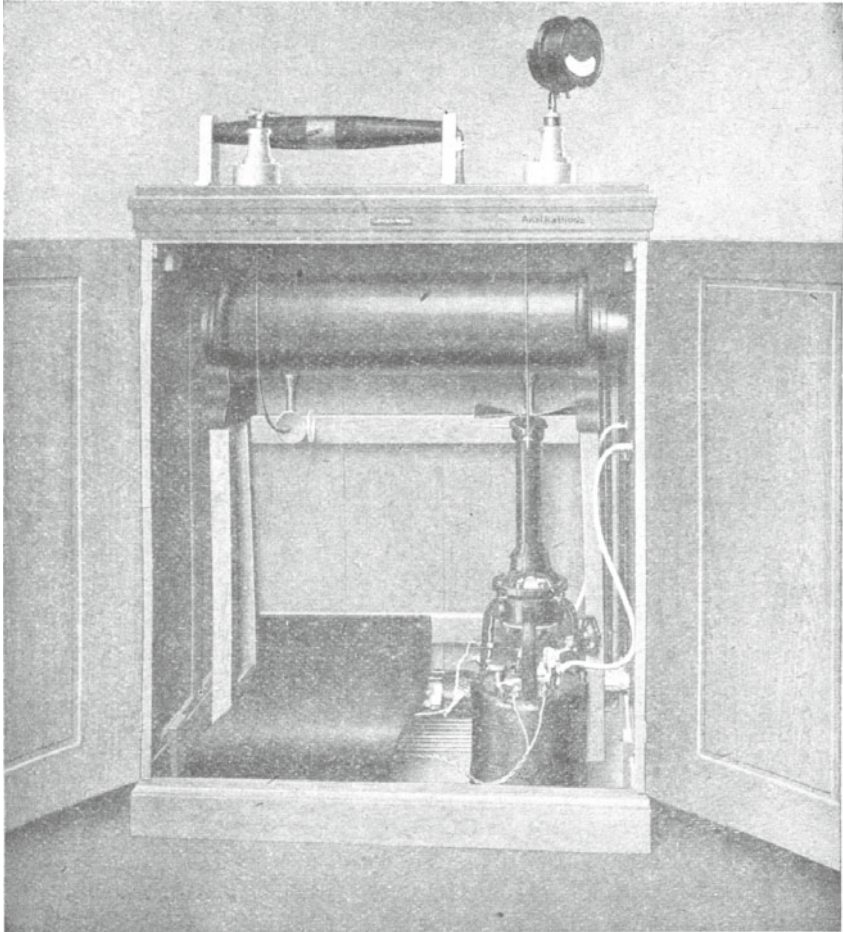
Coolidge-Instrumentarium von Siemens &amp; Halske.
