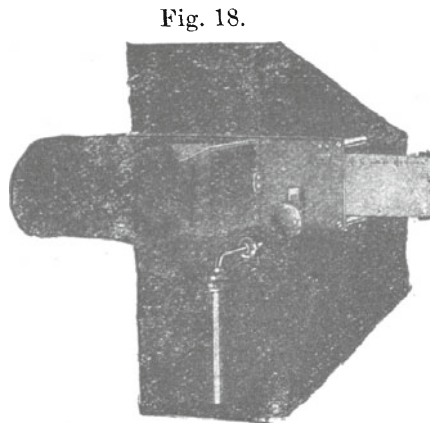
Absoluter Härtemesser nach Christen.
