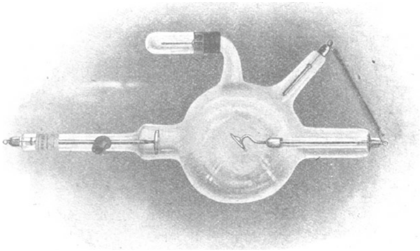
Kleine Therapie-Röhre (Burger).
