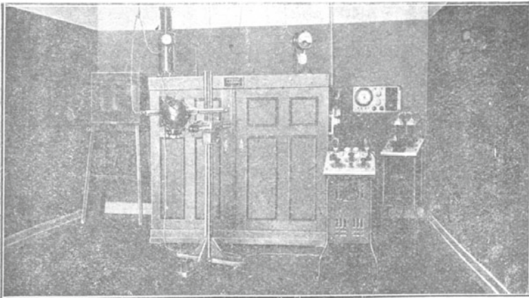
Intensiv-Reformapparat der Veifa-Werke.
