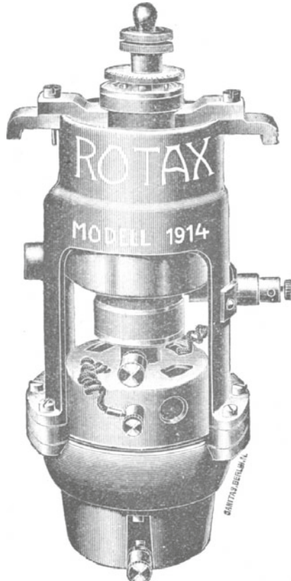
Rotax-Unterbrecher der Elektrizitäts-Gesellschaft „Sanitas“
