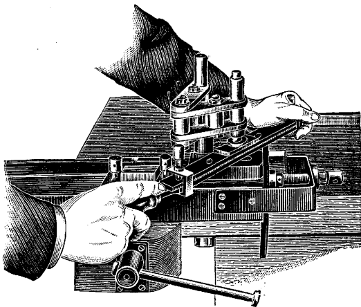
Рис. 8. Опиловочный аппарат.
