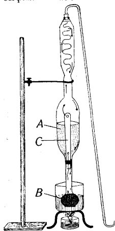
Рис. 1. Аппарат Сокслета.
