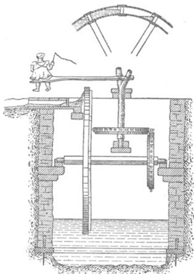
Fig. 5d. Saſie in Unter-Ägypten.
