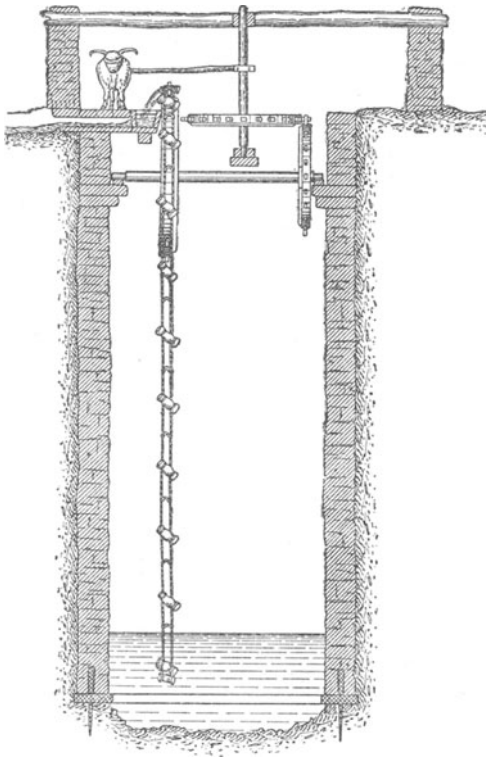
Fig. 5c. Sakie in Ober-Ägypten.
