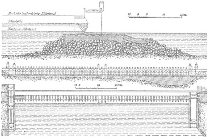
Stauwerk des Rosetta-Nilarms.
