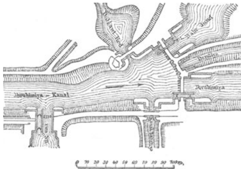
Fig. 12. Regulator bei Derut (W).
