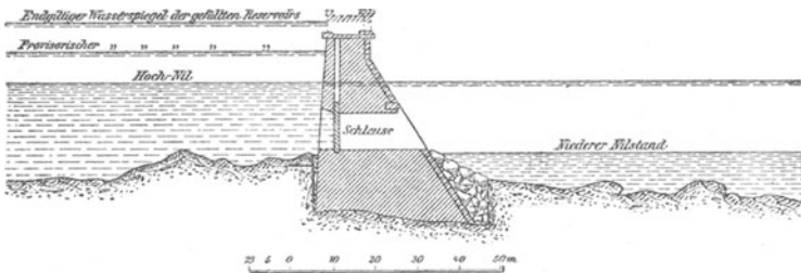
Fig. 15. Querschnitt des Staudamms.
