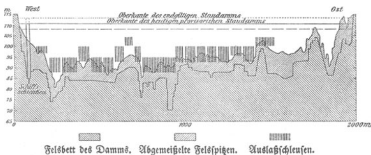
Fig. 16. Querschnitt durch das Nilbett, entlang dem Staudamm.
