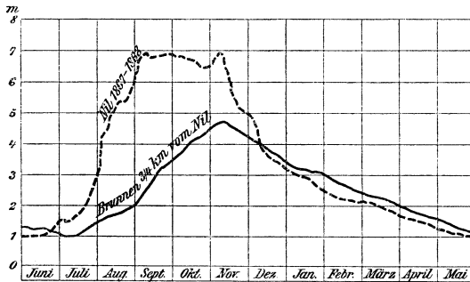
Fig. 3b. Wasserstand des Nils und Niltalbrunnen.
