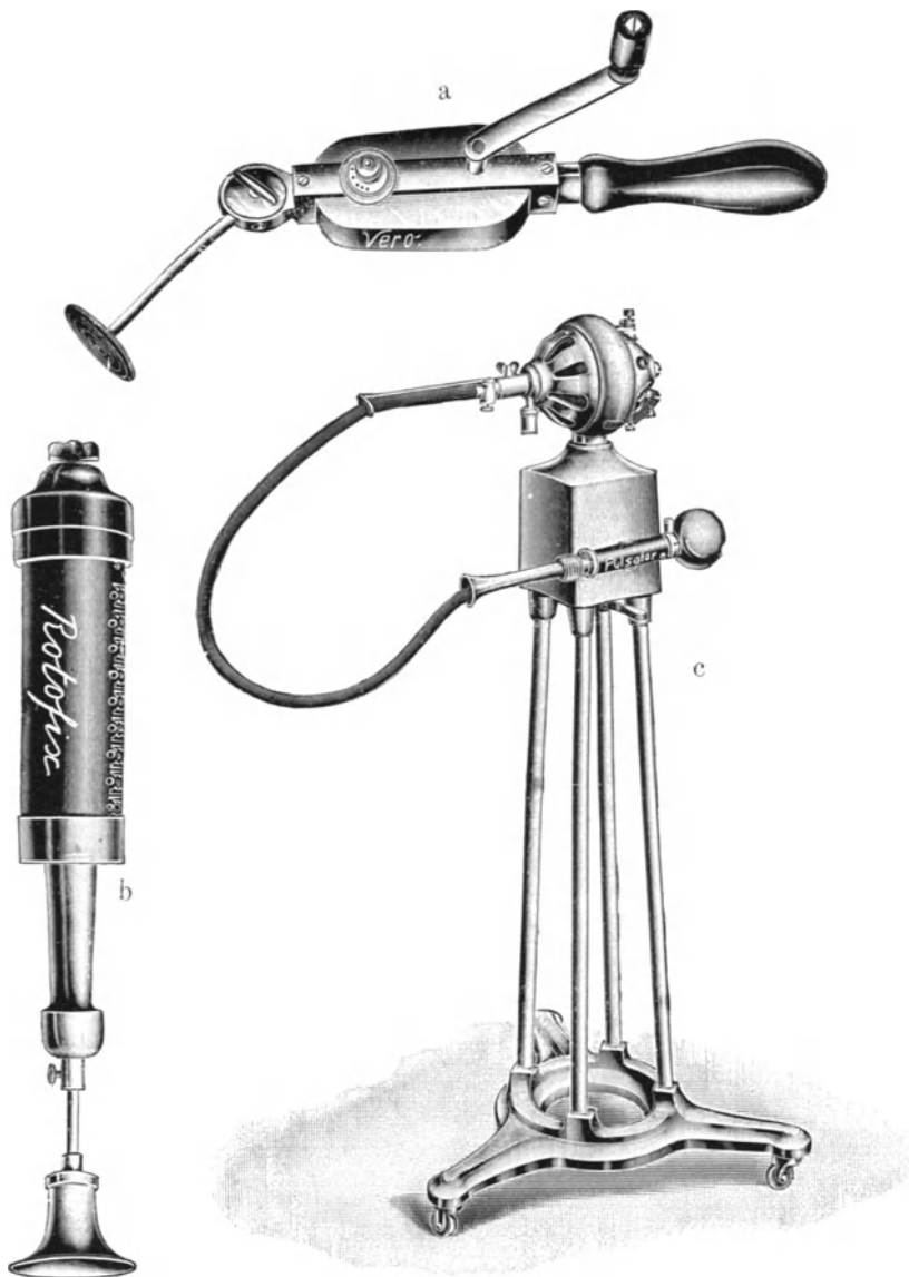
Abb. 54. Vibratoren. a Handbetrieb, b und c elektr. Betrieb.
