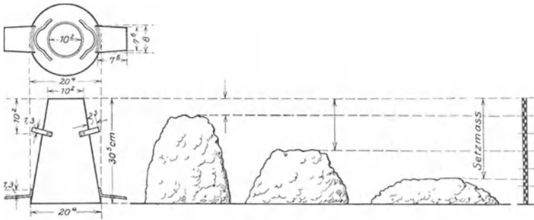
Abb. 1a. Setzprobe.
