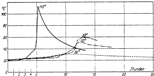
Abb. 3. Abbindetemperaturen.
