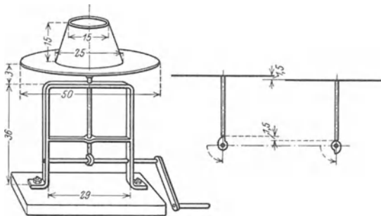
Abb. 1b. Der Fließtisch.
