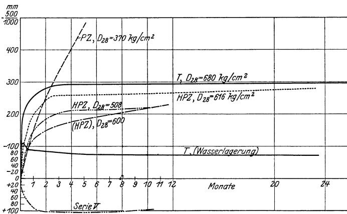
Abb. 7. Volumenänderungen von Beton.
