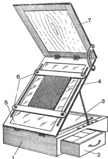
Рис. 40. Ретушевальный станок
