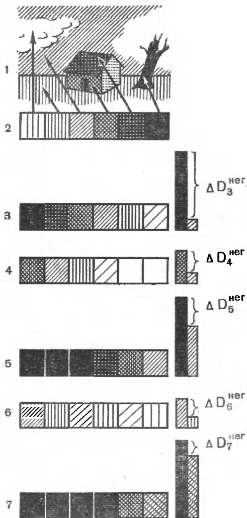
Рис. 20. Схема, поясняющая сущность интервала оптических плотностей почернений негатива: 1 — сюжет, 2 — шкала его яркостей, \Delta D_3^{\text{нег}} — интервал плотностей негатива при нормальной выдержке, \Delta D_4^{\text{нег}} — при недодержке, \Delta D_5^{\text{нег}} — при передержке, \Delta D_6^{\text{нег}} — при недопроявлении и \Delta D_7^{\text{нег}} — при перепроявлении. Вертикальные прямоугольники условно обозначают величину оптической плотности почернений
