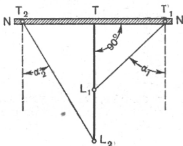
Рис. 104. Зависимость равномерности освещенности негатива от расстояния источника света
