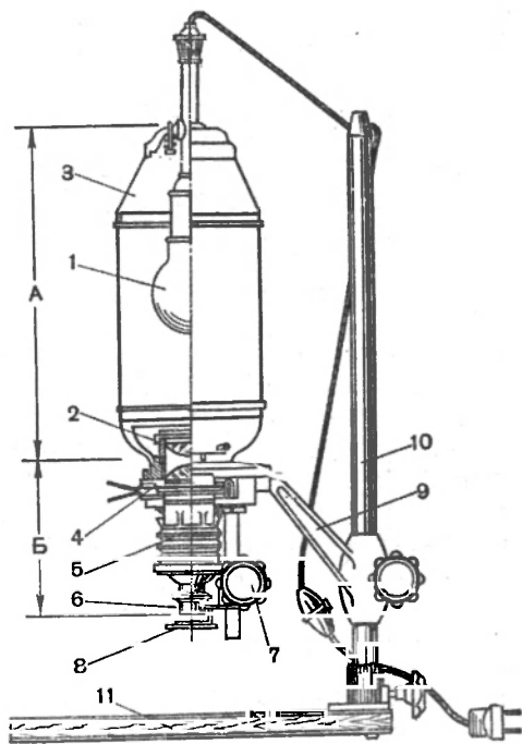
Рис. 71. Основные узлы конденсорного фотоувеличителя
