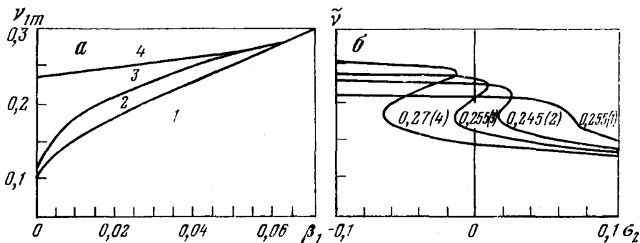
Рис. 14. Зависимость формы выходной характеристики реакции S_1 \xrightarrow{E(R,T)} S_2 от параметров
