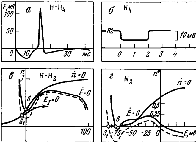
Рис. 42. Отсутствие анодно-размыкательного ответа в модели Нобля N_4 (б). Для сравнения показано возникновение ответа в модели Ходжкина — Хаксли H-N_4 (а)
