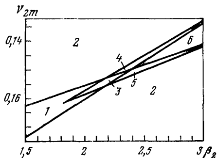
Рис. 15. Параметрический портрет модели (2.7) проточной реакции S_1 \xrightarrow{E(R,T)} S_2 в случае изостерического угнетения олигомерного фермента E(R, T) субстратом S_1
