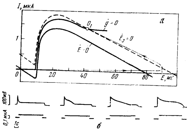
Рис. 57. Продленные потенциалы действия в мембране предсердия лягушки а — фазовый портрет, особая точка O_1 устойчива. ФП предсказывает возникновение второго устойчивого значения потенциала ( \sim 40 \text{ мВ} ); б — ответы мембраны на внешний ток. При увеличении тока от 0,09 \mu\text{A} (крайняя левая запись) до 0,12 \mu\text{A} (крайняя правая запись) длительность ответа возрастает примерно в 7 раз
