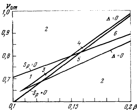
Рис. 25. Параметрический портрет модели (3.7) энергетического метаболизма (3.1), построенный в плоскости параметров источника \beta и v_{om} при \beta_4 = 0,01, \beta_6 = 0,1, \epsilon = 0,05, \eta = 1, \kappa_6 = 0,5
