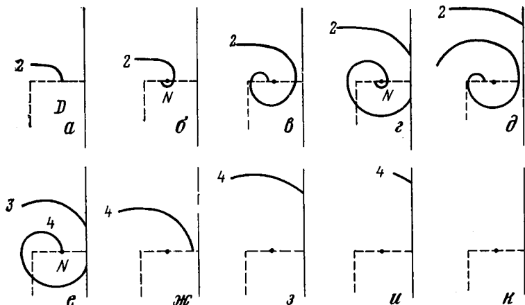
Рис. 69. Конечное время жизни ревербератора в неоднородной среде
