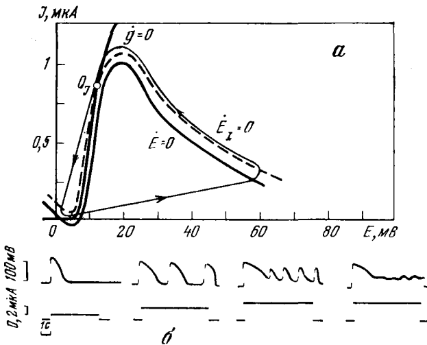
Рис. 56. Повторные ответы в мембране трабекулы предсердия лягушки а — фазовый портрет; особая точка O_1 неустойчива. ФП предсказывает возникновение автоколебаний под током (предельный цикл показан стрелкой); б — ответы мембраны на внешний ток различной амплитуды
