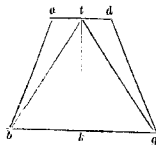
Copulabo rectas .... quadrilaterum abgd. s (fol. 78 recto, lin. 15-21; pag. 126, lin. 25-40).
