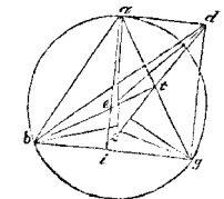
fol. 107 verso. « embadum pyramide .... triangulorum » (fol. 107 verso, lin. 4-7; pag. 169, lin. 23-25).
