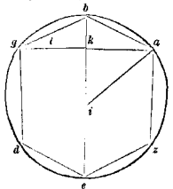
« corda .ag. .... totius exagoni » (fol. 106 verso, lin. 10, 11-13, 20; pag. 168, lin. 12-20).
