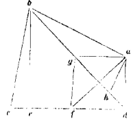
lineæ afc. ... 7. per 15. á fol. 108 recto, lib. 24-30; pag. 171, lib. 29-32.
