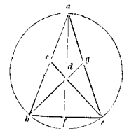
* d et recte ad. ... abg. quidem pluri (fol. 138 recto, lin. 21-29; 31; pag. 213, lin. 8-15).
