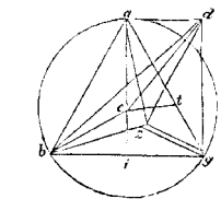
« zb. zg., et .... recte zb. » (fol. 107 recte, lin. 23-26; pag. 169, lin. 12-15).
