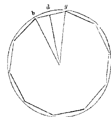
6 est corda ... et diuiserimus ... (fol. 139 verso, lin. 33-35 — marginis inferioris; pag. 215, lin. 26-28).
