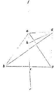
quadratum casus ... unumquodque ... 160. recto, lib. 14-14; pag. 170. lib. 43 — pag. 171, lib. 48.
