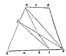
puncta cd. .... quomodo in duo s (fol. 78 verso, lin. 26-32; pag. 127, lin. 21-27).
