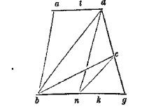
puncta cd. .... quomodo in duo s (fol. 78 verso, lin. 26-32; pag. 127, lin. 21-27).
