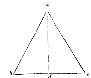
* g multiplicauerimus ... \frac{1}{4} 1 . Vnde si (fol. 138 recto, lin. 8-14; pag. 213, lin. 25-31).
