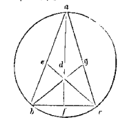
* g multiplicauerimus ... \frac{1}{4} 1 . Vnde si (fol. 138 recto, lin. 8-14; pag. 213, lin. 25-31).
