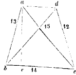
que sunt ... de 160., cum á fol. 108 recto, lib. 24-35; pag. 170, lib. 32-48.
