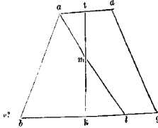
et basis .... quadrilaterum a (fol. 78 verso, lin. 2-7 e 8; pag. 127, lin. 10-15).
