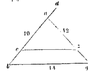
a. ba. in .ad. .... quod est a recta .e. in a (fol. 73 verso, lin. 2-7 e r. pag. 119, lin. 25-31).
