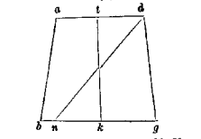
inter dg. .... a linea bc. s (fol. 78 verso, lin. 12-17; pag. 127, lin. 10-20).
