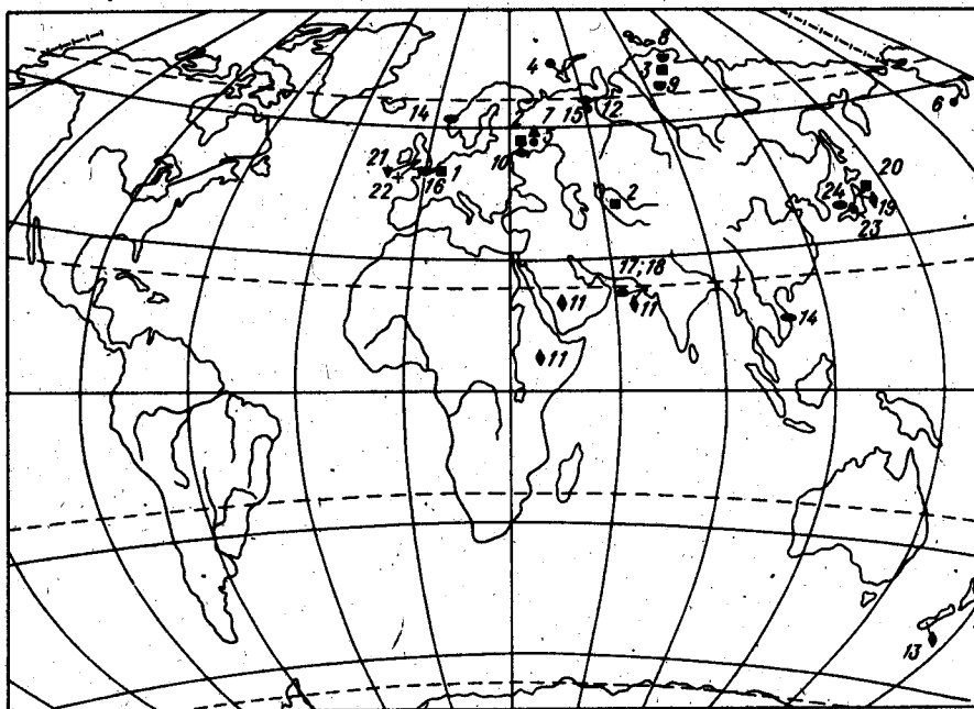
Рис. 8. Распространение представителей надсемейства Arcasea в волжском веке. Усл. обозн. см. рис. 2.
