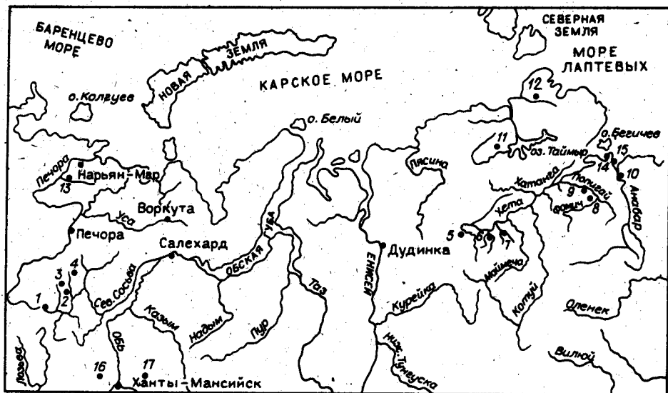
Рис. 1. Схематическая карта района сборов верхнеюрских и нижнемеловых Агсаеа.
