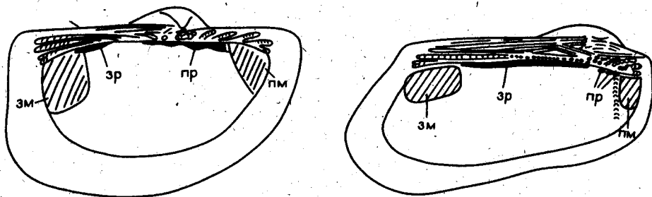
Рис. 14. Внутреннее строение раковины рода Grammatodon (вид G. lopsiensis sp. n., р. Лопсия, обн. 41, сл. 1, шф 3).
