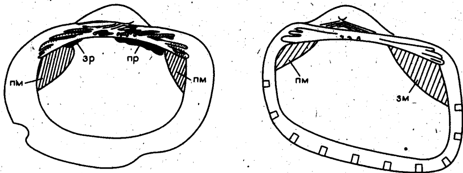
Рис. 12. Внутреннее строение раковины рода Lopatinia (вид L. uratica sp. n., р. Маурья, обн. 5, осьшь).
