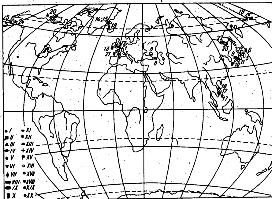
Рис. 2. Распространение представителей надсемейства Arcascea в геттанге, синеморе, плинсбахе, тоаре и аалене.
