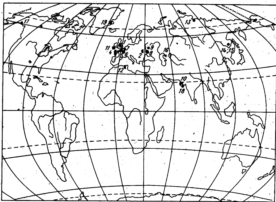
Рис. 4. Распространение представителей надсемейства в бате. Усл. обозн. см. рис. 2.
