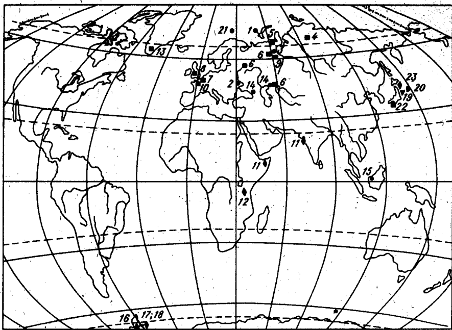
Рис. 7. Распространение представителей надсемейства Arcasea в кимеридже. Усл. обозн. см. рис. 2.
