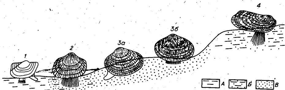
Рис. 24. Палеоэкологическая реконструкция прижизненного положения позд-неюрских – раннемеловых аркаей.
