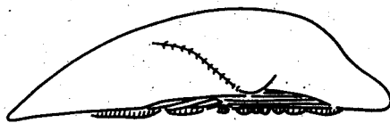
Рис. 23. Строение связочной площадки вида Grammatodon gracialis sp. n. р. Анабар, обн. 5, сл. 10, инт. 0-1,5 м.
