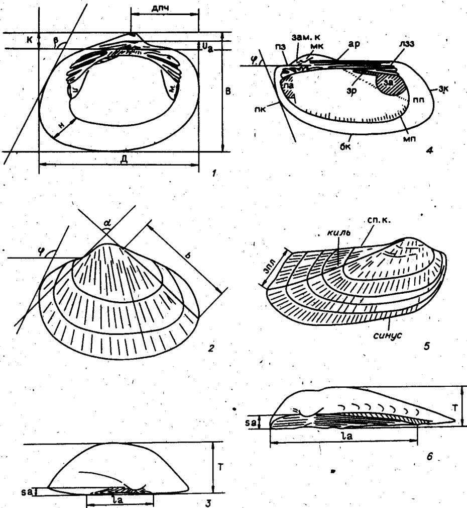
Рис. 11. Строение раковины у представителей родов Loratinia (1,2,3) и Cosmetodon (4,5,6).
