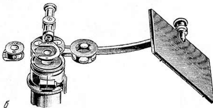
Рис. 18. Рисовальный прибор Аббе а — оптическая схема; б — общий вид
