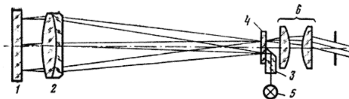
Рис. 22. Автоколлиматор системы Аббе
