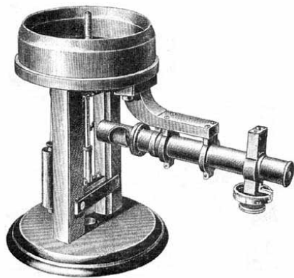
Рис. 25. Сферометр Аббе
