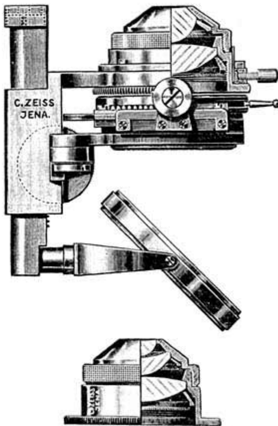
Рис. 15. Осветительный аппарат Аббе (1872 г.)
