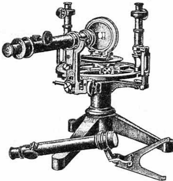
Рис. 21. Спектрометр Аббе
