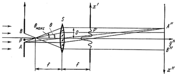
Рис. 5. Схема образования изображения в микроскопе по Аббе
