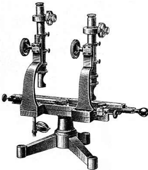
Рис. 26. Вертикальный компаратор Аббе
