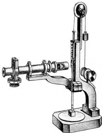
Рис. 24. Контактный микрометр Аббе
