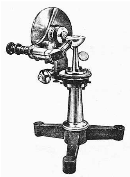
Рис. 27. Кристаллорефрактометр Аббе
