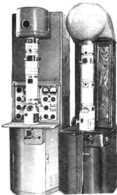
Рис. 8. Советские электронные микроскопы марки ГОИ: слева - конструкция 1955 г.; справа - 1947 г.; Политехнический музей. Москва
