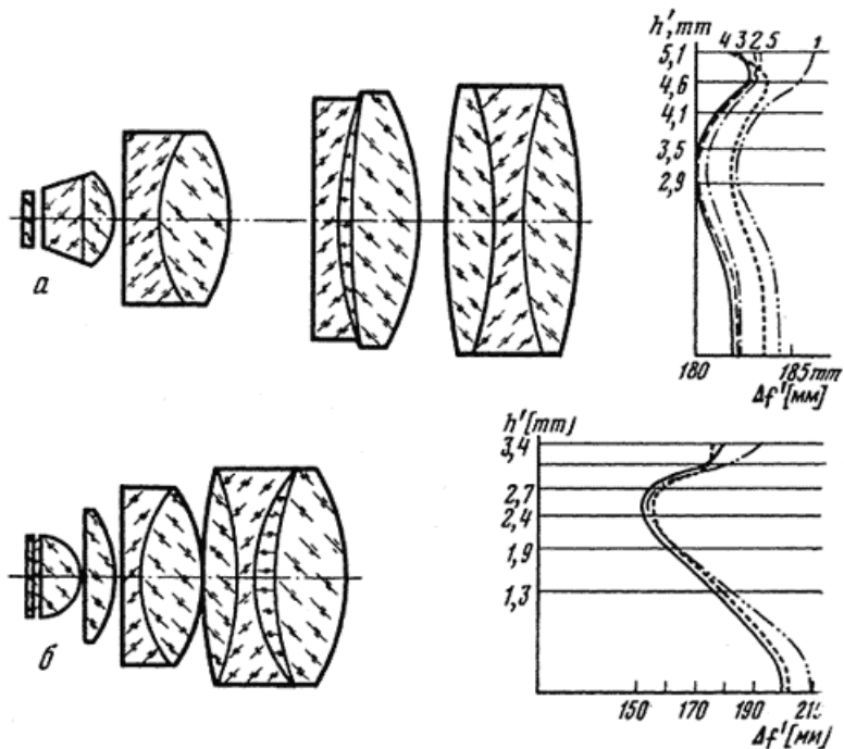
Рис. 11. Апохроматические объективы Аббе и графики их aberrаций
