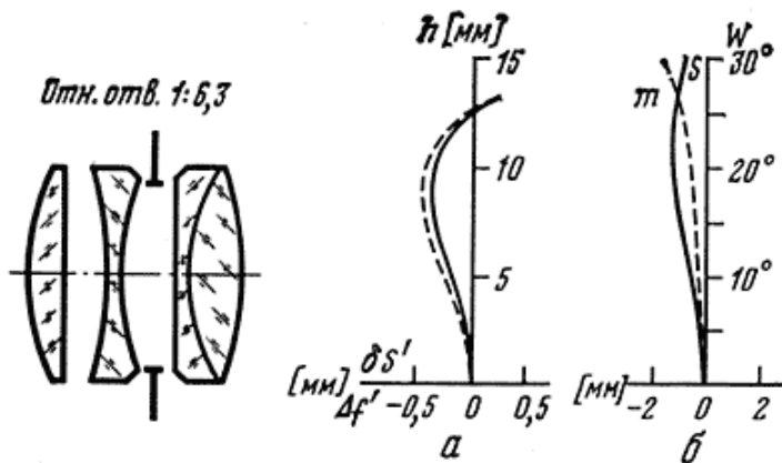
Рис. 13. Фотографический объектив П. Рудольфа «Тессар» и графики его aberrаций. Обозначения см. рис. 12
