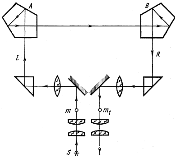
Рис. 29. Оптическая схема стереодальномера Аббе (1893 г.)
