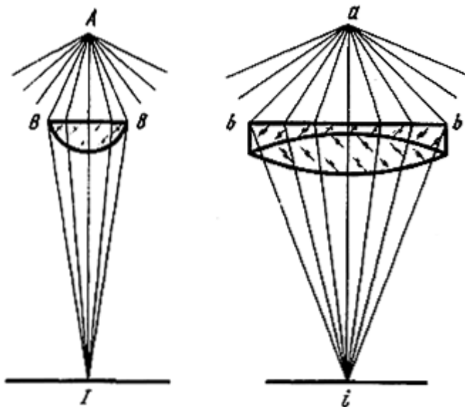
Рис. 4. К определению отверстия угла
