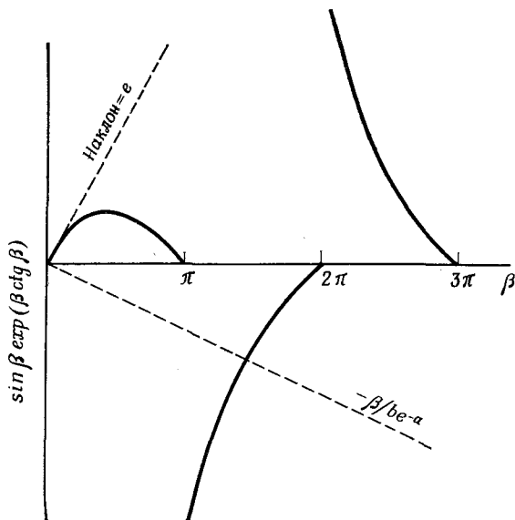
Рис. 23. График \sin \beta \exp(\beta \operatorname{ctg} \beta) как функции \beta Решения уравнения \beta = -b \exp(-a) \sin \beta \exp(\beta \operatorname{ctg} \beta) представляют собой пересечения этого графика с графиком для -b \exp(-a) .
