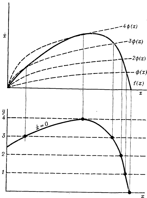
Рис. 15. Построение кривой \dot{x} = 0 .
