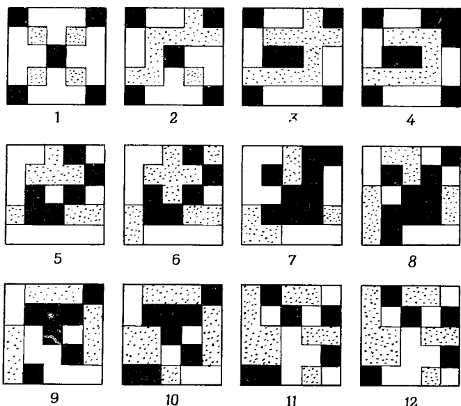
Рис. 36. Имитация системы, представленной на рис. 35, в среде, состоящей из 25 клеток.
