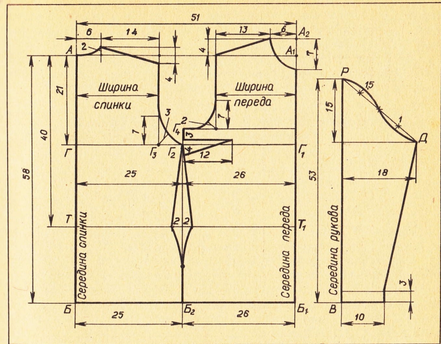
Рис. 73. Построение чертежа выкройки основы жакета.
