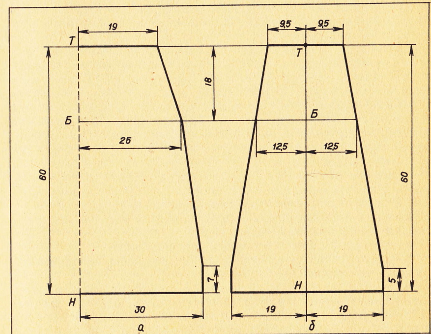
Рис. 76. Построение чертежей выкройки юбки: а — из двух клиньев; б — из четырех клиньев.
