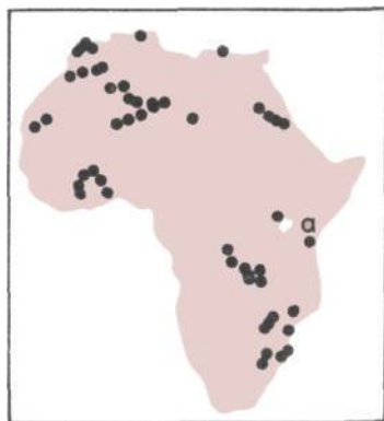
Олдованская культура в Африке. На карте показаны места находок каменных орудий, похожих на орудия из Олдувая (отмечено буквой а).
