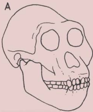
Сравнение черепов (изображения с поворотом в три четверти). А — Череп австралопитека африканского. Б — Череп современного человека.
