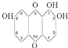
1, 2, 7 Trioxyanthrachinon.
