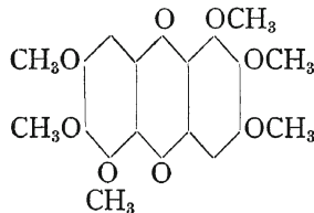
Rufigallussäurehexamethyläther.
