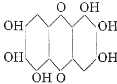
Rufigallussäure (1, 2, 3, 5, 6, 7 Hexaoxyanthrachinon.)
