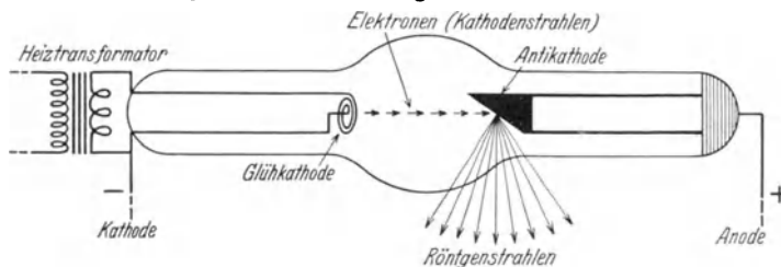
Abb. 1. Röntgenröhre.
