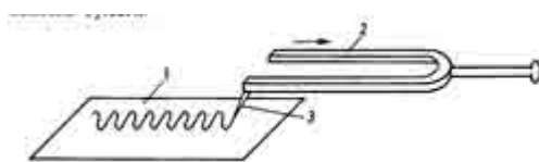
Схема 3. Визуализация колебаний ножек камертона 1 – бумага; 2 – камертон; 3 – карандаш
