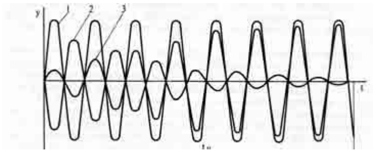
Схема 11. Вынужденные колебания 1 — периодическая внешняя сила; собственные затухающие колебания вибратора; 3 — вынужденные колебания вибратора
