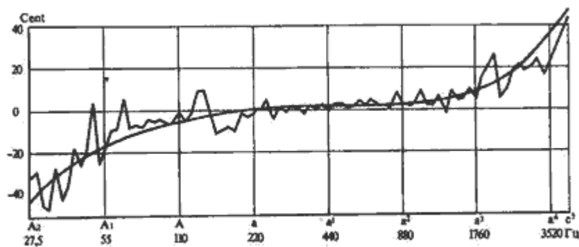
Схема 15. Кривая настройки пианино и ее сглаженная форма
