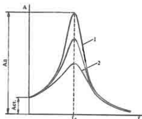
Схема 12. Резонансные кривые
