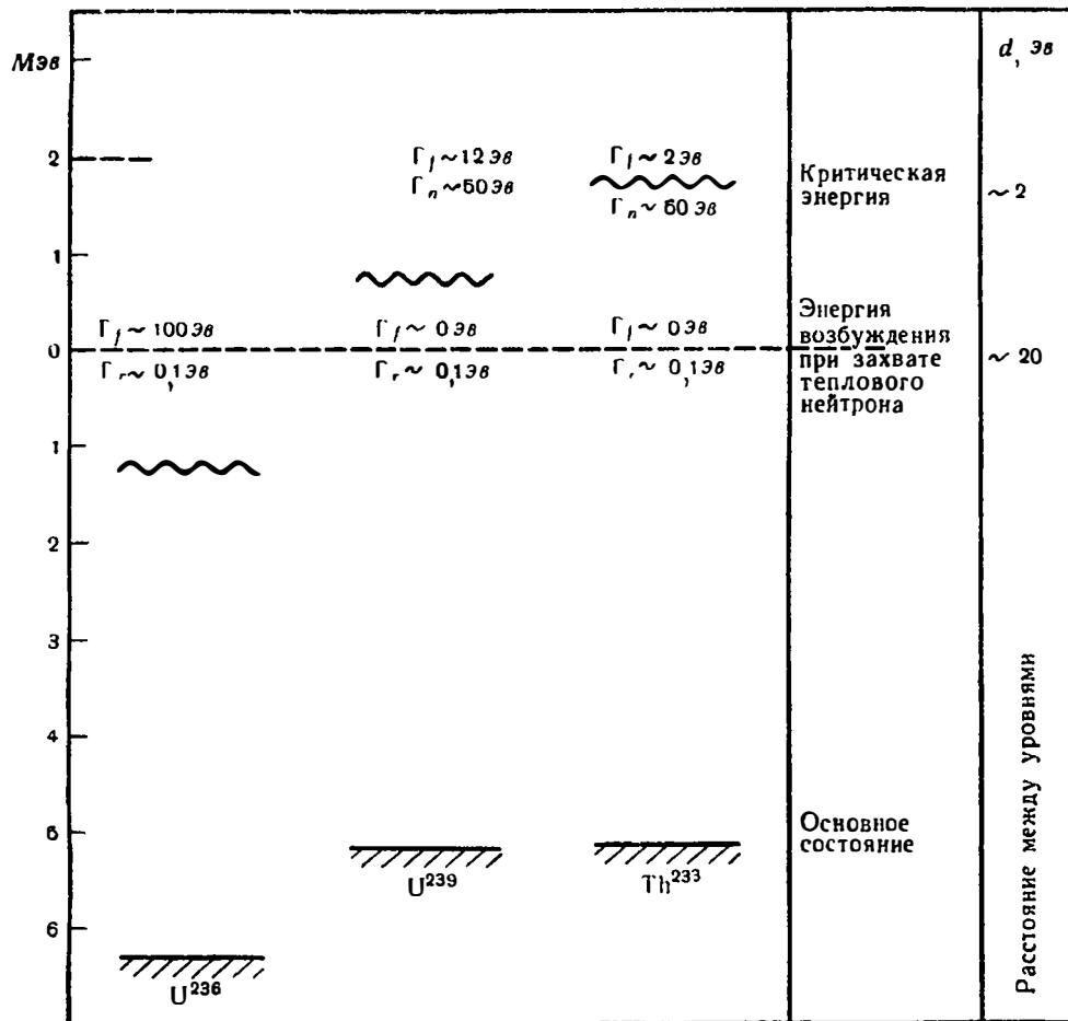
Рис. 7. Сравнительная сводка оценочных значений энергии деления, энергии связи нейтрона, расстояний между уровнями, а также ширины деления и нейтронных ширины для трех ядер, в отношении которых имеются экспериментальные данные. Для быстрых нейтронов значения \Gamma_f , \Gamma_n и d менее надежны, чем их отношения. Числа, расположенные в самой верхней части рисунка, во всех случаях соответствуют энергии нейтронов, равной 2 Мэв
