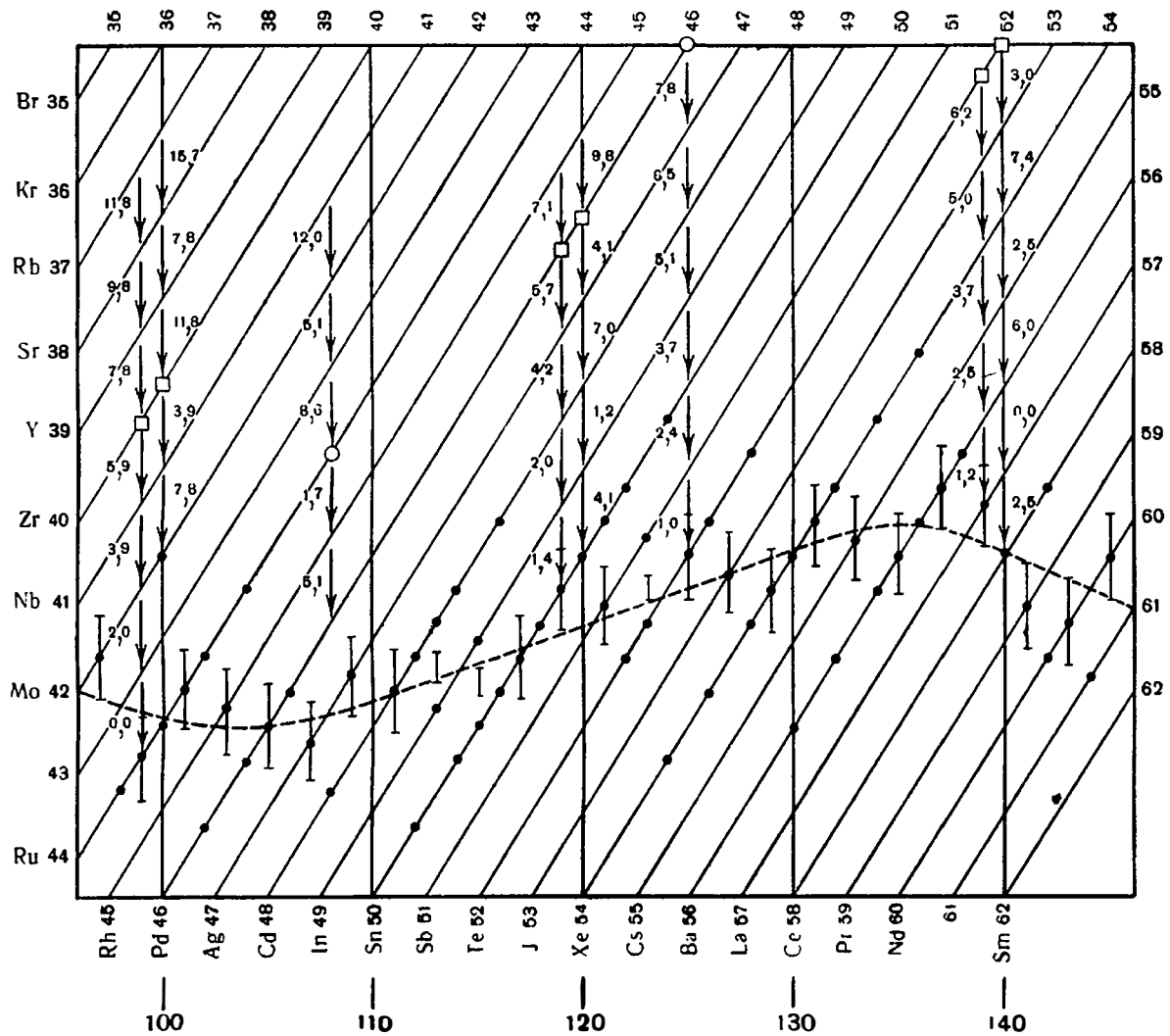
Рис. 8. Бета-распад осколков деления, приводящий к стабильным ядрам. Стабильные ядра обозначены малыми кружками. Примером является ядро {}_{50}\text{Sn}^{120} , расположенное у нижнего конца стрелки, помеченной числом 4,1; это число указывает оценку энергии (в \text{Мэв} ) бета-превращения предшествующего ядра {}_{49}\text{In}^{120} (см. раздел I). Заметно характерное различие в энергиях последовательных переходов между ядрами с четными и нечетными массовыми числами. Пунктирная линия проведена согласно рекомендации Гамова таким образом, чтобы не выходить за отмеченные пределы стабильности ядер с нечетным массовым числом. В разделе I говорится о том, как использовать данные этого рисунка
