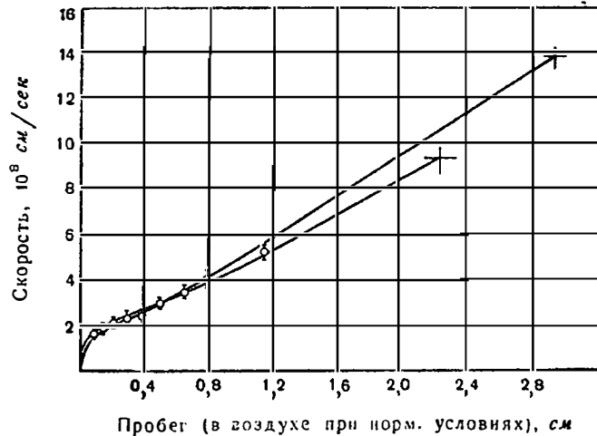
Рис. 1. Соотношение скорость—пробег для осколков деления
