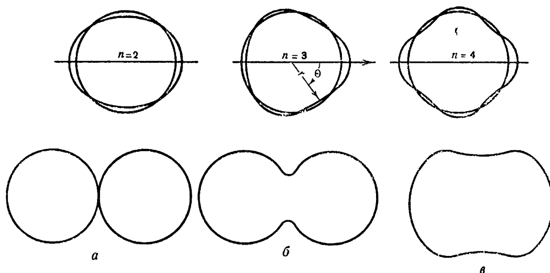
Рис. 2. Малые деформации жидкой капли, описываемые формулой \delta r(\theta) = \alpha_n P_n(\cos \theta) (верхняя часть рисунка), приводят к характерным колебаниям около сферической формы устойчивого равновесия, даже если жидкость имеет некоторый равномерно распределенный электрический заряд. Однако по достижении зарядом критического значения, равного [10 \times (\text{коэффициент поверхностного натяжения}) \times (\text{объем})^{1/2}] , сферическая форма становится неустойчивой по отношению к бесконечно малым деформациям четного типа (с n=2 ). С другой стороны, при несколько меньших значениях заряда требуется конечная деформация (в) для достижения конфигурации неустойчивого равновесия, и с уменьшением плотности заряда критическая форма постепенно переходит (в, б, а) в две незаряженные сферы, разделенные бесконечно малым расстоянием (а)
