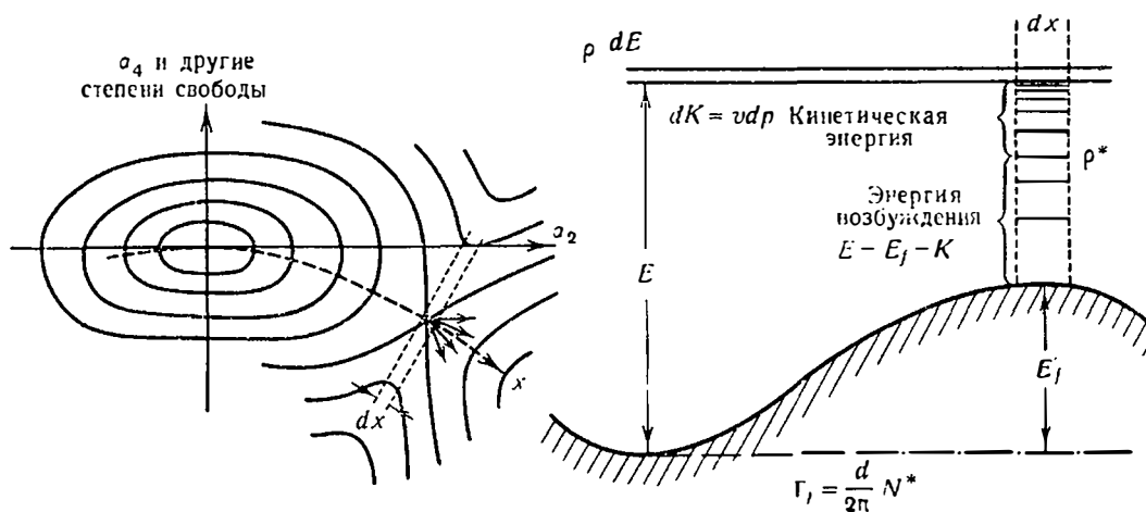
Рис. 3. Потенциальная энергия, связанная с произвольным изменением формы ядра, в зависимости от параметров, определяющих деформацию, может быть графически представлена некоторой поверхностью, горизонтали которой схематически изображены в левой части рисунка. Перевал, или седловидная точка, соответствует критической деформации неустойчивого равновесия. В той мере, в какой мы можем пользоваться классической картиной, течение реакции деления можно уподобить поведению шарика, лежащего в углублении в начале координат (сферическая форма ядра) и внезапно испытывающего толчок, который заставляет его колебаться около положения равновесия, описывая сложную фигуру Лиссажу. Если энергия достаточно велика, шарик с течением времени может случайно получить скорость в нужном направлении и преодолеть седловидную точку (это соответствует тому, что произошло деление) при условии, что он не потеряет до этого своей энергии (это соответствует испусканию нейтрона или гамма-кванта). Справа для иллюстрации расчета вероятности деления в единицу времени, который делается в тексте, изображено сечение поверхности вдоль линии, пересекающей барьер деления
