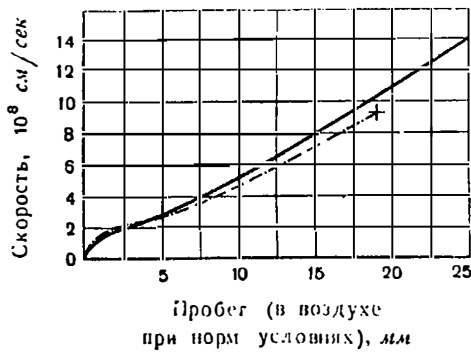
Рис. 1. Эмпирические кривые скорость — пробег в аргоне (штрих-пунктирная кривая — для тяжелого осколка, сплошная кривая — для легкого)
