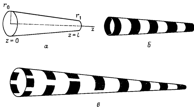
Рис. 6.5. Область реакции с диффузией в виде конической поверхности: а — геометрические данные; б — r_0 < r < r_1 , r_1 мал; в — r_1 мал, а r_0 достаточно велико для возникновения двумерных эффектов вблизи z = 0 .
