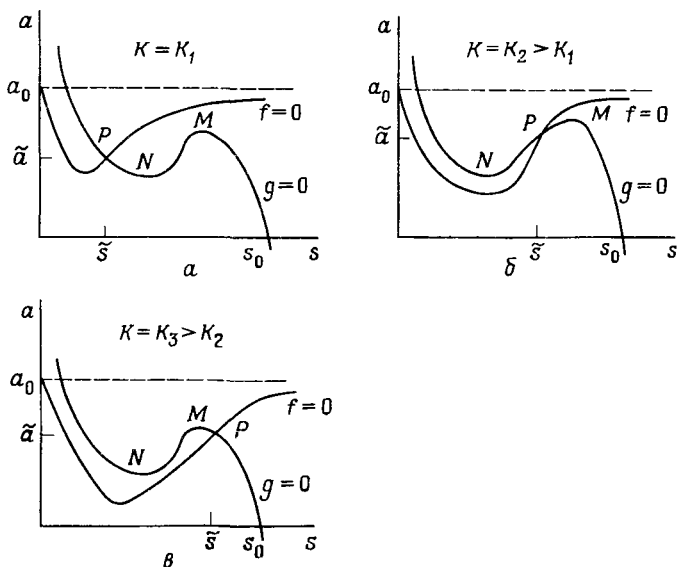
Рис. 6.2. Схема изоклин скоростей реакций f(s, a) = 0 и g(s, a) = 0 с f и g из уравнений (6.3). Стационарному состоянию соответствует точка P(\tilde{s}, \tilde{a}) . В случаях a и \beta система устойчива, в случае b может наблюдаться диффузионная неустойчивость.
