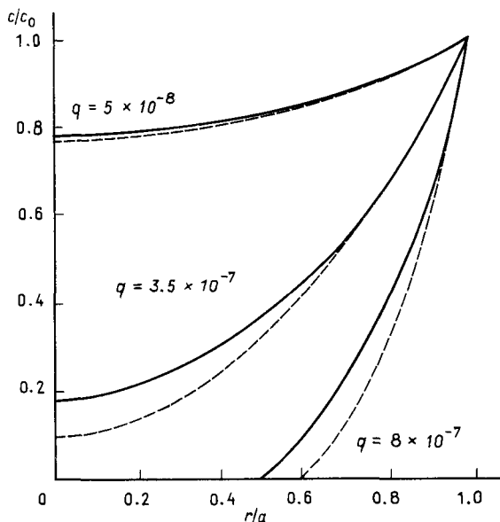
Рис. 2.7. Концентрация кислорода в мышечном волокне при различных значениях метаболической активности q моль/ (\text{см}^3 \cdot \text{с}) . Сплошные линии — диффузия, облегченная миоглобином; штриховые линии — простая диффузия. Условия указаны в табл. 2.4.
