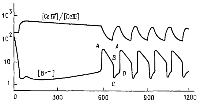
Рис. 4.7. Потенциметрические экспериментальные кривые \lg[\text{Br}^-] и \lg\{[\text{Ce IV}]/[\text{Ce III}]\} из работы Филда, Керёса и Нойеса (1972) для типичных временных осцилляций в реакции Белоусова–Жаботинского (воспроизведено с любезного согласия авторов работы). По оси абсцисс – время в секундах; [\text{Br}^-] в молях \times 10^{-7} .
