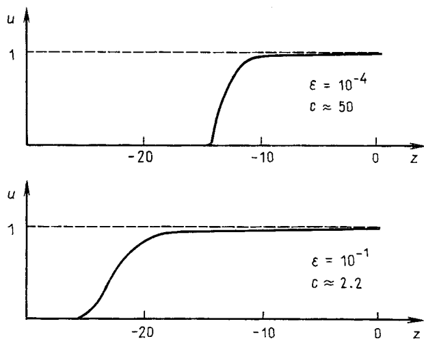
Рис. 5.10. Решения уравнения (5.75) типа волны, бегущей с минимально возможной скоростью c = k/2 + 2/k , \epsilon = 1/k^2 , для двух значений \epsilon . В начальной точке u = 1 - 10^{-6} .
