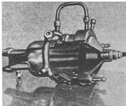
ОРМ-65 — один из наиболее совершенных ЖРД, созданных в РНИИ.
