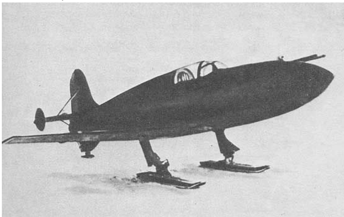
Ракетный самолет БИ.
