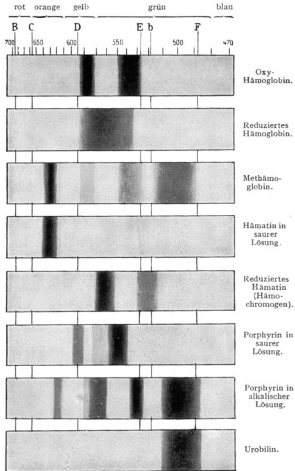
Abb. 50. Spektraltafel.
