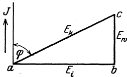
Abb. 13. Darstellung der Phasenverschiebung eines Wechselstromes zwischen Spannung und Strom im Vektorendiagramm.
