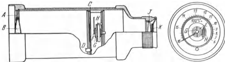
Abb. 52. Das Taschenpyrometer von Keiser & Schmidt. Die Strahlung fällt auf eine Bimetallspirale ( E , F ), die unmittelbar den Zeiger bewegt.
