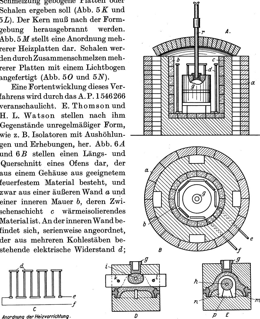
Abb. 6, A bis E. Erschmelzung von Quarz und Herstellung von Isolatoren nach E. Thomson. A. P. 1 546 266.
