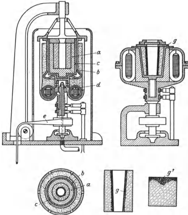
Abb. 15. Läuterung von Quarz nach British Thomson-Houston-Co. E. P. 252747 (1926).
