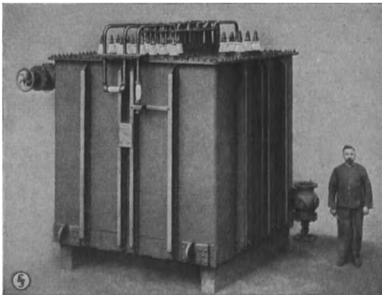
Abb. 10. Fertig zusammengebauter Drehstromöltransformator mit Umlaufwasserkühlung.
