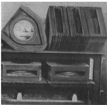
Abb. 15. Bodensteine zum Induktionsofen Ajax-Wyatt.
