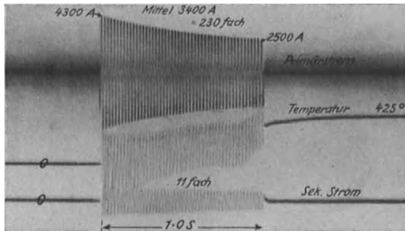
Abb. 3. Oszillogramm eines Überstromversuchs an einem Dreheisen-Strommesser nach Abb. 2a.
