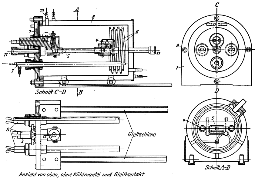
Abb. 5. Wolframrohröfen.
