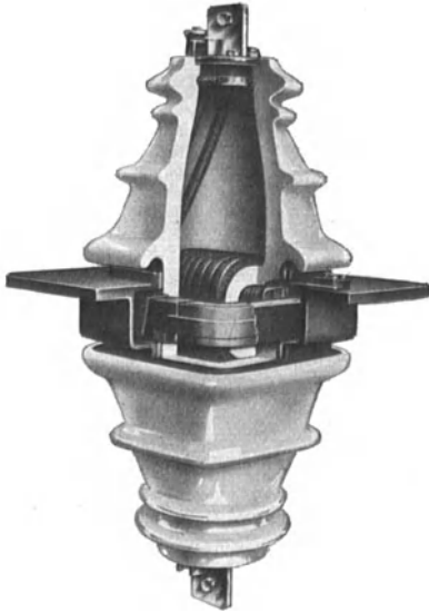
Abb. 11. Querloch-Durchführungs-Stromwandler mit Porzellan-Isolierung.
