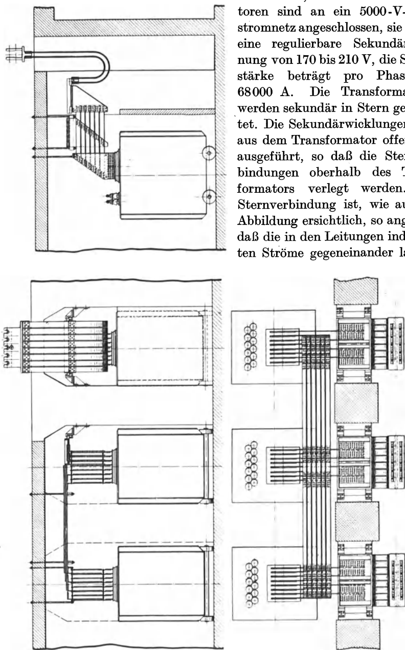
Abb. 22. Anordnung der Leitungsführung des aus drei Einphasentransformatoren kombinierten Drehstromtransformators von Karbidöfen.
