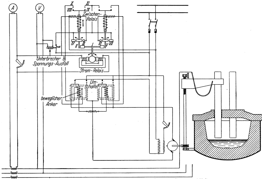
Abb. 39. Automatische Elektrodenregulierung, System AEG.
