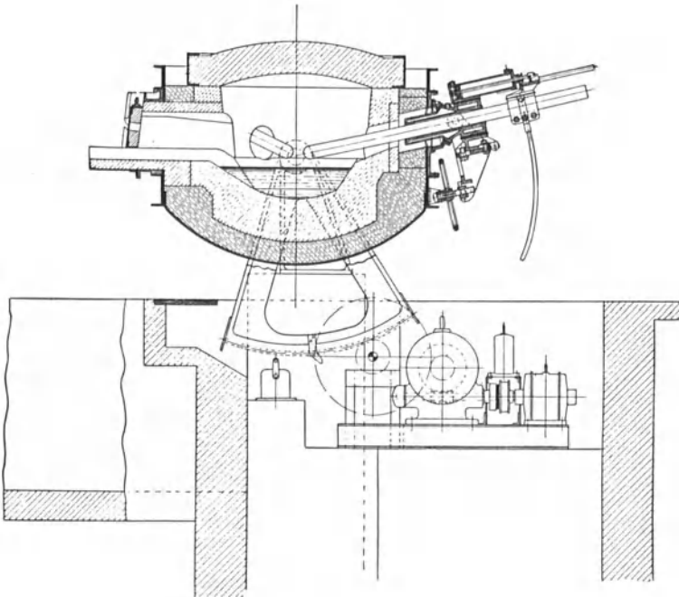
Abb. 26b. Indirekte Lichtbogenheizung.
