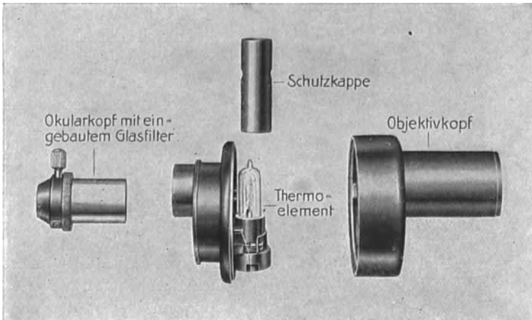
Abb. 49. Das „Ardometer“ von Siemens & Halske.
