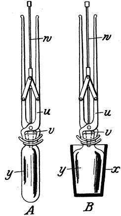
Abb. 9. Formzangen nach Bottomley und Paget. D.R.P. 174509.
