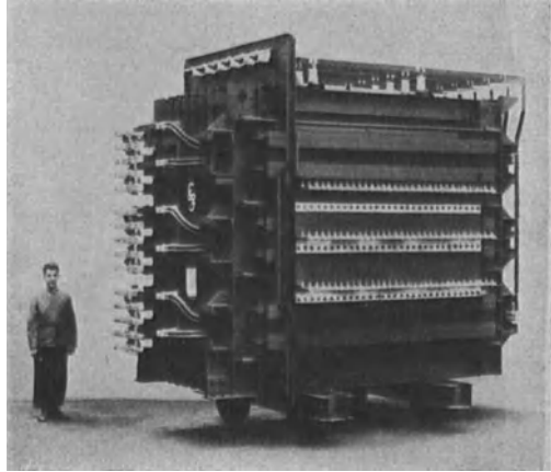
Abb. 11. Drehstromtrockentransformator für Karbidofenbetrieb.
