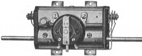
Abb. 24. Zweiteilige Meßkammer eines \text{CO}_2 -Messers mit aufgebaute Regelwiderstand zur Nullpunkt-Korrektion.
