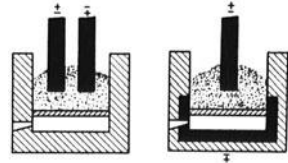
Abb. 30. Kombinierte Lichtbogen-Widerstandsheizung.
