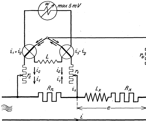
Abb. 19. Schaltbild für die Leistungsmessung bei Hochfrequenz mit zwei Thermo-Umformern. R_n = induktionsfreier Nebenwiderstand, L_x + R_x = induktiver Nutzwiderstand, W = Gleichstrom-Galvanometer, in Watt geeicht.
