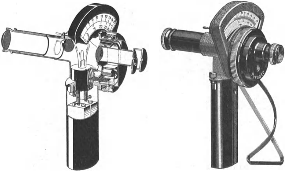
Abb. 64. Das „Pyropto“-Glühfadenpyrometer von Hartmann & Braun. Batterie, Anzeiginstrument, Glühlampe und Fernrohr sind zu einem einzigen Apparat vereinigt.
