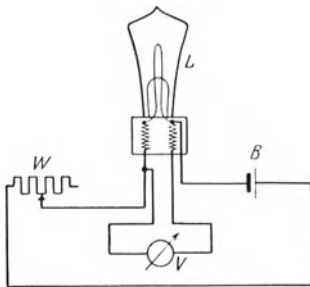
Abb. 65. Schaltung des Pyropto-Glühfadenpyrometers.
