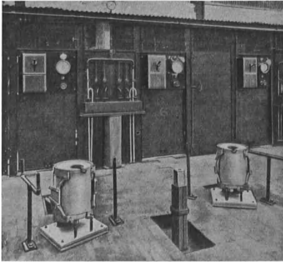
Abb. 23. Anlage von Laboratoriums-Hochfrequenzöfen mit Quecksilber-Funkenstrecke.
