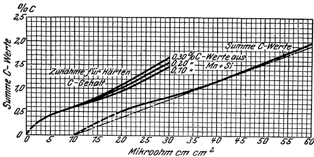
Abb. 22. Widerstandszunahme beim Härten von Stahl verschiedenen Kohlenstoff-Gehaltes. (Grundlage der Stahlanalyse nach Enlund.)
