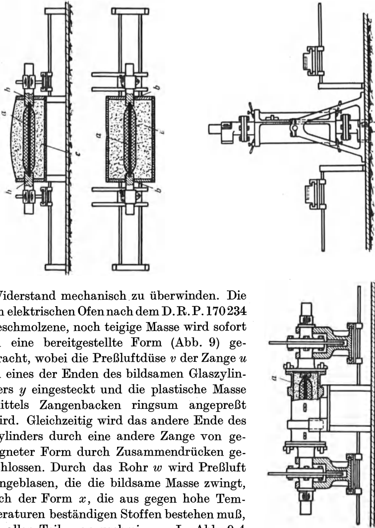
Abb. 8. Schmelzofen nach Bottomley u. Paget. D.R.P. 170234.
