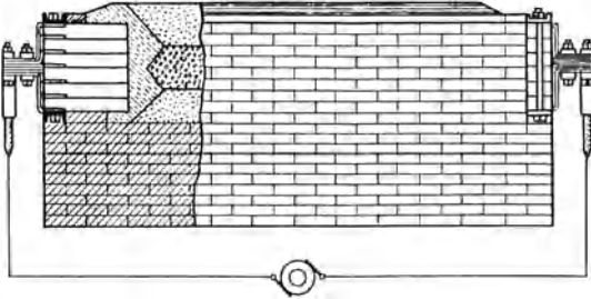
Abb. 1. Schematische Darstellung eines Siliziumkarbid-Ofens.
