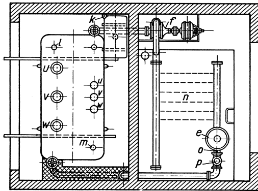
Abb. 5. Wasserkühlung durch eine außen liegende Kühlschlange.
