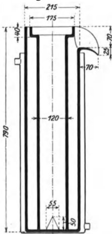
Abb. 24. Schwefelsäurekühltopf.
