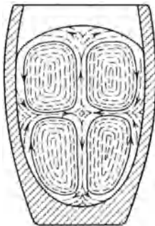
Abb. 24. Schematische Darstellung der Bewegung des Schmelzgutes im Hochfrequenzofen.
