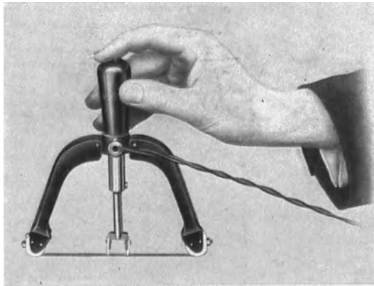
Abb. 40. Oberflächen-Thermoelement zur Temperaturmessung an konvexen, konkaven und ebenen Oberflächen (Siemens & Halske).
