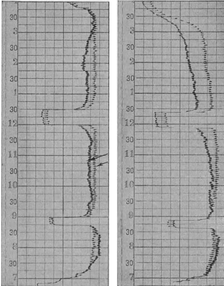
Abb. 20a, b. Diagramme eines Wirk- und Blindlast-Registrierapparates (dicke und dünne Kurve). Die ziemlich konstante Blindlast ist gegeben durch die Zahl der laufenden Maschinen, die Wirklast entspricht der Inanspruchnahme (20b am letzten Nachmittag des Jahresendes aufgenommen!) durch die Arbeiter und der Zusatzlast durch Beleuchtung (20a, Anstieg um 3 Uhr, Wintertag).
