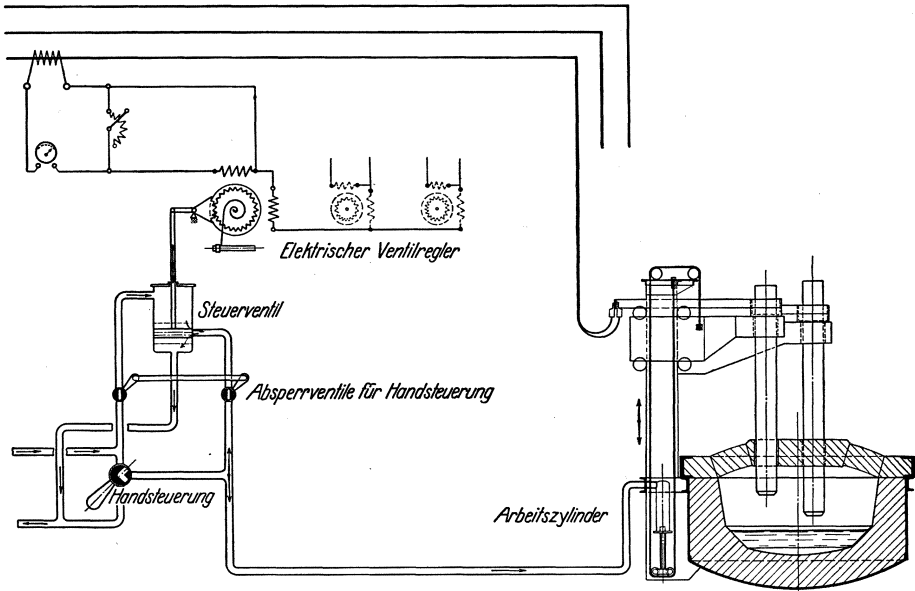
Abb. 42. Automatisch hydraulisch gesteuerte Elektrodenregulierung.
