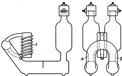
Abb. 29. Jaenicke-Quecksilberdampflampe. D. R. P. 384027.
