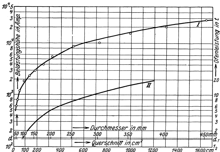
Abb. 3. Belastbarkeit von Graphitelektroden in Ampere in Abhängigkeit vom Querschnitt (I) und dazu gehörige Offenleistung in t (II).
