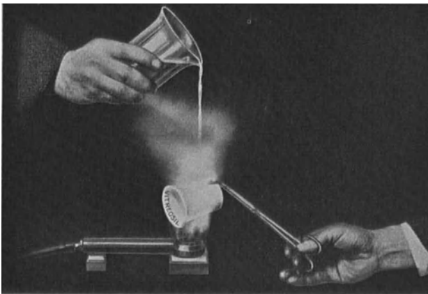
Abb. 18. Gleichzeitiges Glühen und Abschrecken eines Vitreosilbeckers.
