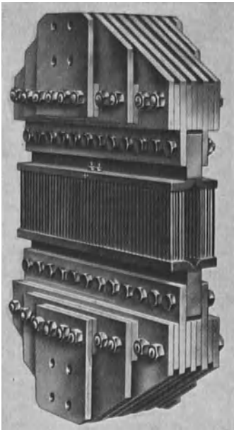
Abb. 6. Meßwiderstand für 25000 A Gleichstrom. Spannungsabfall 150 mV.
