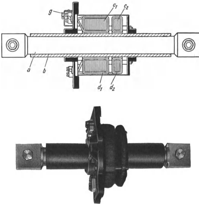
Abb. 8. Stabwandler mit Hartpapier-Isolierung b , Meßkern c_1 und Relaiskern c_2 .
