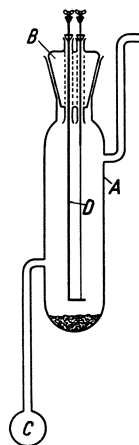
Abb. 19. Vorrichtung zum Züchten eines Metalkristalles aus der Gasphase.
