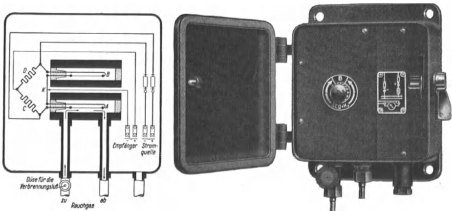
Abb. 27a, b. Gaslauf und Innenschaltung, Außenbild des Gebers für einen CO-Messer (Siemens & Halske).
