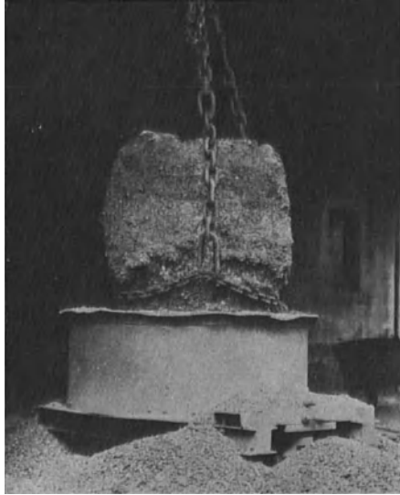
Abb. 10. Der Korundblock wird ausgehoben.
