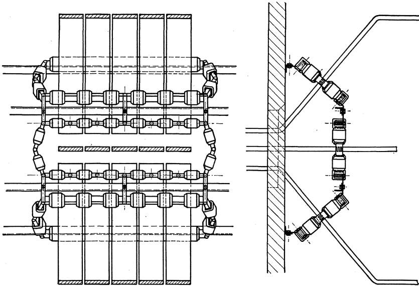
Abb. 14. Ketten-Stromwandler aus Einzelgliedern zur Messung sehr hoher Stromstärken.
