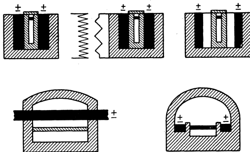
Abb. 49. Widerstandsstrahlungsheizung.
