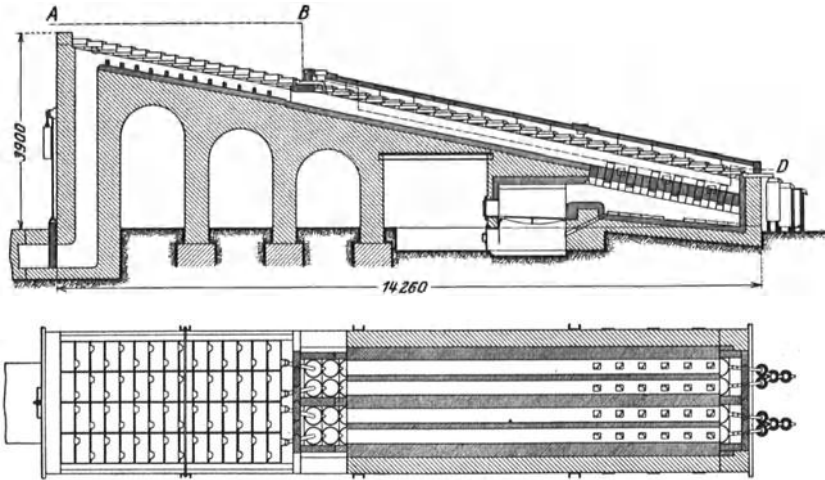
Abb. 23. Schwefelsäureanlage.
