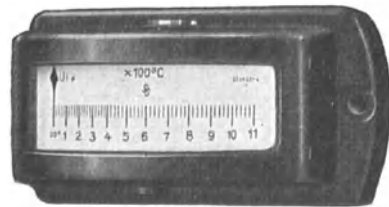
Abb. 34. Hochempfindliches Anzeigeinstrument in Profilform. Endausschlag 15 bis 25 mV, Widerstand 300 bis 500 \Omega .
