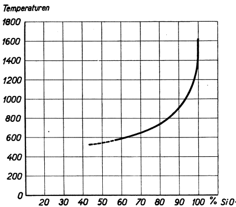
Abb. 1. Schematische Darstellung des Schmelzpunktes von Gläsern in Abhängigkeit vom Kieselsäuregehalt.
