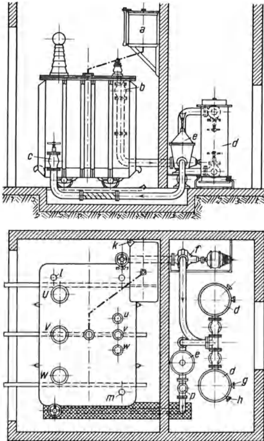
Abb. 6. Wasserkühlung durch einen außen liegenden Rohrkühler.
