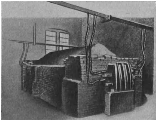
Abb. 2. Siliziumkarbid-Ofen.
