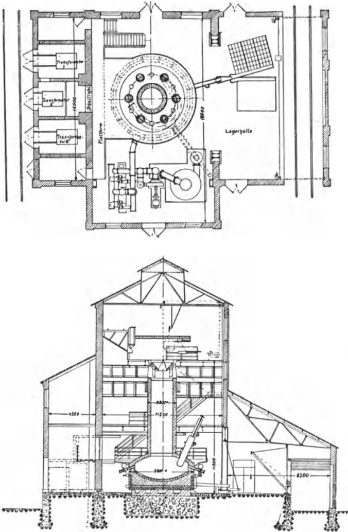
Abb. 56. Schema einer vollständigen elektrischen Ofenanlage.
