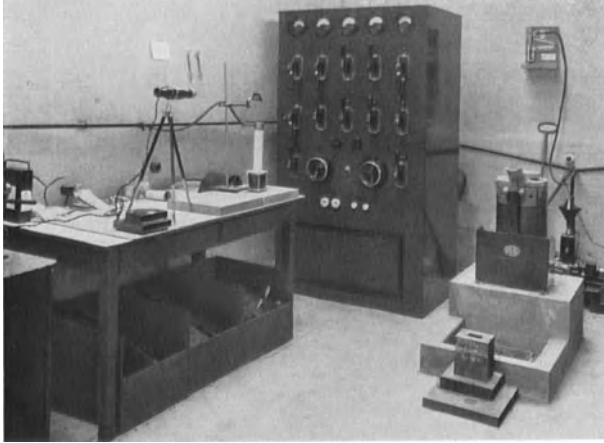
Abb. 71. Hochfrequenzofen, System Lorenz, für Laboratoriumszwecke.
