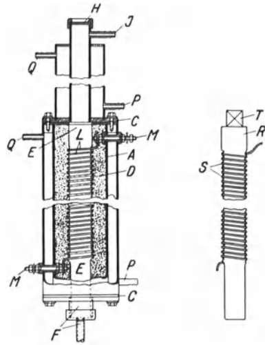
Abb. 4. Ofen mit Innenwicklung.
