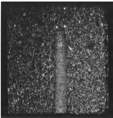
Abb. 24. Bohrung in gesintertem Wolframstab.
