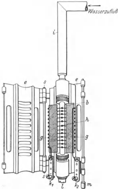
Abb. 41. Feuchtigkeitsmesser nach dem Psychrometerprinzip (Keiser & Schmidt).
