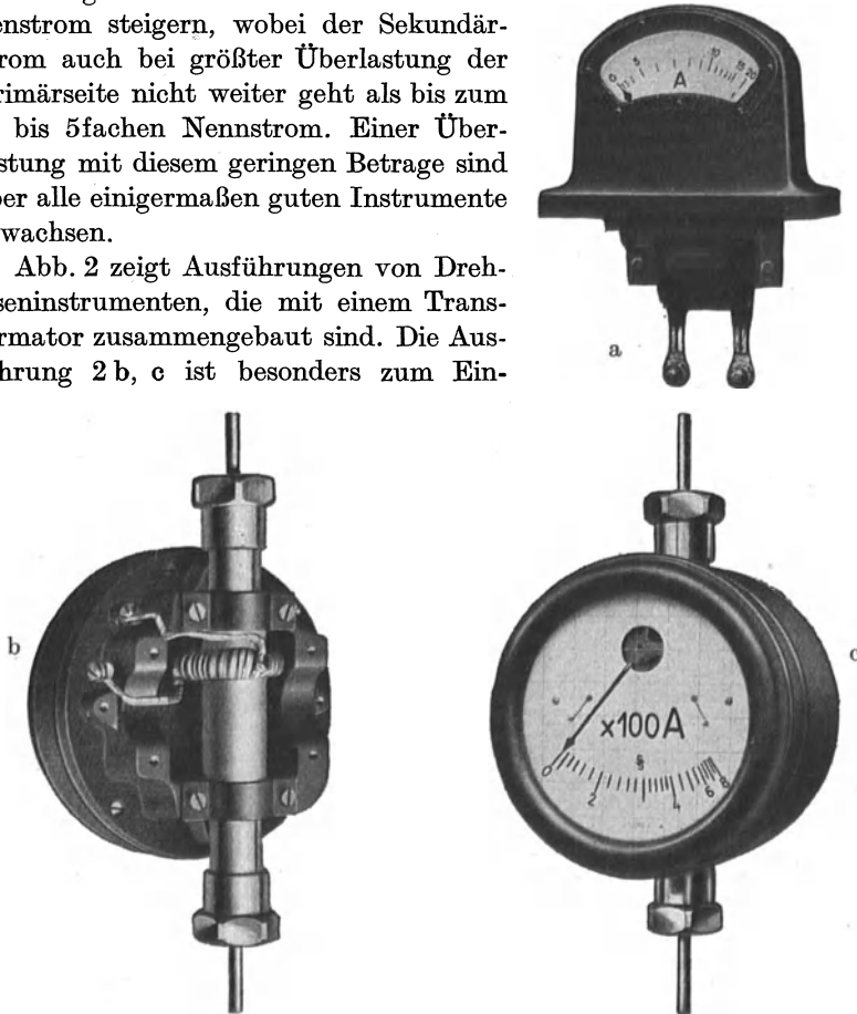
Abb. 2. Kurzschlußfeste Dreheisen-Instrumente mit Klein-Transformatoren zusammengebaut. a zum Einbau in Schaltkasten, b, c zum Einbau in Hochspannungsleitungen.
