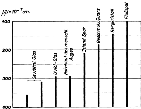
Abb. 22. Durchlässigkeit für ultraviolette Strahlen.
