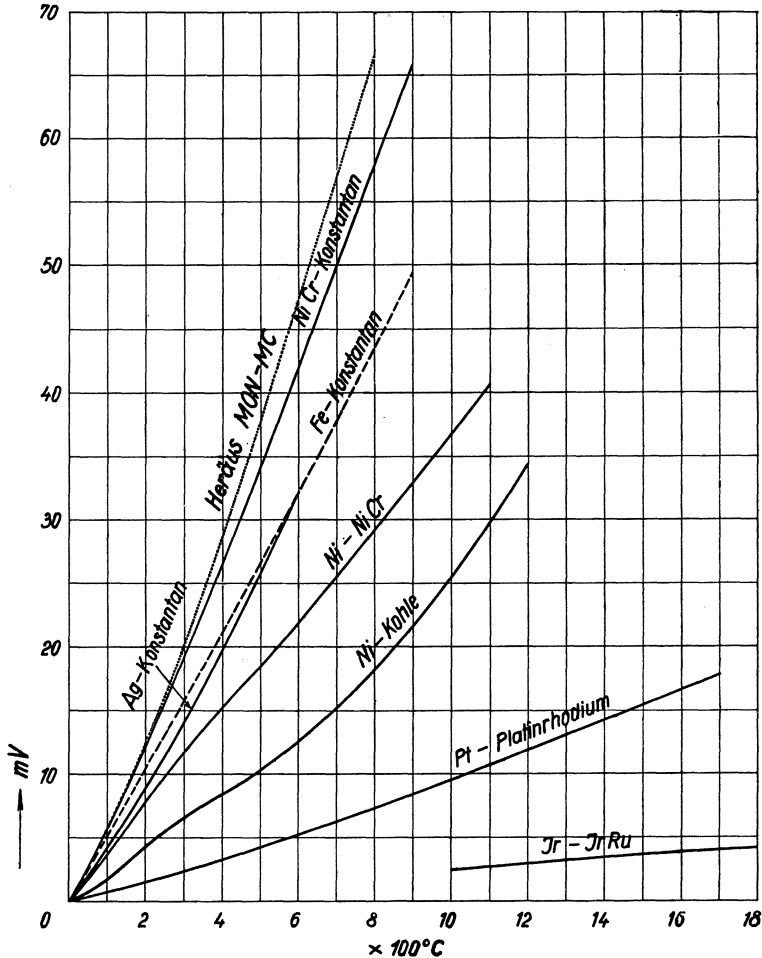
Abb. 33. Thermokraft verschiedener Elementpaare in Abhängigkeit von der Temperatur.
