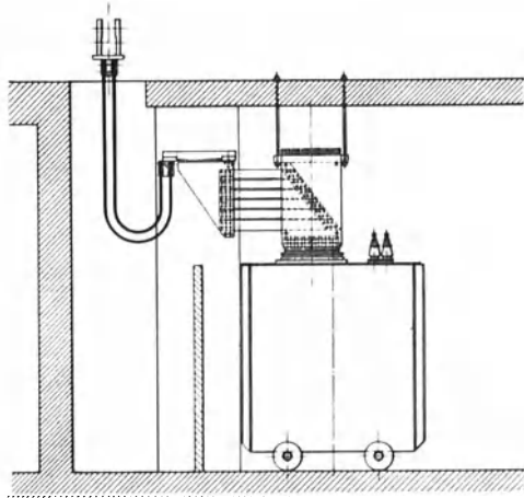
Abb. 23. Anordnung von Hochstromleitungen für Karbidöfen.
