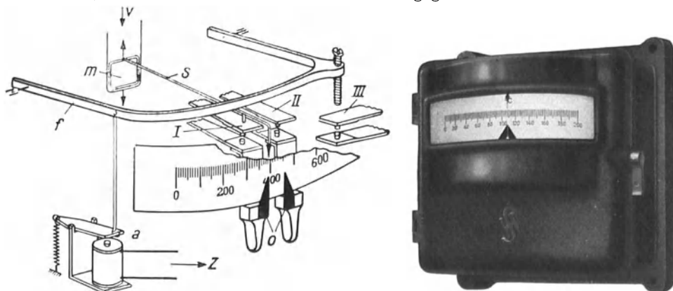
Abb. 43. Schema und Ausführung eines Temperatur-Reglers mit Bimetall-Motor zur Fallbügel-Betätigung (Siemens & Halske).
