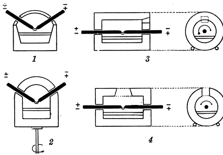
Abb. 26a. Indirekte Lichtbogenheizung.
