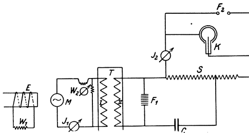
Abb. 10. Schaltbild des Kathodenstrahl-ofens.
