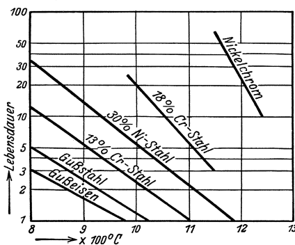
Abb. 37. Relative Lebensdauer verschiedener Pyrometer-Schutzhrohre bei Temperaturen von 300 bis 1250° C.
