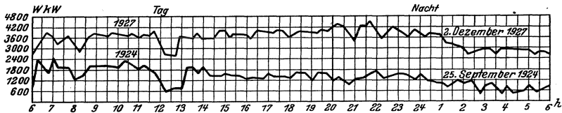
Abb. 1. Belastungskurve eines großen Metallwerkes.
