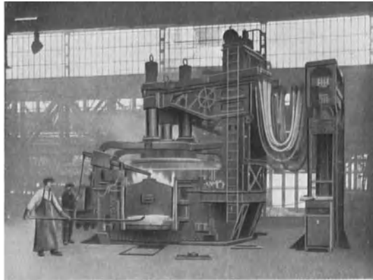
Abb. 59. 15 t-Drehstromlichtbogenofen, System Siemens & Halske.
