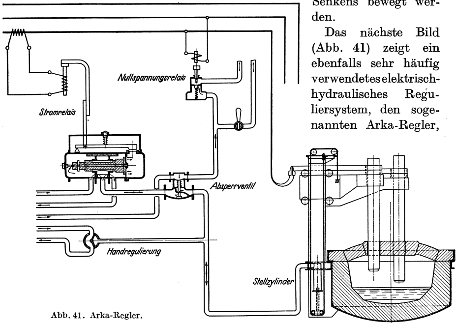
Abb. 41. Arka-Regler.
