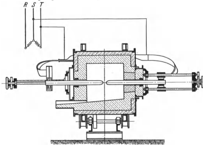
Abb. 2. Einphasen-Lichtbogen-Rollofen.
