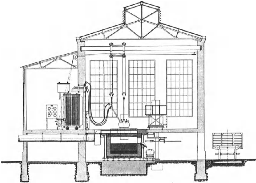
Abb. 31. Schnittzeichnung einer Karbidofenanlage.
