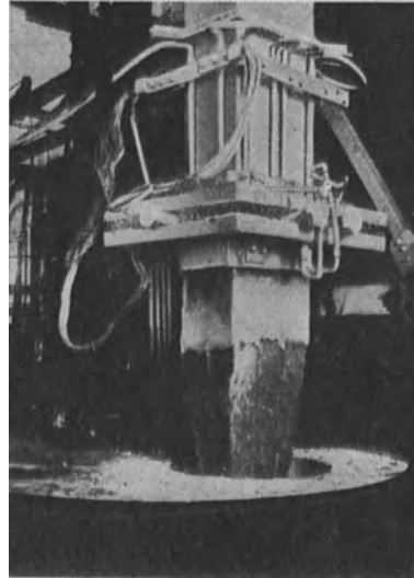
Abb. 34. Selbstbrennende prismatische Elektrode (Söderberg).
