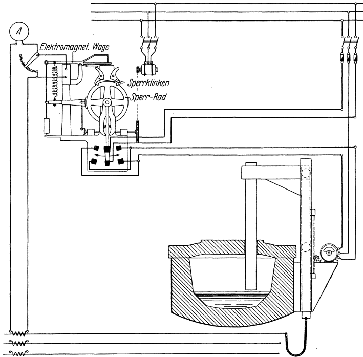
Abb. 43. Elektrodenregulierung (Tury-Regler).
