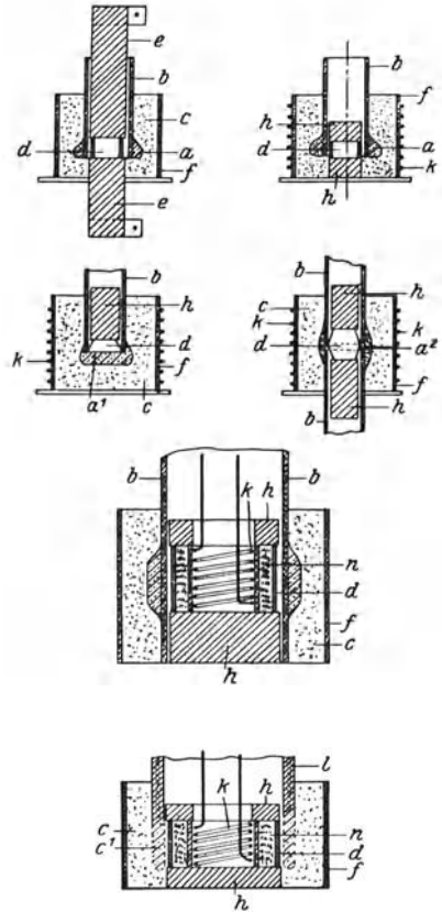
Abb. 13. Hochfrequenz-Induktionsofen der S. A. Quartz & Silice, Paris. F. P. 626432.
