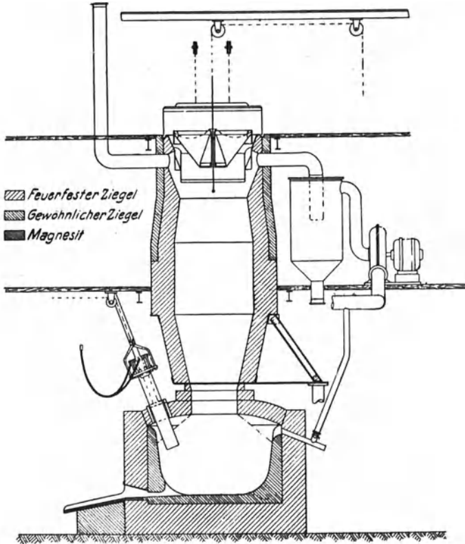
Abb. 55. Elektrischer Hochofen, System Grönwall.
