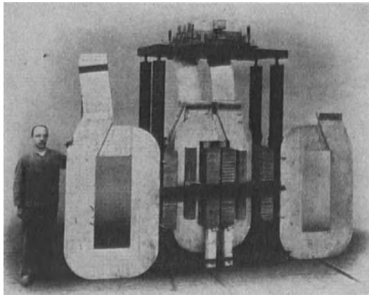
Abb. 8. Einphasentransformator mit sekundärer Spule auf dem Ölkessel montiert.
