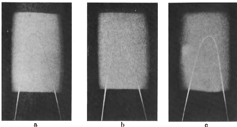
Abb. 60 a, b, c. Sehfeld eines Glühfadenpyrometers beim Anvisieren eines glühenden Blockes. a Temperatur zu tief eingestellt, b Temperatur richtig eingestellt, c Temperatur zu hoch eingestellt.
