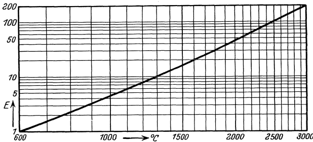
Abb. 47. Relative Zunahme der Gesamtstrahlungsenergie eines schwarzen Körpers für Temperaturen von 600 bis 3000° C.
