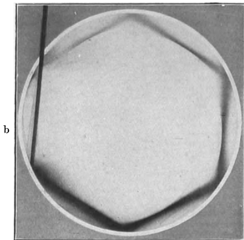
Abb. 45. Strahlungs-Reflexion und Absorption in einem Hohlraum mit kleiner Öffnung 1 .
