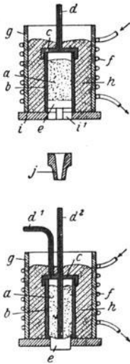
Abb. 12. Hochfrequenz-Induktions- ofen der S. A. Quartz & Silice, Paris. F. P. 585214.
