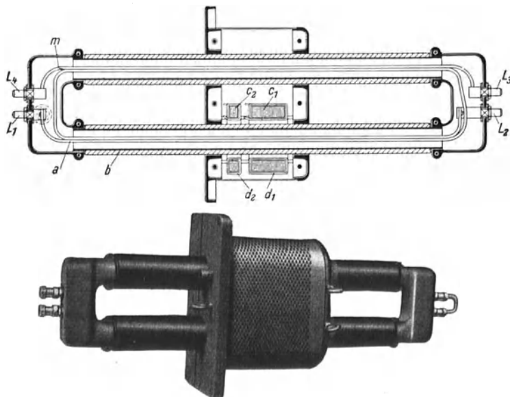
Abb. 9. Schleifen-Stromwandler mit Hartpapier-Isolierung b , Meßkern c_1 und Relaiskern c_2 .
