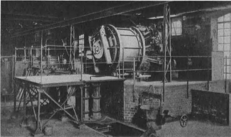
Abb. 6. Drehstrom-Rollofen.
