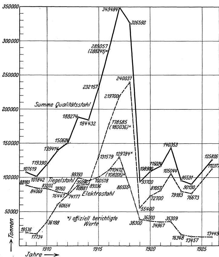
Abb. 53. Verdrängung der Tiegelstahlproduktion durch Elektro Stahl in Deutschland und Luxemburg.
