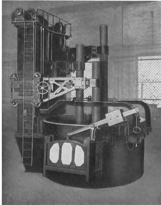
Abb. 64. 7 t-Drehstromlichtbogenofen mit abgedichteten Elektroden, System Siemens & Halske A. G.
