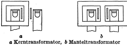
a Kerntransformator, b Manteltransformator
