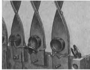
Abb. 7. Messung des Stromes in Kupferschienen unter Verwendung des Spannungsabfalles. Kompensationsspulen zum Ausgleich des Anwärmefehlers.
