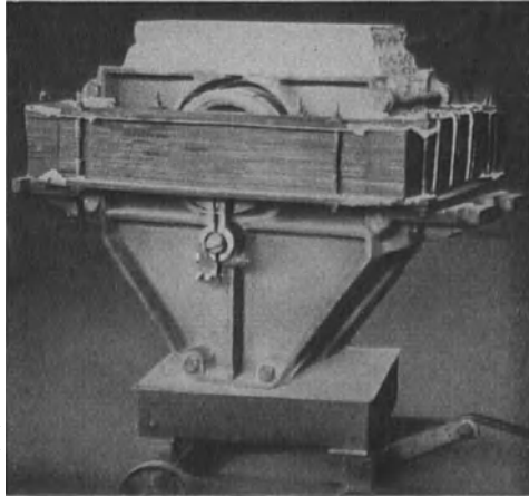
Abb. 17. Bodenstein, Spule und Transformatorkörper zum Einbau vorbereitet (Ajax-Wyatt-Ofen).
