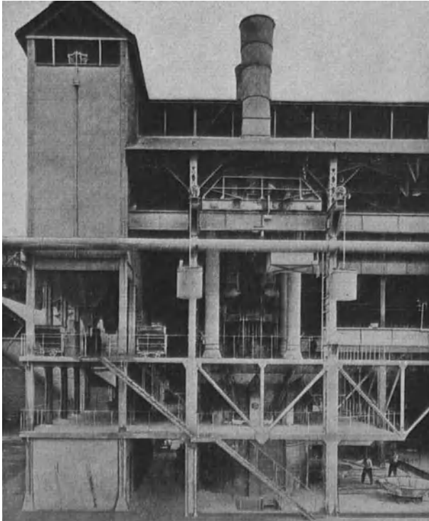
Abb. 1. Einphasenkarbidofen, System Miguet.
