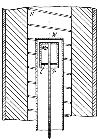
Abb. 29. Anordnung zur Messung des Elektronentransportes bei hohen Temperaturen.
