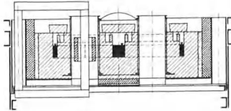
Abb. 9. Induktionsofen nach Röchling-Rodenhauser.
