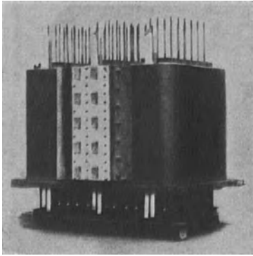
Abb. 9. Drehstromtransformator mit Umlaufwasserkühlung mit abgenommenem oberen Joch.
