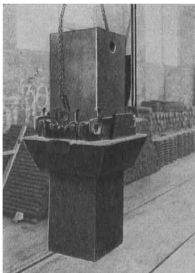
Abb. 36. Elektrode mit Rutschfassung.
