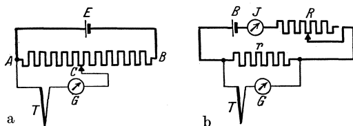
Abb. 35. Messung der EMK von Thermoelementen.
