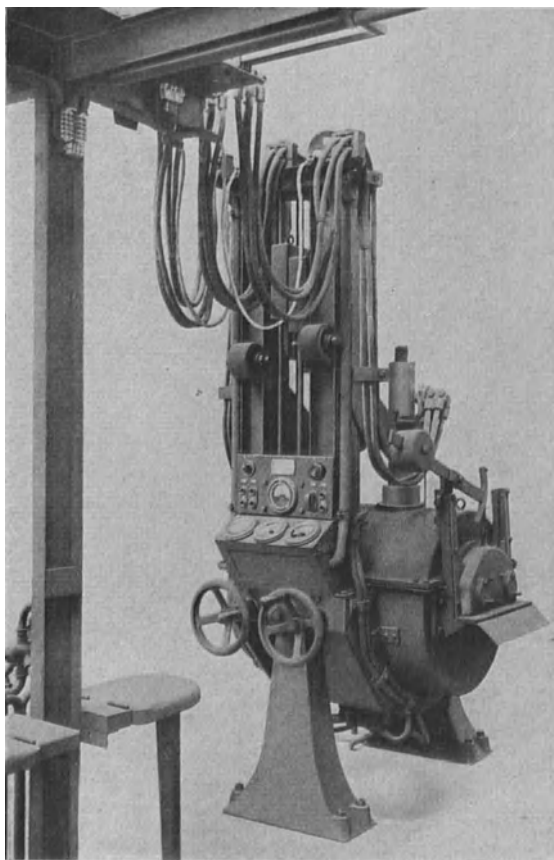
Abb. 8. BBC-Lichtbogenofen zum Schmelzen von Nickel.
