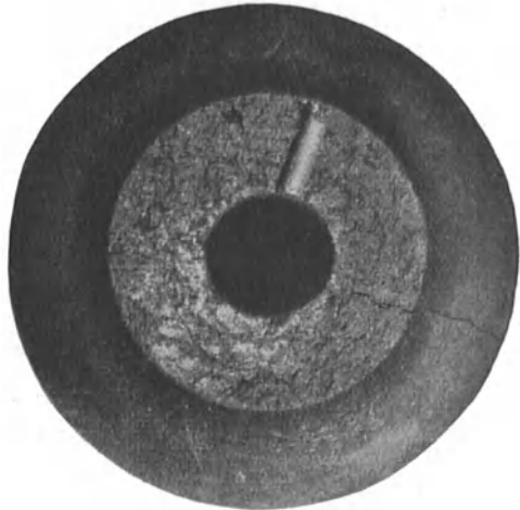
Abb. 28. Bohrkanal mit geschmolzenem Graphit gefüllt.
