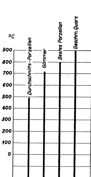
Abb. 19. Verschiedene Isolierstoffe bei gleichem Widerstand 1 mg-Ohm per \text{cm}^3 .
