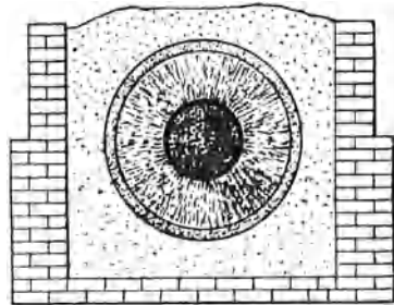
Abb. 5. Querschnitt durch einen Siliziumkarbid-Ofen.
