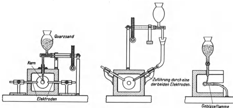
Abb. 16. Lichtbogenofen vom Silica Syndicate Ltd. London. D. R. P. 241260.
