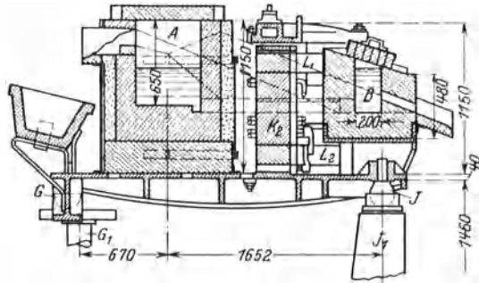
Abb. 10. Induktionsöfen nach Schneider-Creusot (senkrechter Schnitt).
