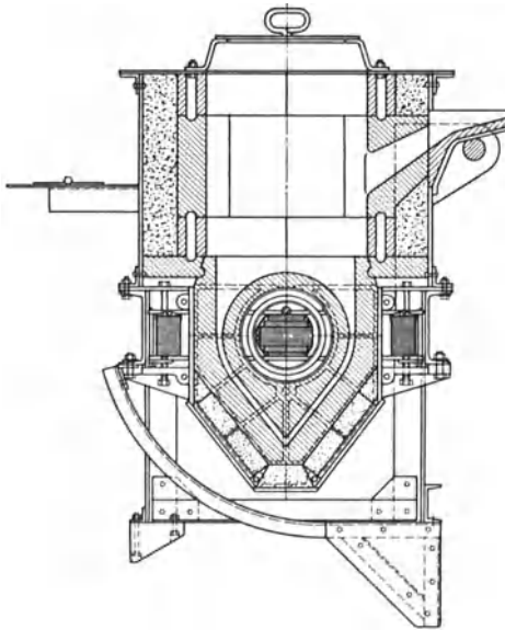
Abb. 13. Einphasen-Induktionsofen, System Ajax-Wyatt.
