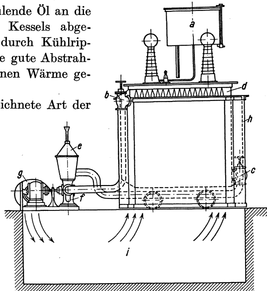
Abb. 3. Kühlung durch künstliche Luft und Ölumlauf (innerer Ölumlauf).
