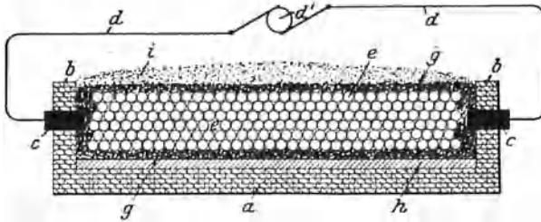
Abb. 1. Graphitierung von Elektrodenstäben.
