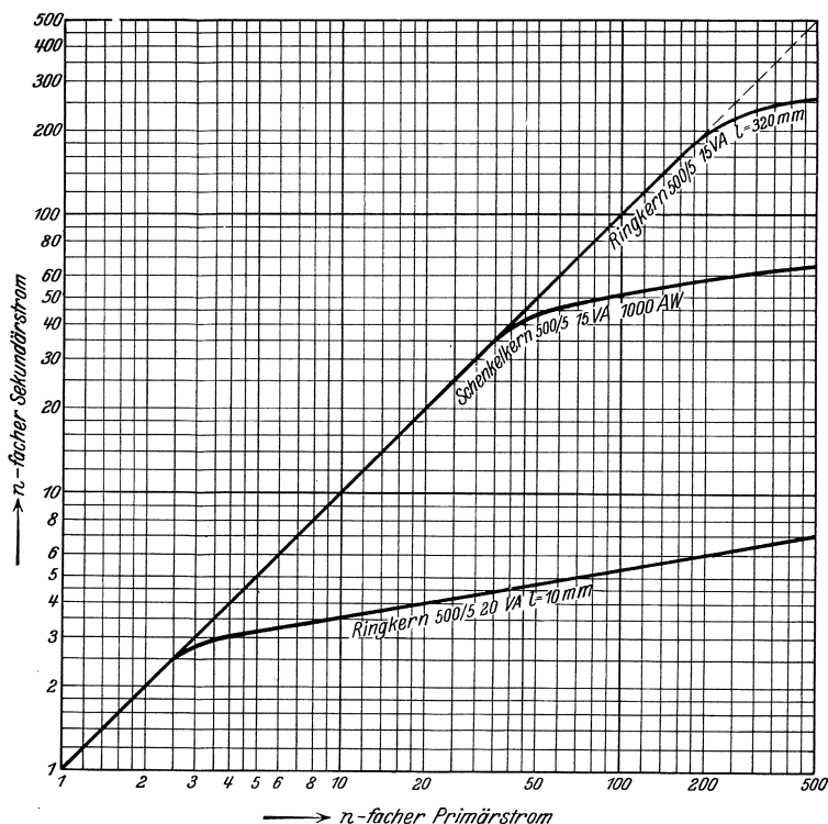
Abb. 15. Verhalten dreier verschiedener Stromwandler bei Überstrom. Der Ringkern mit 10 mm hoher Eisenpackung fällt schon beim 3fachen Primär-Nennstrom ab, der mit 320 mm langem Kern erst beim 200fachen Strom.
