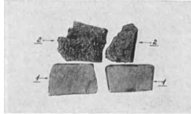
Abb. 68. Gußproben aus Elektroofen (1) und Kupolofen (2).
