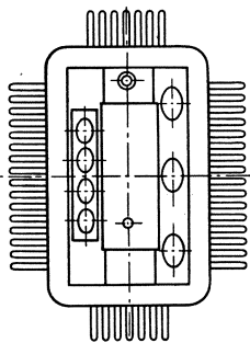
Abb. 1. Selbstkühlung im Wellblechkessel.
