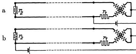
Abb. 30a. Temperaturmessung mit Widerstandsthermometern und Kreuzspul-Instrumenten.
