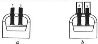
Abb. 26c. Indirekte Lichtbogenheizung.
