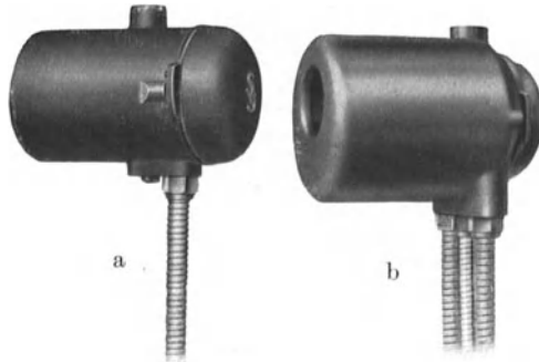
Abb. 54. Betriebs-Bauformen des Siemens-Ardometers. a Normale Ausführung, b Ausführung mit Wasserkühlung.
