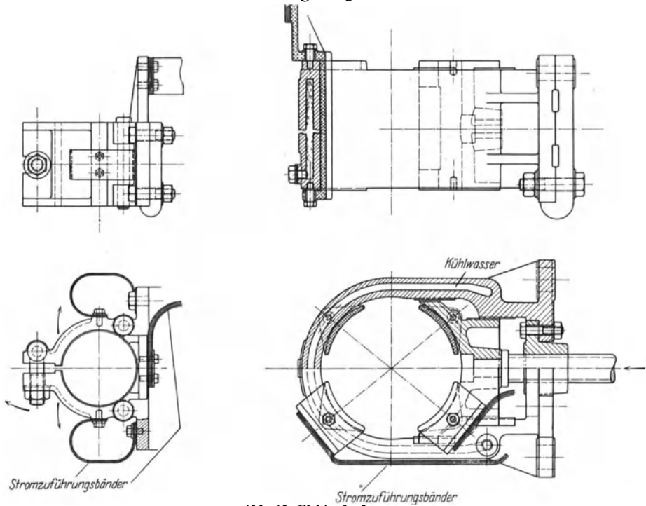
Abb. 46. Elektrodenfassung.
