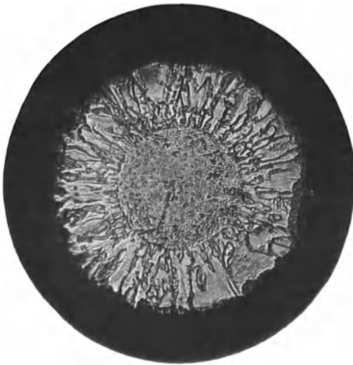
Abb. 21. Querschliff eines feinkristallinen Anwachskristalles.
