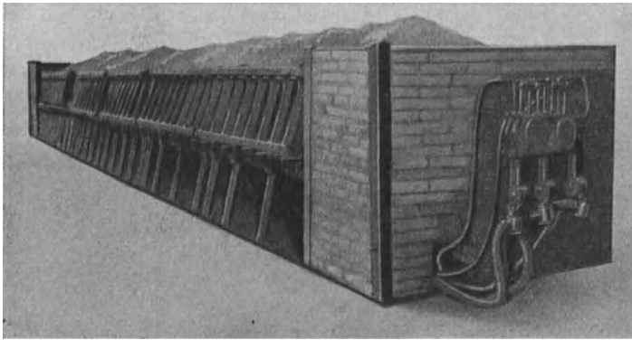
Abb. 3. Transportable Seitenwände eines Siliziumkarbid-Ofens.
