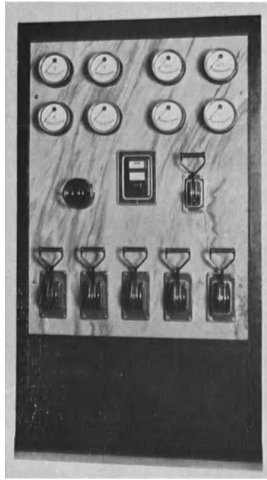
Abb. 74. Schaltanlage, System Siemens & Halske A.G.
