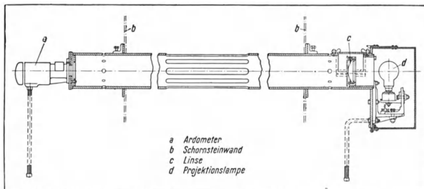
Abb. 57. Rauchdichteanzeiger. Schematische Darstellung der Meßanordnung.
