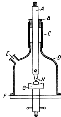
Abb. 15. Lichtbogenofen. A Elektrode, wassergekühlt, B Gummistopfen, C Gummischlauch, D Kupferglocke, E Schauloch, F Gummidichtung, G Nickelpfanne, H Tantal.
