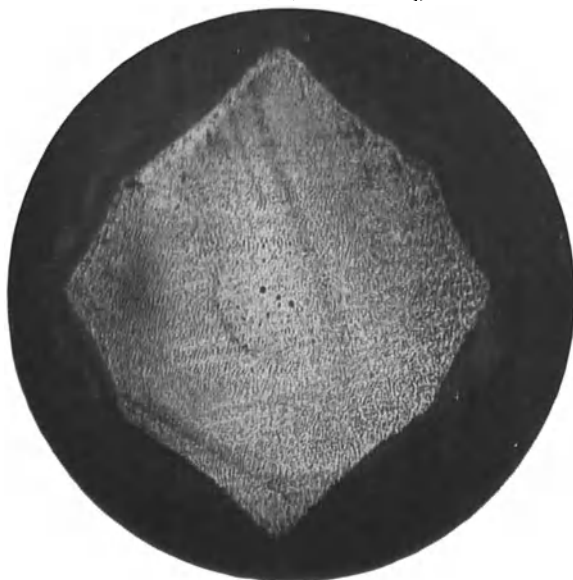
Abb. 22. Querschnitt durch einen aus der Gasphase gewachsenen abgeätzten Einkristall.
