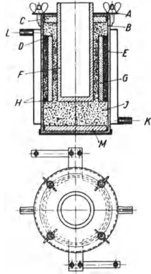
Abb. 6a. Wassergekühlter Kohlekörnerofen der Auergesellschaft.
