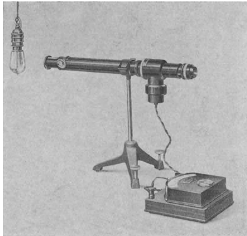
Abb. 63. Mikro-Glühfadenpyrometer zur Temperaturmessung an Leuchtfläden.
