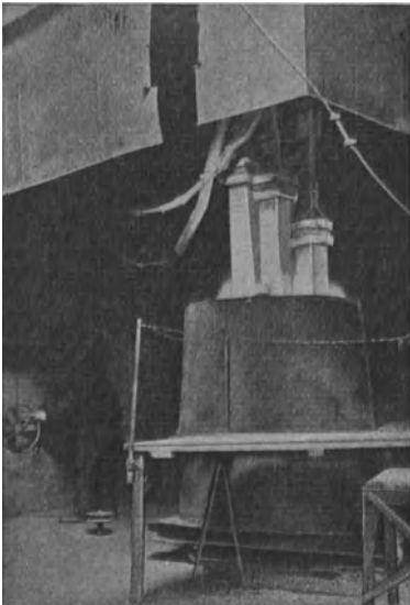
Abb. 6. Korundofen in Betrieb.
