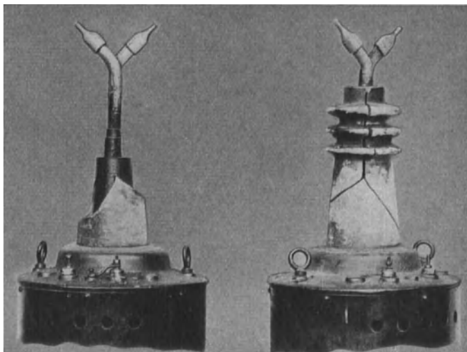
Abb. 18. Zwei dynamisch zerstörte Topf-Stromwandler: Isolatoren durch Auseinanderschlagen der Primärleiter zertrümmert.
