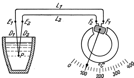
Abb. 32. Schema der Temperaturmessung mit einem Thermolement.
