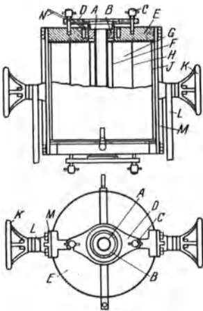
Abb. 7. Nernst-Tammann-Ofen des Elektroschaltwerks.
