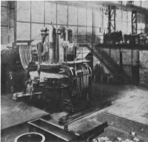
Abb. 63. 8 t-Drehstromlichtbogenofen mit abgedichteten Elektroden, System Siemens & Halske A.G.
