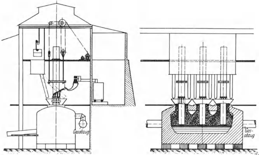
Abb. 57. Schema einer Niederschachtroheisen-Elektroofenanlage.
