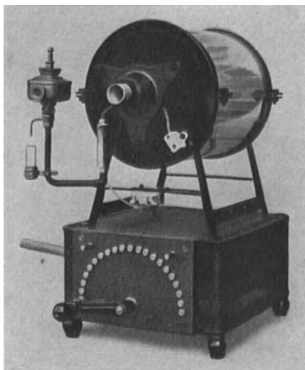
Abb. 2. Molybdändrahtofen mit Regulatorwiderstand.
