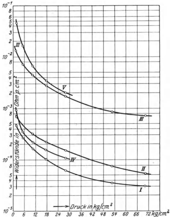
Abb. 4. Übergangswiderstände in Ohm/cm 2 bei verschiedenen Auflagedrücken für I Graphit auf Graphit, II Graphit auf Kupfer, III Graphit auf Stahl, IV Graphit auf Messing, V Graphit auf Aluminium.
