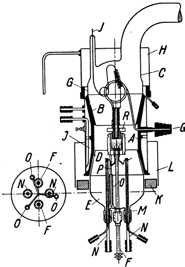
Abb. 13. Hochvakuumofen.
