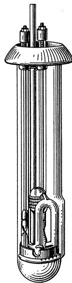
Abb. 30. Quecksilberdampflampe zum Eintauchen in Flüssigkeiten (A. Jaenicke).
