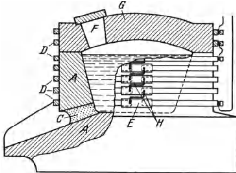
Abb. 22. Hochfrequenzofen.
