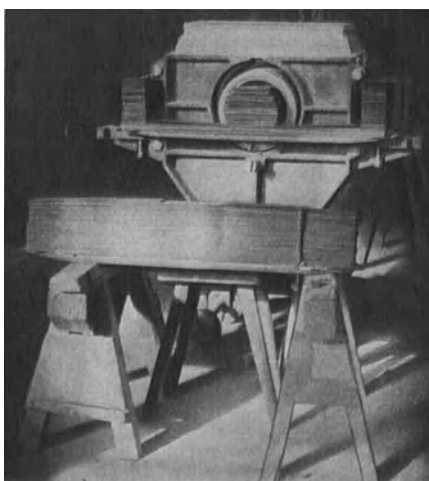
Abb. 16. Transformatorkörper mit abgenommenem Joch (Ajax-Wyatt-Ofen).
