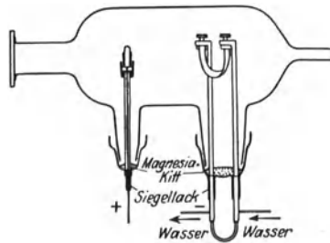
Abb. 8. Vakuumschmelzapparat mit Glühkathode.
