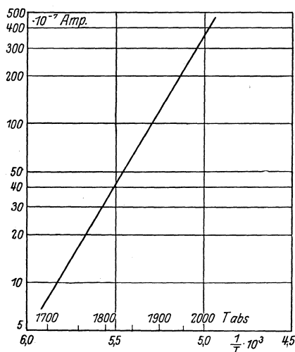
Abb. 30. Zusammenhang zwischen Stromstärke und Temperatur im Wasserstoff.
