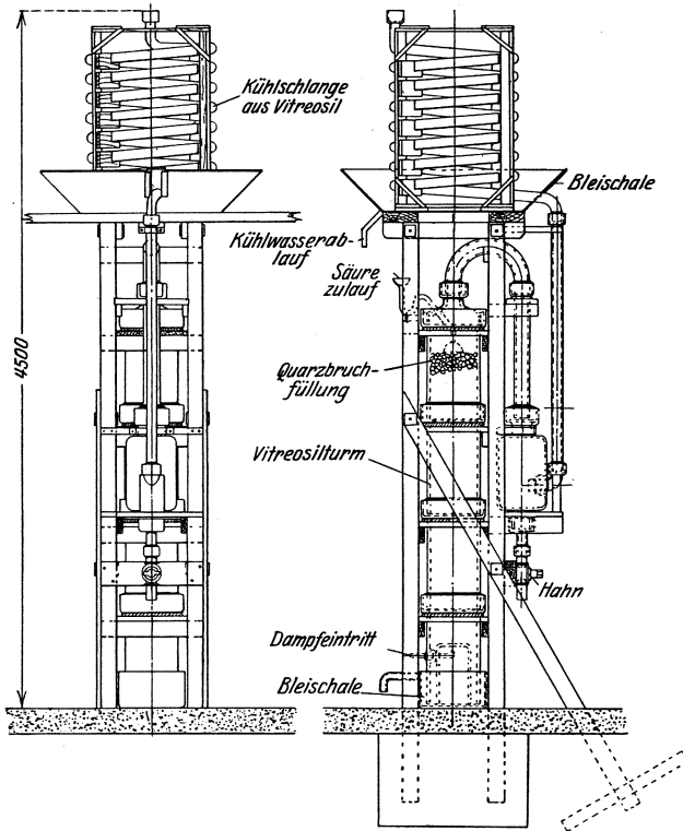
Abb. 26. Denitrieranlage.
