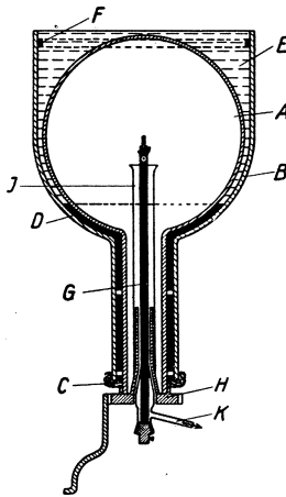
Abb. 9. Kathodenstrahl-ofen.
