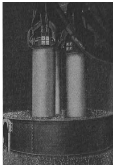
Abb. 8. Korundofen nach vollendeter Füllung.
