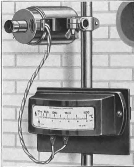
Abb. 51. Das „Pyrradio“ von Hartmann & Braun. Temperaturkompensation durch eine von einem Bimetallstreifen Bm bewegte Blende.
