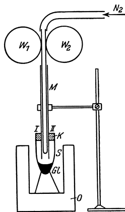
Abb. 18. Vorrichtung zum Züchten eines Metalkristalles aus der Schmelze.
