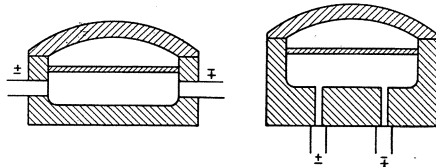
Abb. 48. Direkte Widerstandsöfenheizung.
