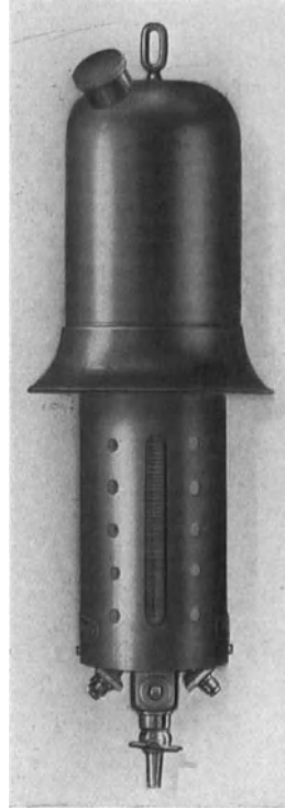
Abb. 41. Feuchtigkeitsmesser nach dem Psychrometerprinzip (Keiser & Schmidt).
