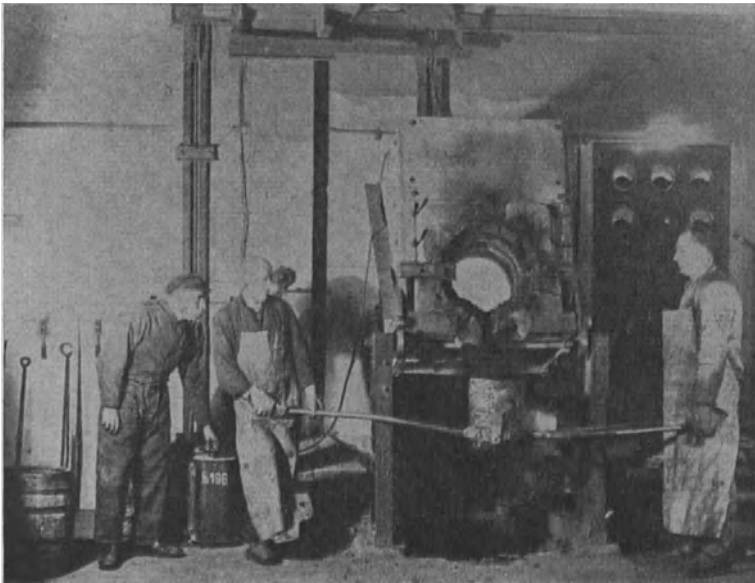
Abb. 26. 100 kW-Hochfrequenzofen, System Ajax-Northrup, während des Gießens.
