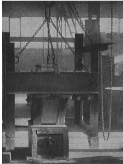
Abb. 18. Traggestell während der Montage (Ajax-Wyatt-Ofen).
