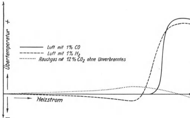
Abb. 26. Einfluß von Wärmeleitfähigkeit und katalytischer Verbrennung auf die Drahttemperatur.
