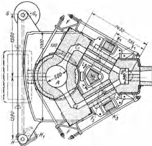
Abb. 11. Induktionsofen nach Schneider-Creusot (wagerechter Schnitt).
