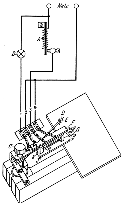
Abb. 44. Schema und Ausführung eines Pyrometeranzeigeeinstrumentes mit Maximal- und Minimalkontakt. Auch hier wird der Fallbügel durch einen Bimetall-Motor ausgelöst (Keiser & Schmidt).
