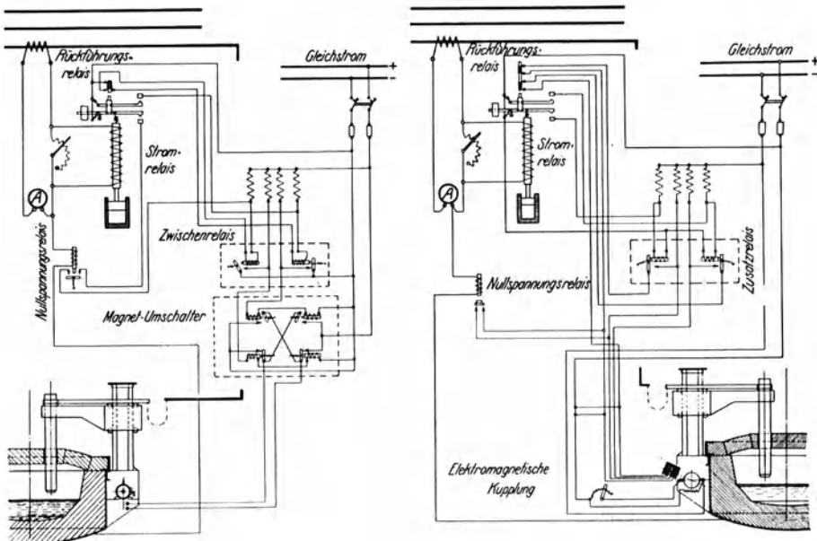
Abb. 44. Automatische Elektrodenregulierung, System Fuss.
