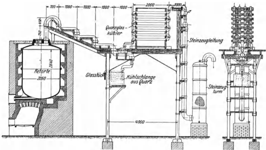
Abb. 25. Salpetersäureanlage.
