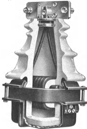
Abb. 13. Querloch-Topf-Stromwandler mit Porzellan-Isolierung.
