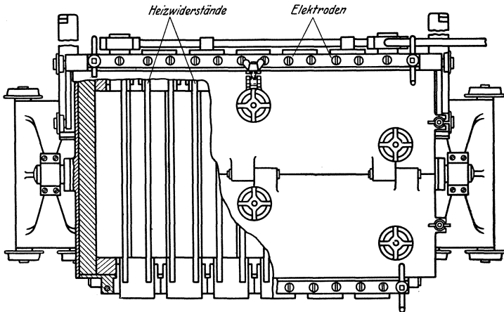
Abb. 9a. Erschmelzen flächenhafter Gegenstände. D.R.P. 445763.
