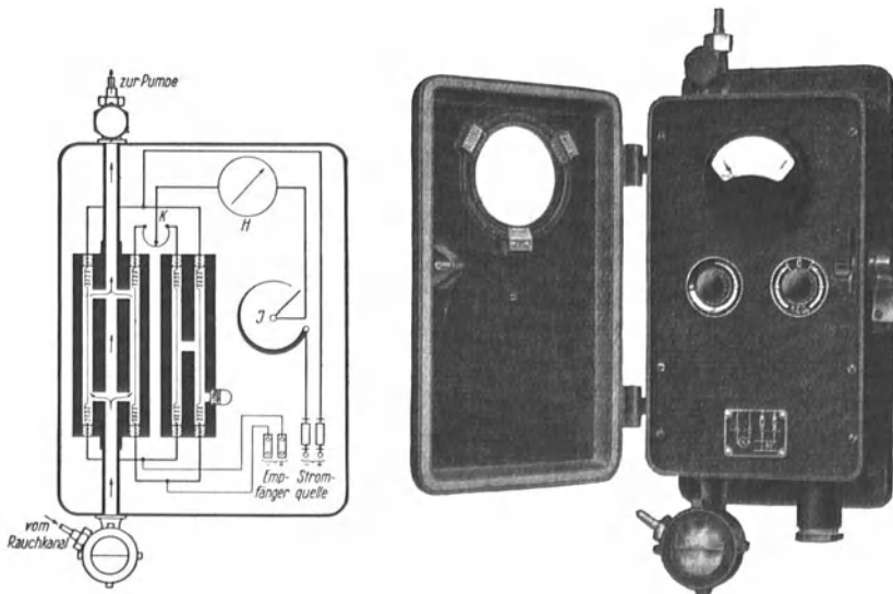
Abb. 25. Gaslauf und Innenschaltung, Außenbild des Gebers für einen \text{CO}_2 -Messers (Siemens & Halske).
