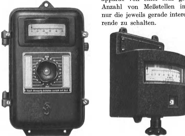
Abb. 39. Anzeigeeinstrumente mit eingebautem Drehschalter zur Vielfach-Messung (Siemens & Halske, Dr. R. Hase).
