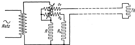
Abb. 31. Temperaturmessung mit Widerstands-Thermometer, Wechselstrom und Doppelspul-Instrumente.
