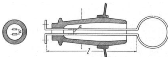
Abb. 17. Schema der Leitungseinführung in einen Topf-Stromwandler.
