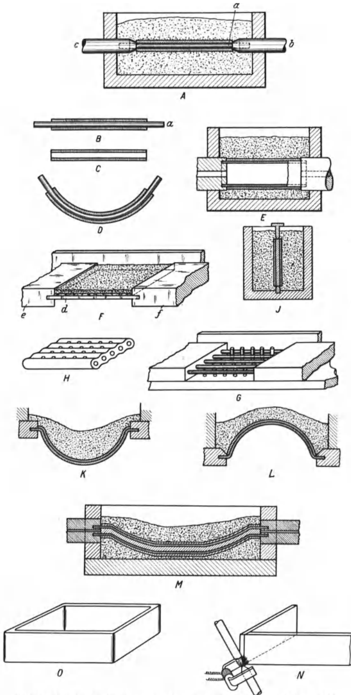
Abb. 5, A bis O. Erschmelzung von Quarz nach E. Thomson. A. P. 778286.
