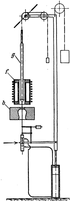
Abb. 14. Schema einer Gasglocken-Blasemaschine
