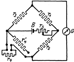
Abb. 30. Grundsaltung für die Temperaturmessung mit Widerstands-Thermometer in Brückenschaltung.
