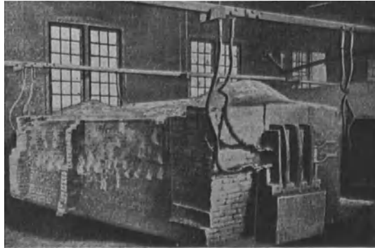
Abb. 4. Siliziumkarbid-Ofen während des Betriebes.
