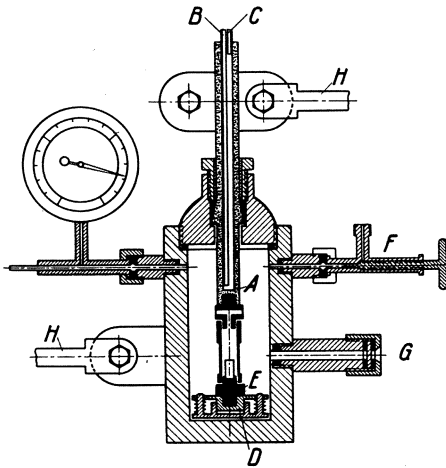
Abb. 17. Druckofen.
