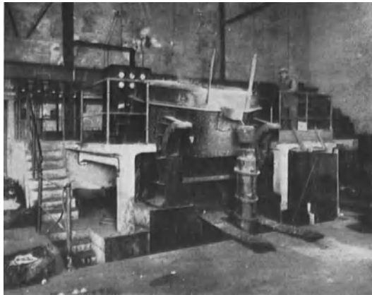
Abb. 69. Induktionsofen für Nichtisenmetalle, System Siemens & Halske, 712 kg Abstichgewicht.
