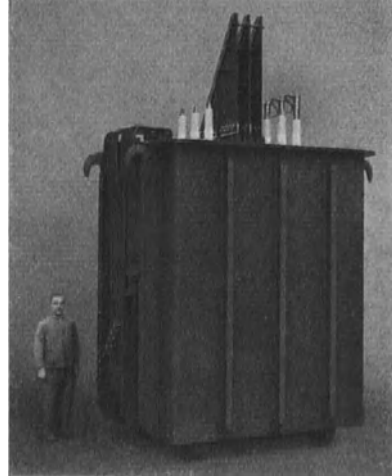
Abb. 7. Öltransformator mit innerer Wasserkühlung.
