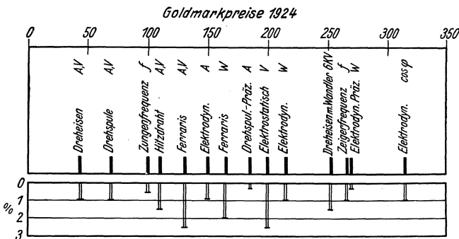
Abb. 1. Ungefährer Preis und Genauigkeit elektrischer Zeiger-Meßgeräte.
