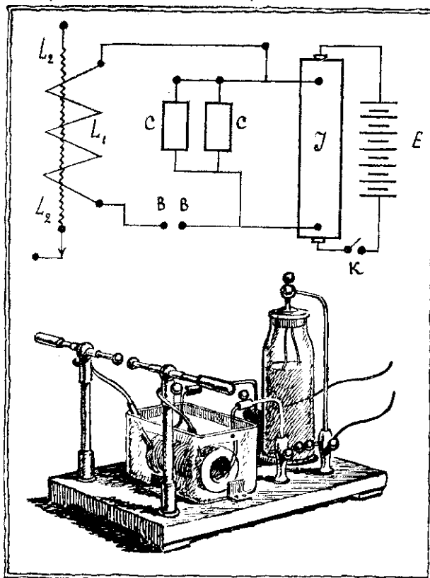
Резонанс-трансформатор Теслы: E — батарея или другой источник тока. J — индукционная катушка. BB — искровой разрядник. CC — батарея лейденских банок. L 1 — первичная катушка трансформатора. L 2 — вторичная катушка трансформатора, K — механический прерыватель. На нижнем рисунке катушки L 1 и L 2 погружены в масло.
