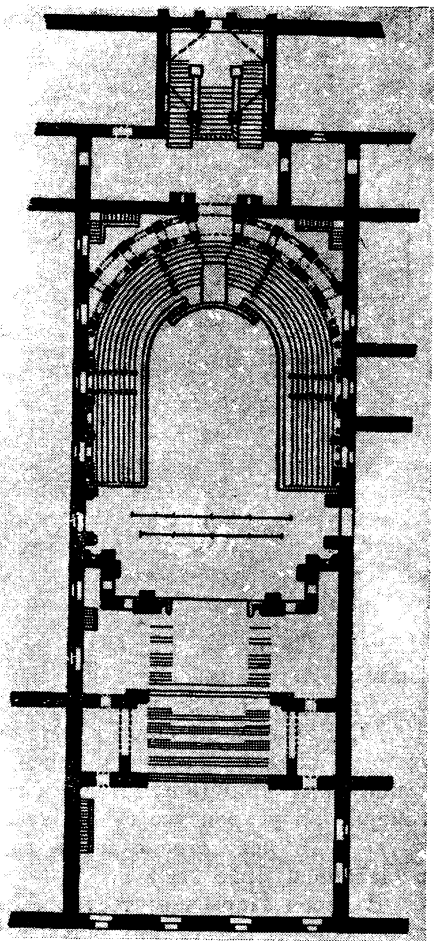
План театра Фарнезе в Парме Архитектор Дж. Алеотти. 1619 г.
