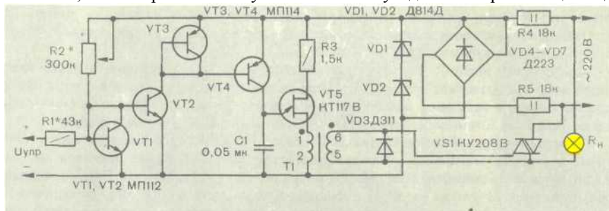
Рис. 49. Схема блока усиления мощности СМН
