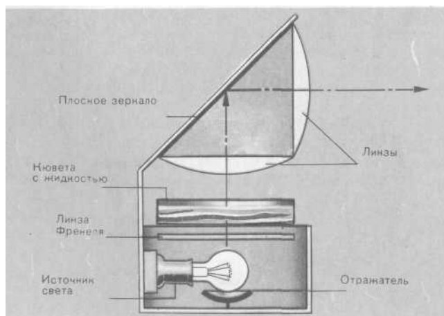
Рис. 18. Схема диапроектора с поворотом луча
