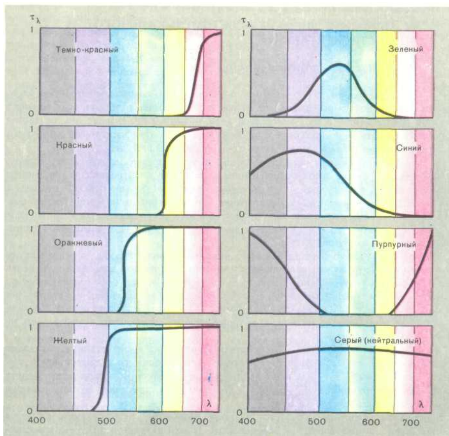
Рис. 11. Характеристики пропускания набора цветных стеклянных фильтров
