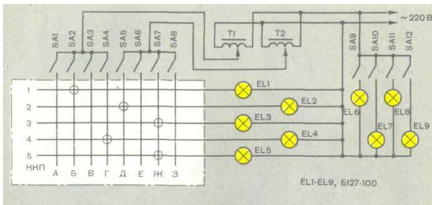
Рис. 37. Схема СМИ "Харьков"
