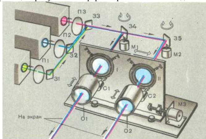
Рис 71. Принцип действия многоцветного ЛСМИ
