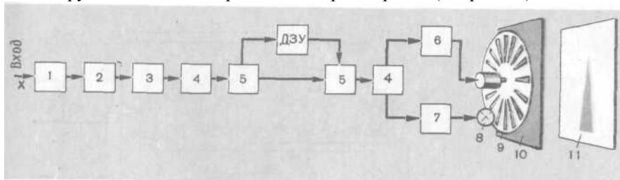
Рис. 81. Структурная схема канала управления СМИ МИСС-2
