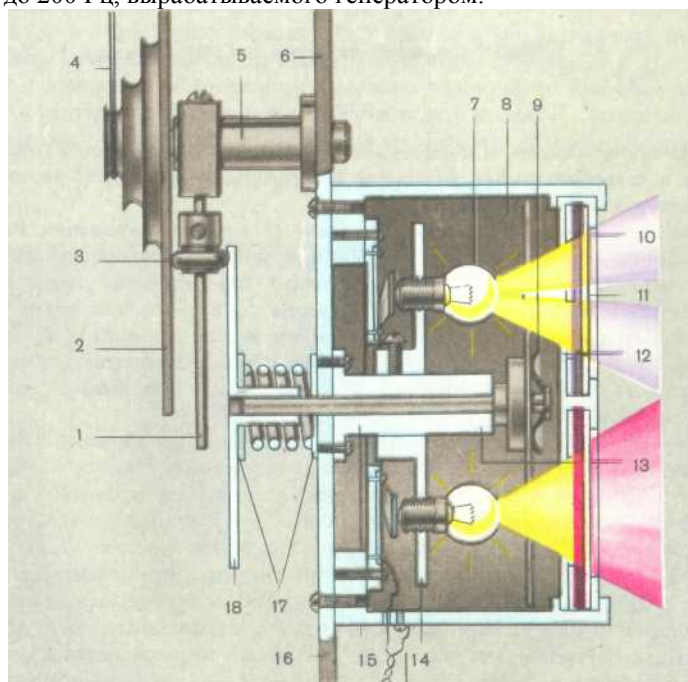
Рис 44. Проекционная ячейка СМИ "Полтава"
