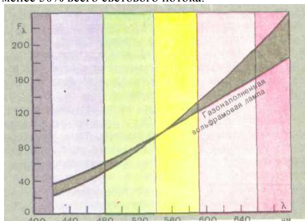
Рис. 13. Распределение энергии излучения в спектре семейства газонаполненных ламп накаливания
