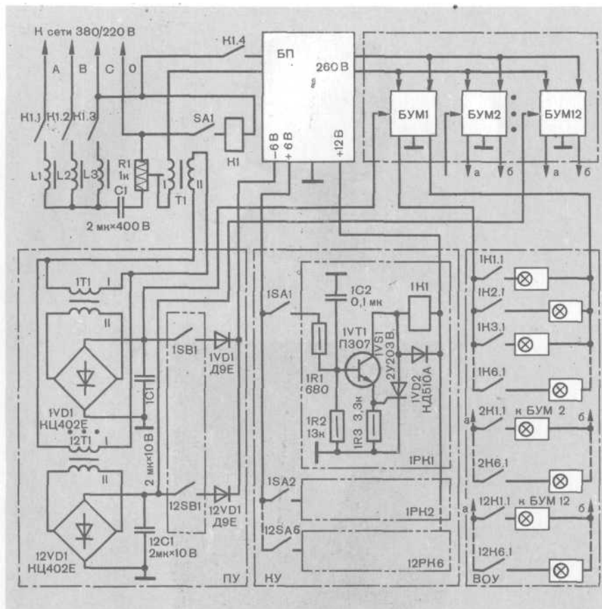
Рис. 66. Принципиальная схема одного сквозного канала управления СМИ "Прометей-3"
