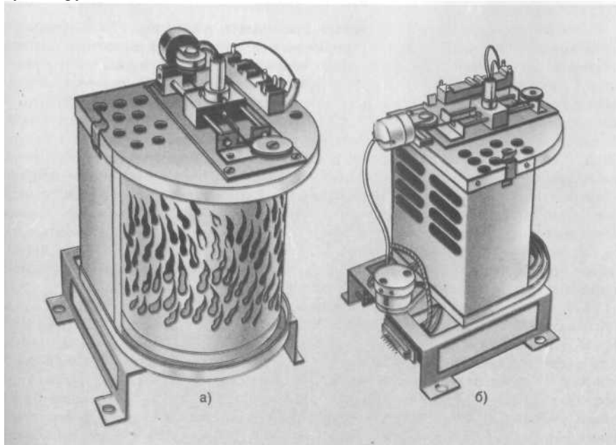
Рис. 48. Проекционная ячейка СМИ "Полтава-2"
