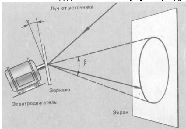
Рис. 74. Развертка луча по окружности
