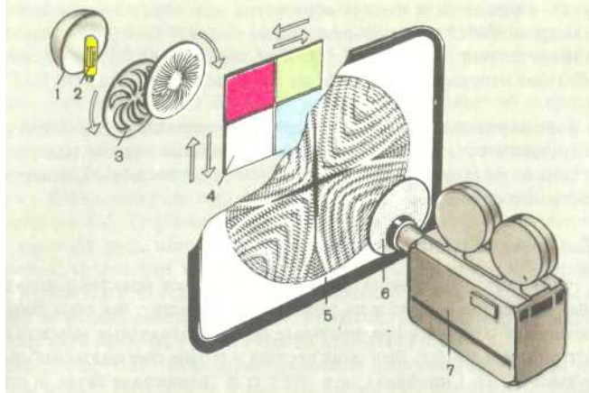
Рис. 84. Схема аппаратуры для съемки светомузыкальных фильмов
