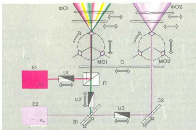
Рис. 70. Сценический ЛСМИ фирмы "Сименс"
