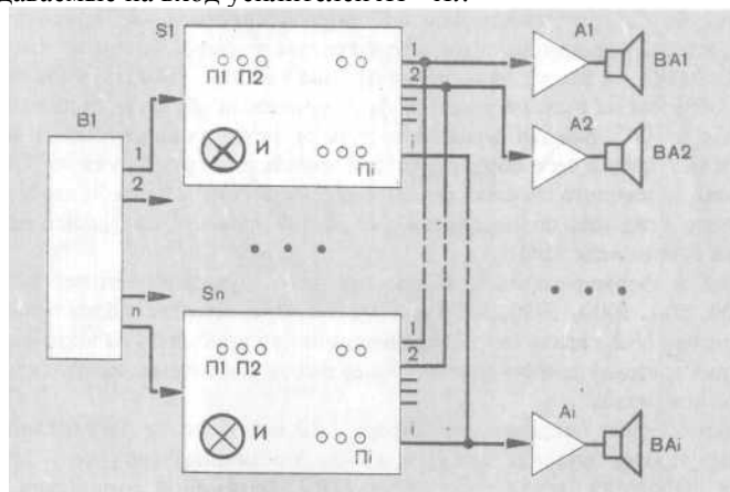
Рис. 77. Обобщенная структурная схема установки "пространственной музыки"
