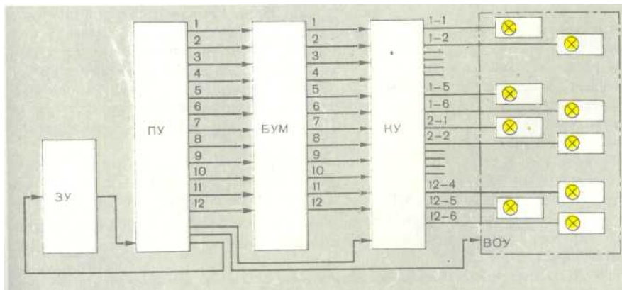
Рис. 57. Структурная схема СМИ "Прометей-3"
