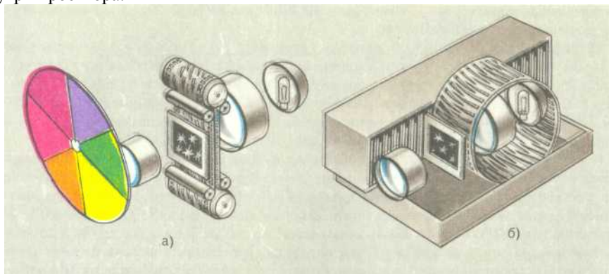
Рис. 55. Светозффектные устройства на базе слайдпроекторов: а — с кольцевой пленкой (конструктор С. М. Зорин); б — с автоматической сменой статоров (конструкция СКБ "Прометей")
