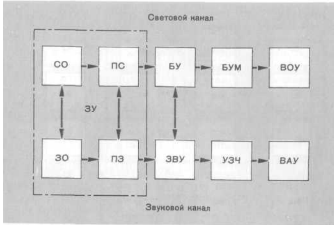
Рис. 8. Структурная схема аудиовизуального инструментария
