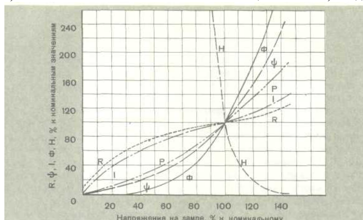
Рис. 12. Зависимость основных параметров лампы накаливания от напряжения
