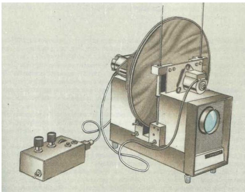
Рис. 59. Светозффектный проектор с двумя дисковыми роторами
