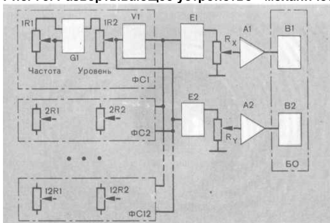
Рис. 76. Функциональная схема пульта управления ЛСМИ
