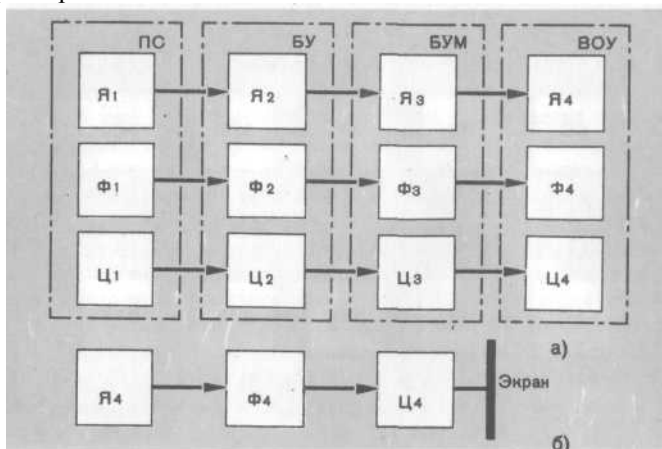
Рис. 9. Структурная схема светового канала (а) и вариант расположения элементов в ВОУ (б)
