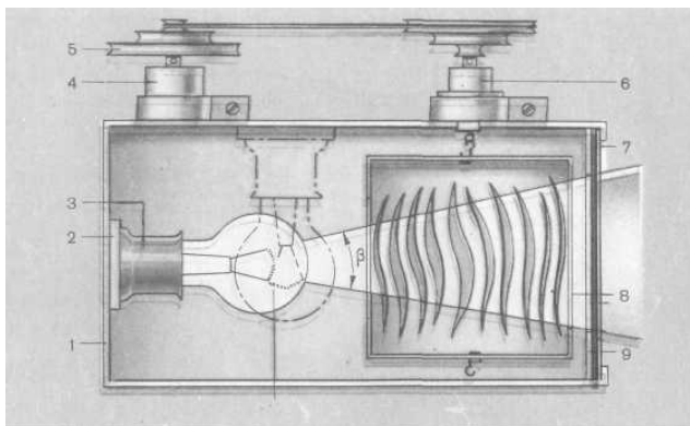
Рис 40. Формообразующая проекционная ячейка СМИ "Харьков"
