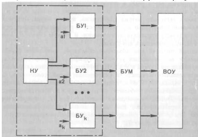
Рис. 10. Многоканальный светомузыкальный инструмент проекционного типа
