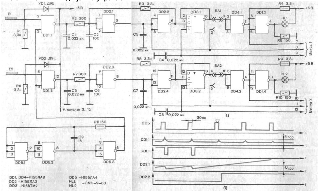
Рис 68. Принципиальная схема сенсорного переключателя
