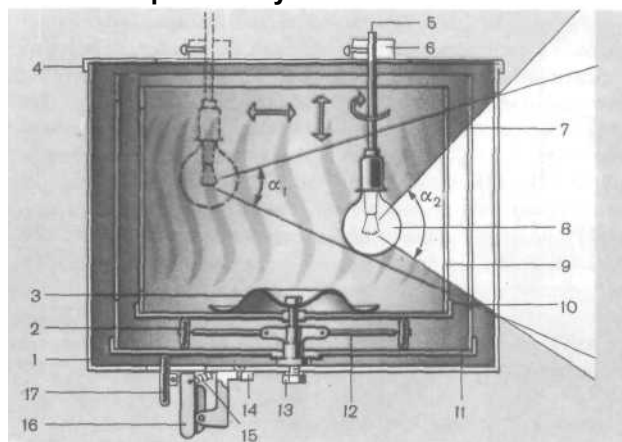
Рис. 47. Формообразующая проекционная ячейка с двойным барабаном
