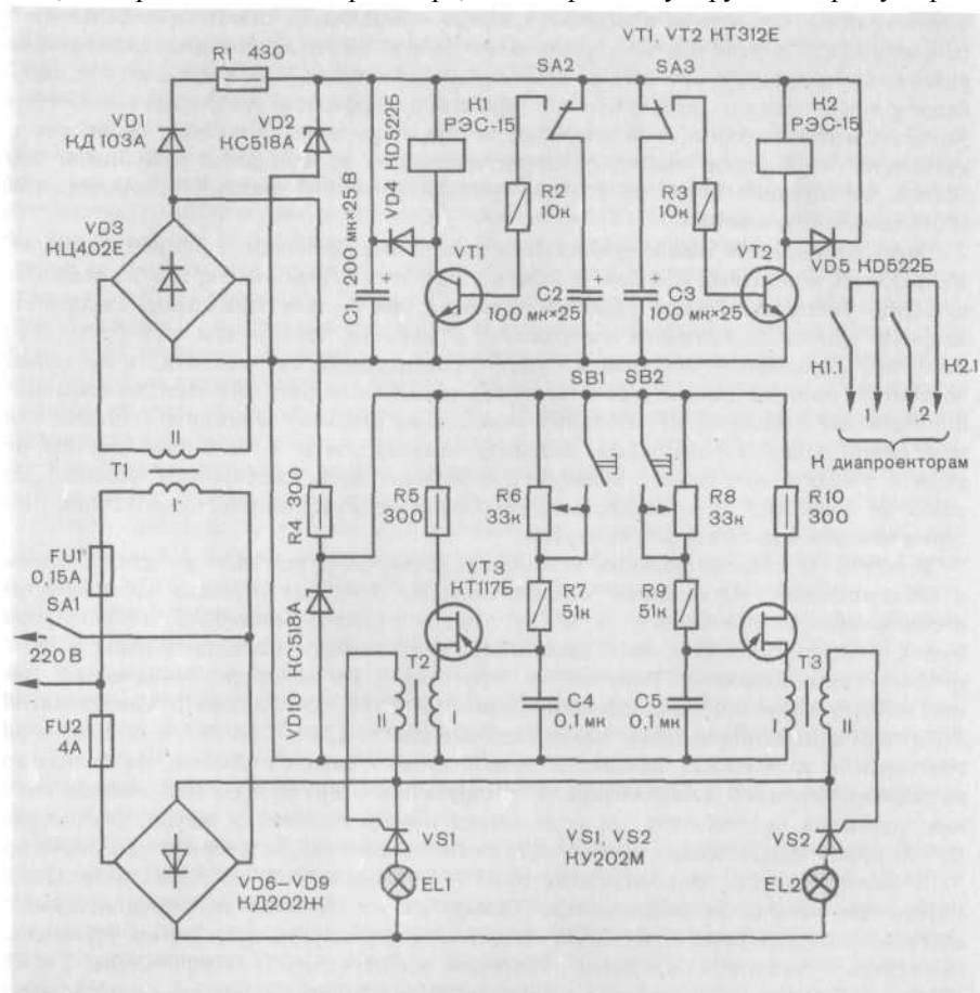
Рис. 54. Принципиальная схема пульта для управления диапроекторами
