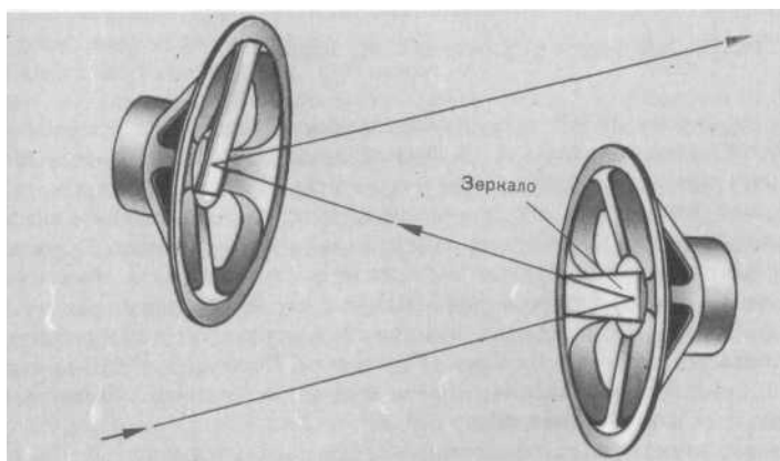
Рис. 75. Развертывающее устройство - механический осциллограф
