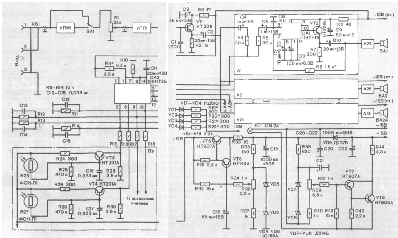
Рис. 79. Принципиальная схема канала управления движением звука
