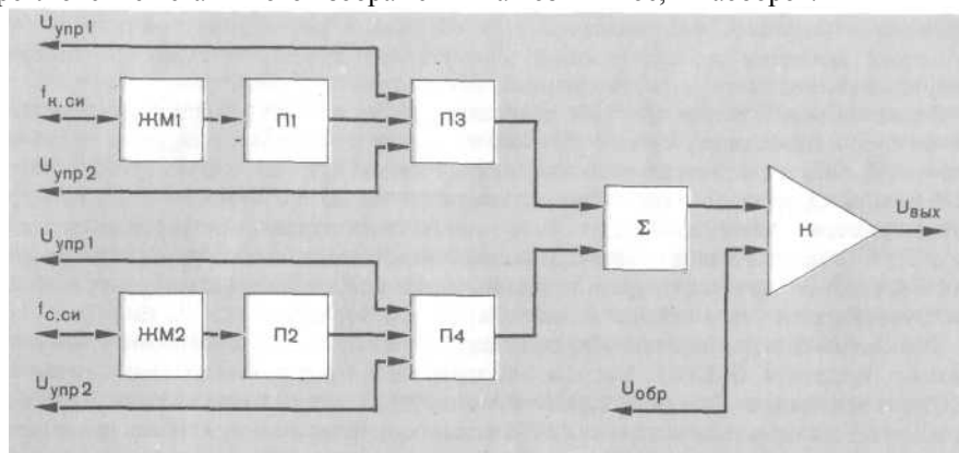
Рис. 89. Структурная схема ГФН
