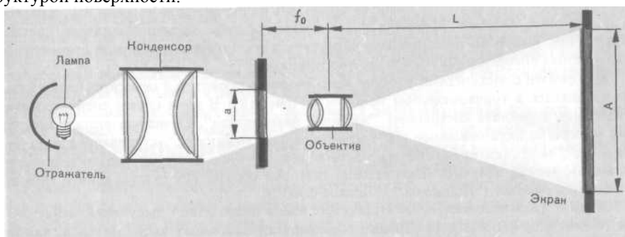
Рис. 16. Схема диапроекции
