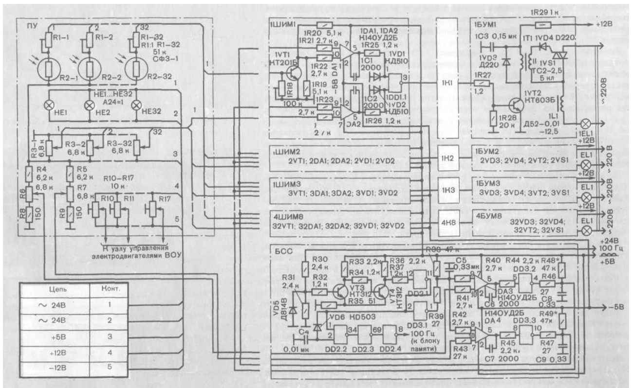
Рис. 83. Принципиальная схема СМИ "Мираж" (без системы записи)
