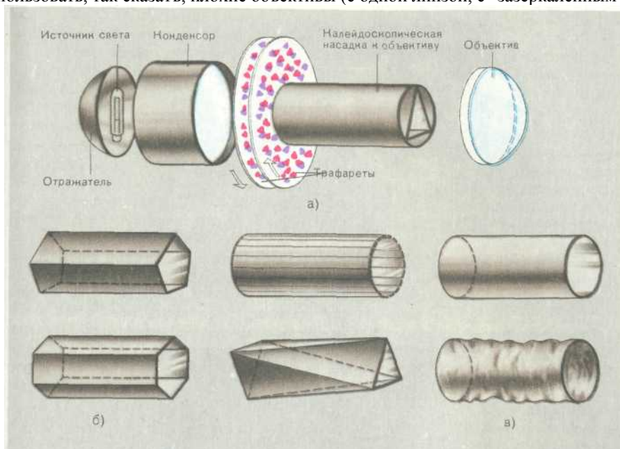
Рис. 61. Принцип действия "Калейдофона" (а) и исполнение калейдоскопических (б) и деформирующих (в) насадок
