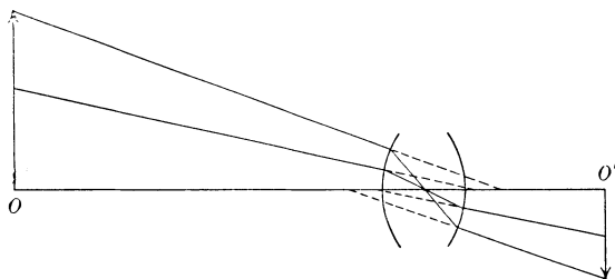
Fig. 31. Schema für den Gang der Hauptstrahlen bei einem holosymmetrischen Objektiv mit unkorrigierten Pupillen.
