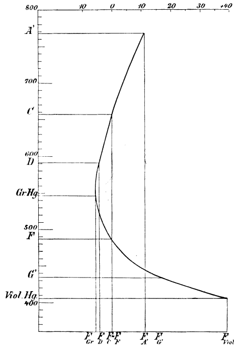
Fig. 34. Sekundäres Spektrum der Kombination O. 1726, O. 108. Optische Korrektion f_C = f_F = 100 mm. Die Ordinaten ergeben die Wellenlängen in \mu\mu . Die Abscissen ergeben f_\lambda - f_C in hundertel Millimeter, abgetragen von F_C = F_F .
