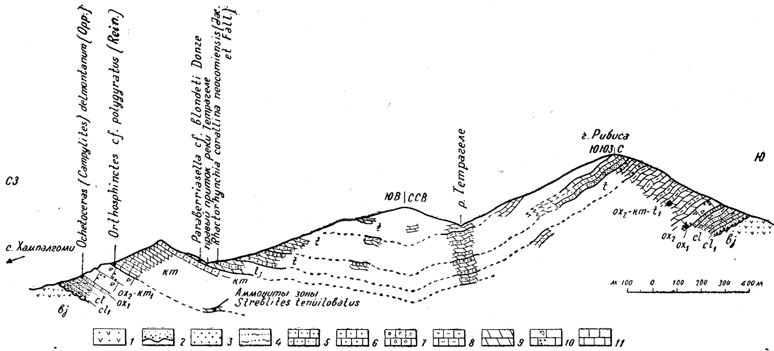
Рис. 2. Разрез Рибисской синклинали
