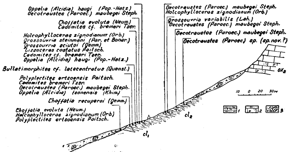
Рис. 5. Разрез в окрестностях кладбища с. Цона
