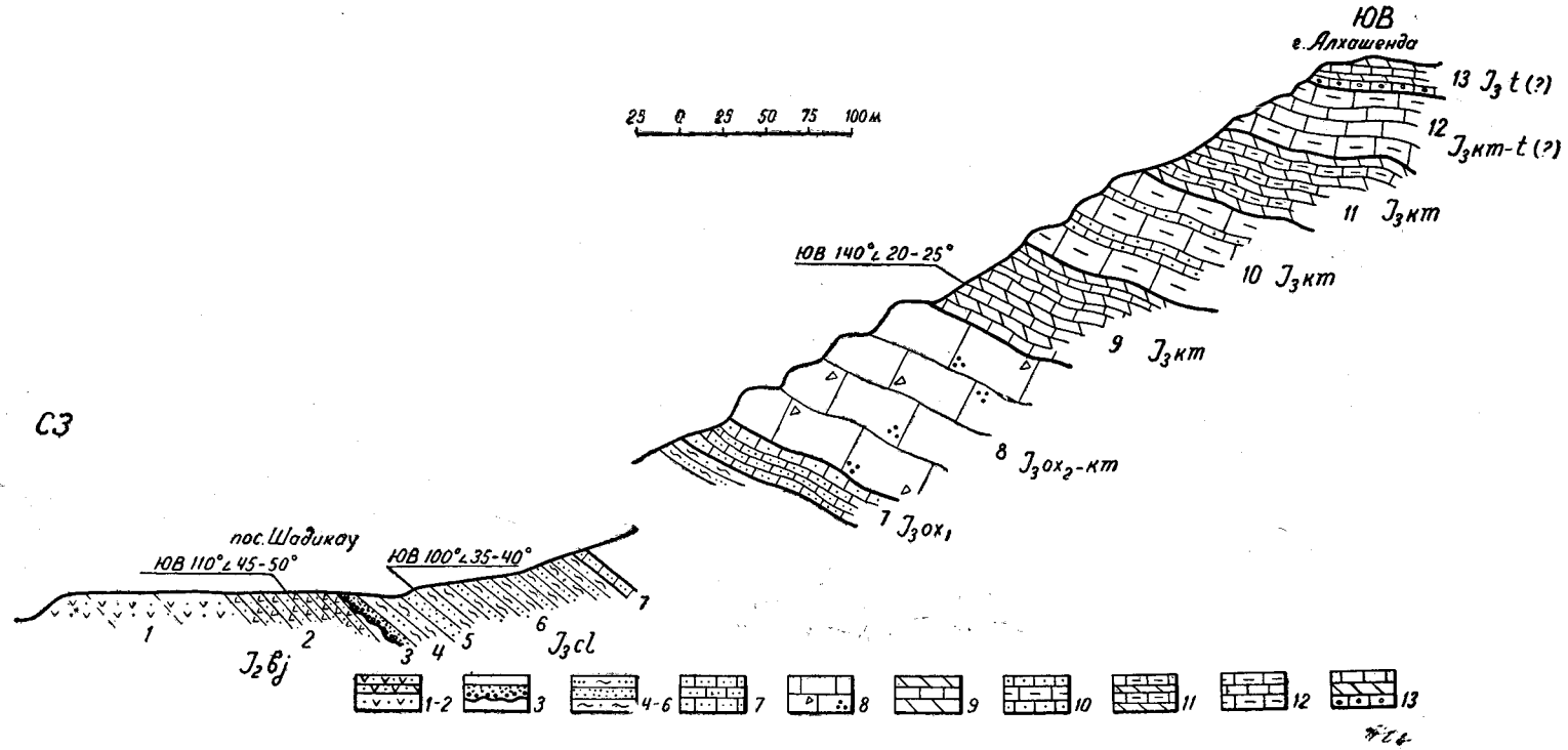
Рис. 3. Разрез с. Шадикау — г. Алхашенда.
