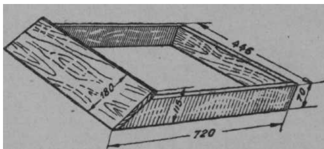
РИС. 17. Подставка под улей.
