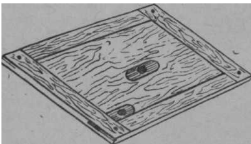
РИС. 41. Потолок в два удалителя пчел. Через угловой пчелы выходят наружу, через средний — в гнездо.
