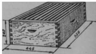
РИС. 3. Корпус улья.
