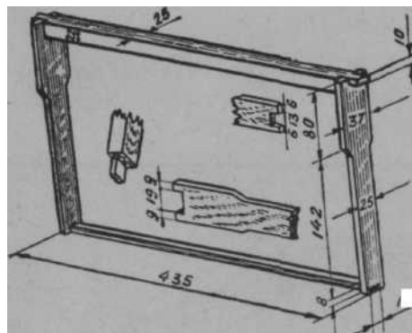
РИС. 15. Рамка с постоянными разделителями Гофмана.
