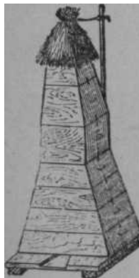
РИС. 1. Улей Витвицкого последнее» образца. Он имеет только один леток (в дне), В задних стенках надставок просверлены отверстия для вентиляции, которые открываются в жаркую погоду и во время взятков.
