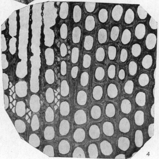
Acanthocladia , Archimedes
