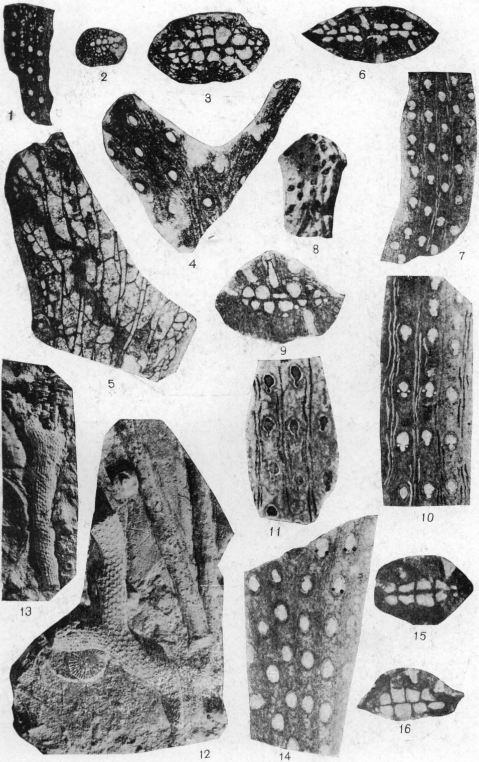
Sulcoretepora
