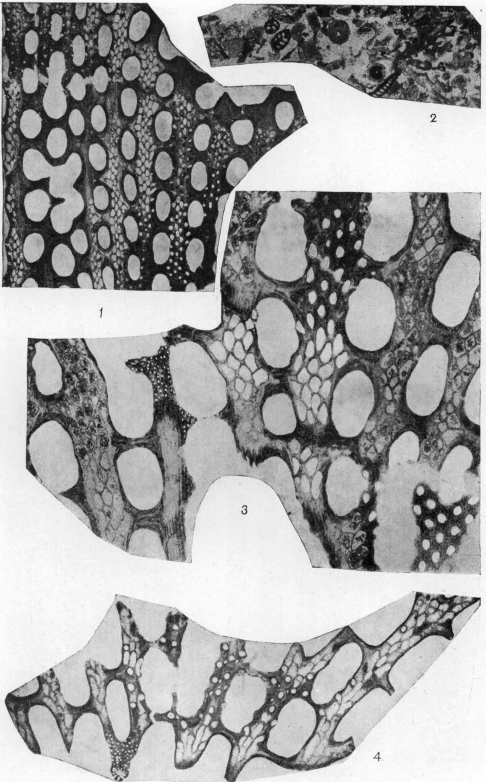
Polypora
