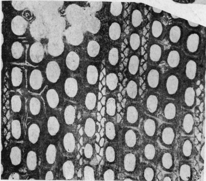
Fenestella, Nematopora
