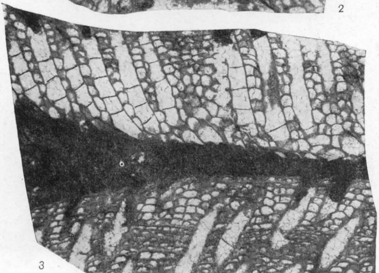
Fistulipora
