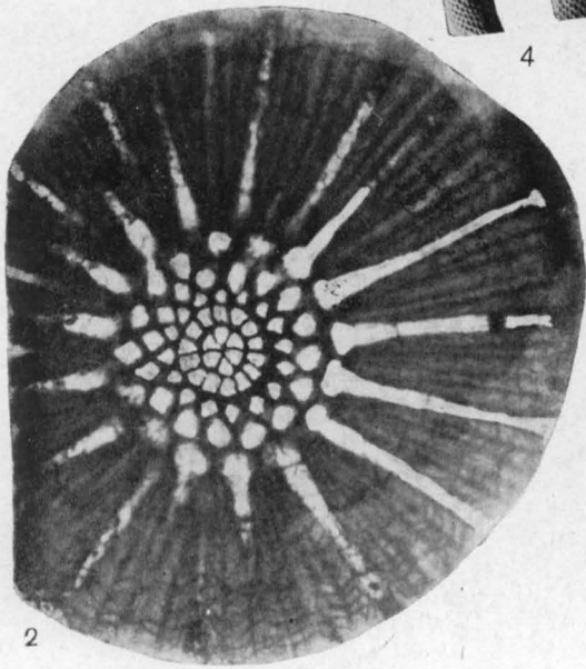
Ascopora
