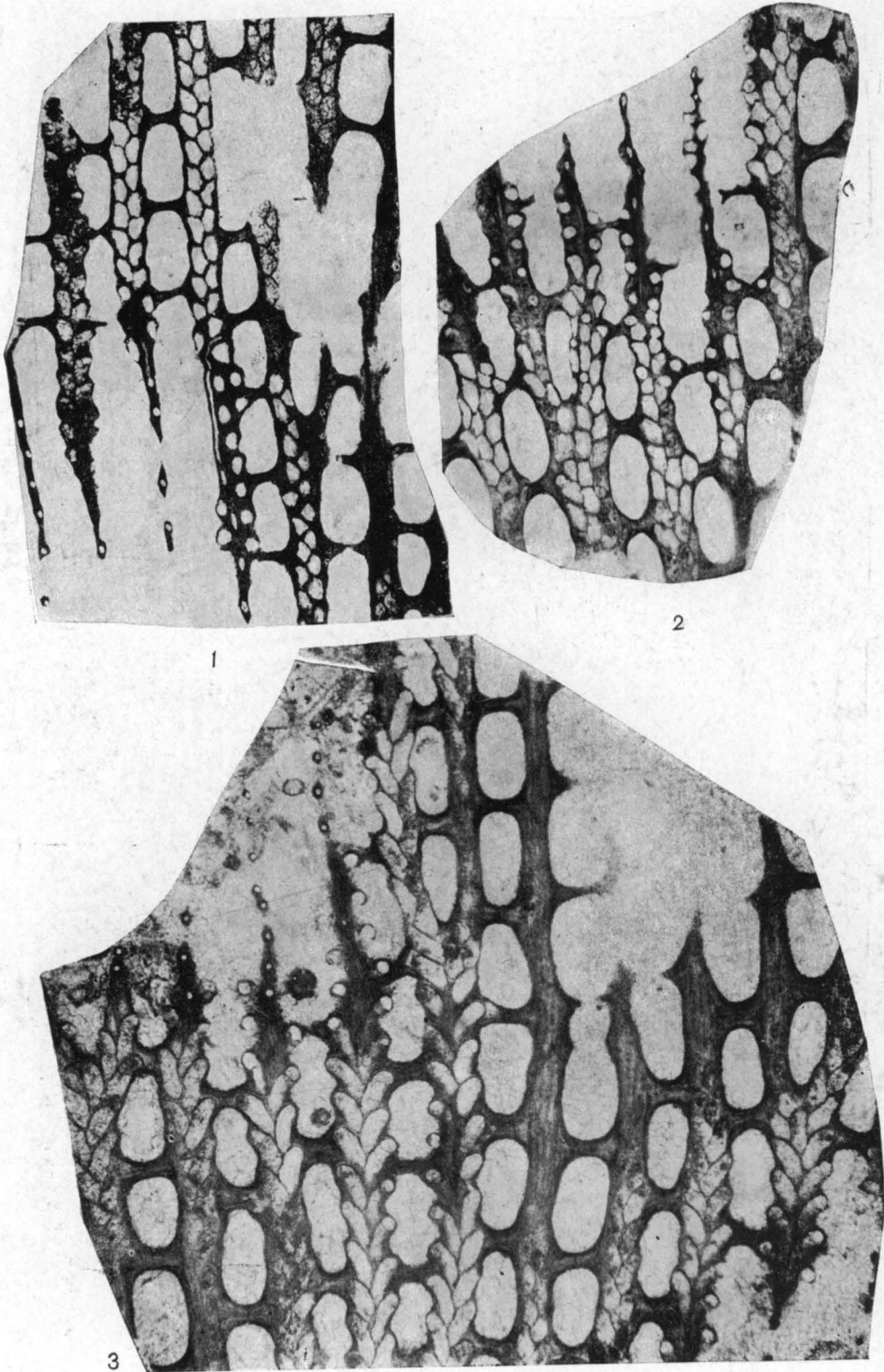
Fenestralia, Fenestella
