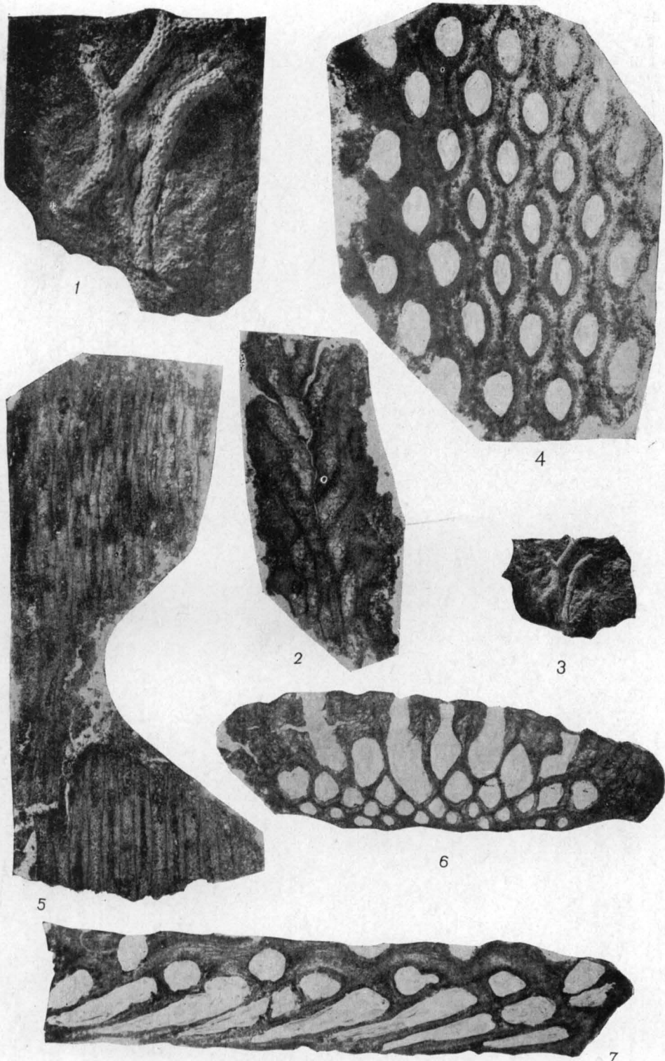
Bashkirella. Rhombocladia
