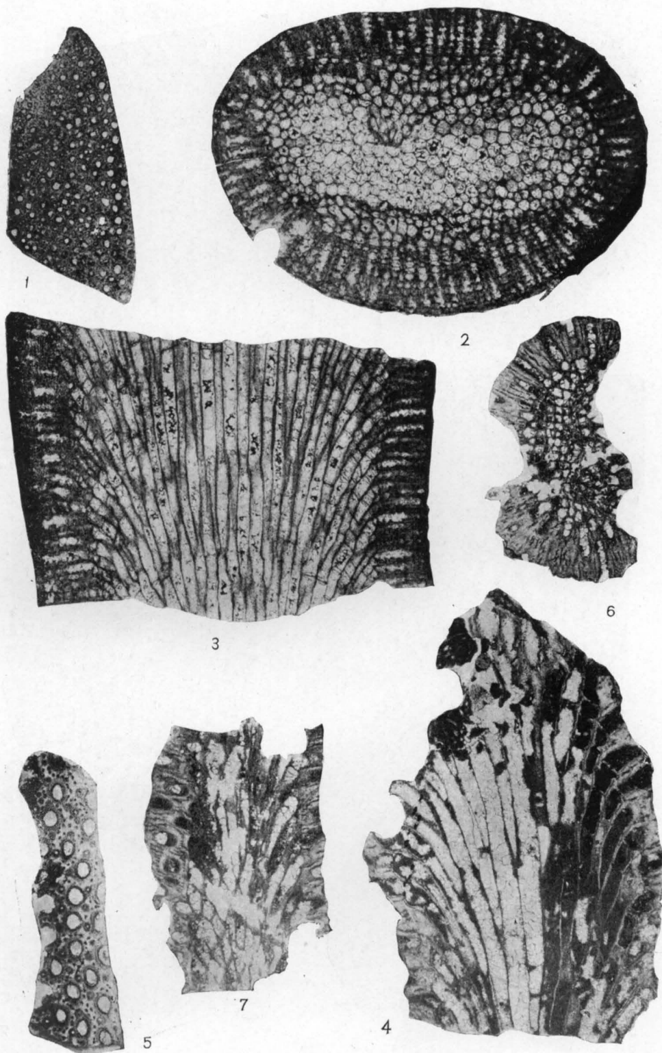
Tabulipora , Rhombotrypella
