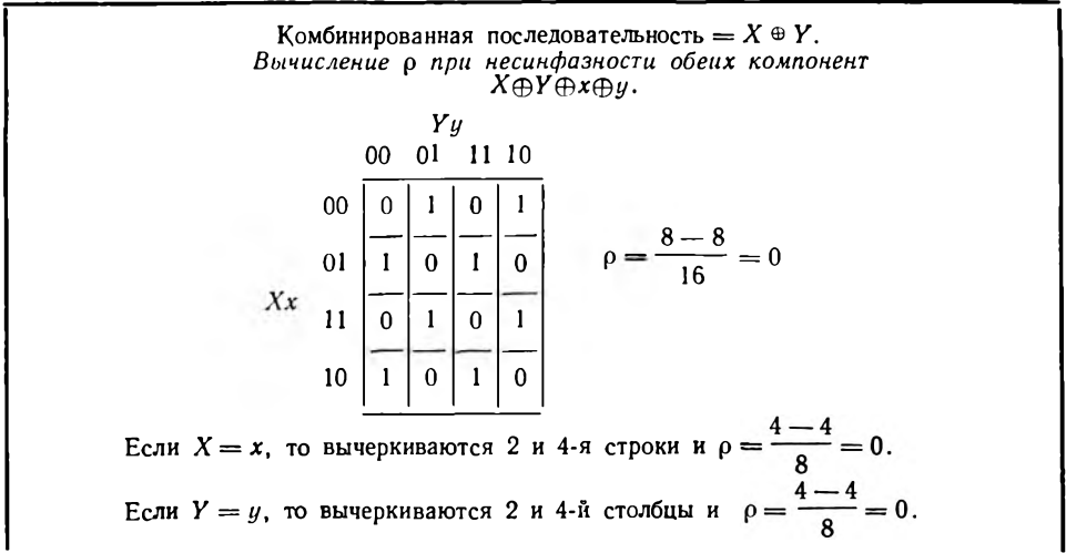
Рис. 5.8. Автокорреляционная функция комбинированной последовательности, не имеющая дополнительных пиков
