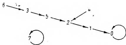
Рис. 2.6. Диаграмма состояний для X_n = X_{n-2}X_{n-3} в десятичном обозначении
