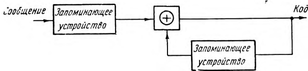
Рис. 7.4. Схема кодера
