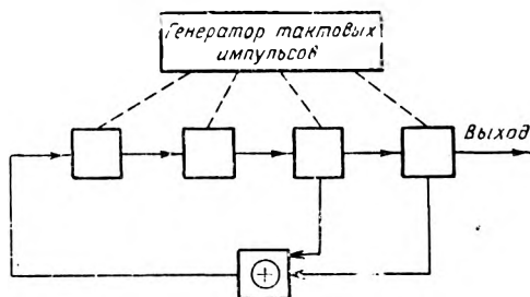
Рис. 2.1. Генератор последовательности с внутренней логикой
