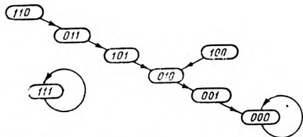
Рис. 2.5. Диаграмма состояний для X_n = X_{n-2}X_{n-3}
