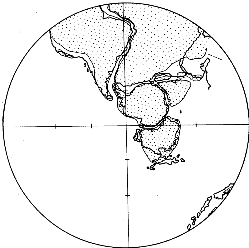
Рис. 46. Схема географического распространения белемнитов в позднеааленское время
