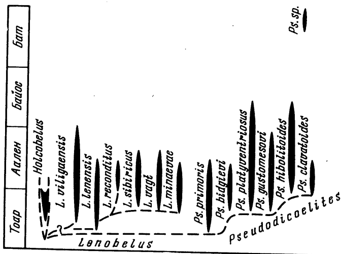
Рис. 43. Схема предполагаемого развития родов и видов подсемейства Pseudodicoelitinae
