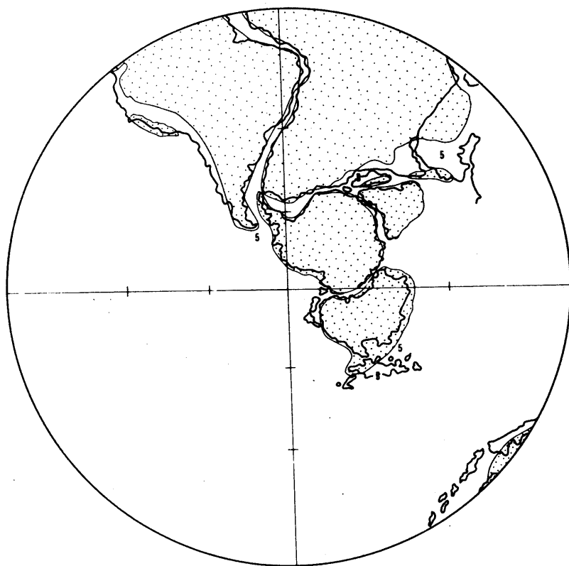
Рис. 48. Схема географического распространения белемнитов в среднебатьское время
