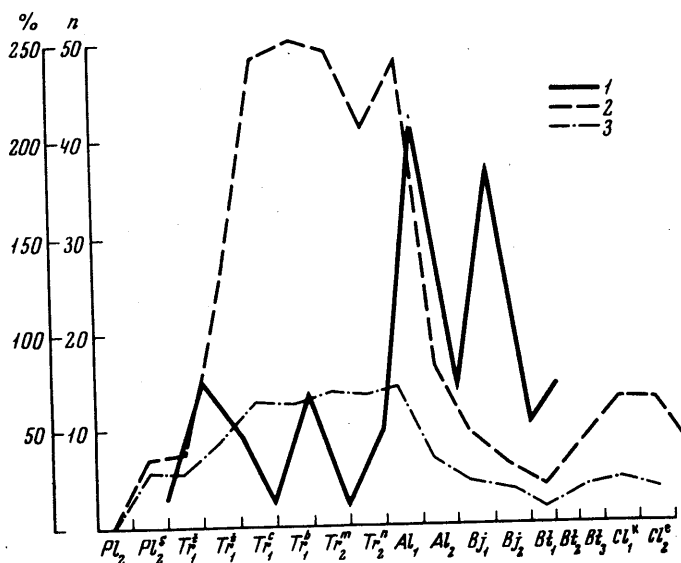
Рис. 45. Колебания коэффициента изменения видового состава белемнитов (1), количества видов (2) и родов (3) в Сибири на протяжении ранне- и среднеюрской эпох
